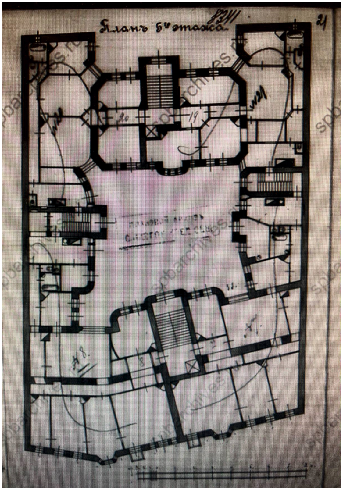
Ил.8 Чертежи дома Г.Г. Гесселя по Невскому пр.95. План 5-го этажа. Гр.инж. Л.М.Харламов. 1912 г. ЦГИА СПб., Ф. 515. Оп. 4. Д.3921. Л. 21.
