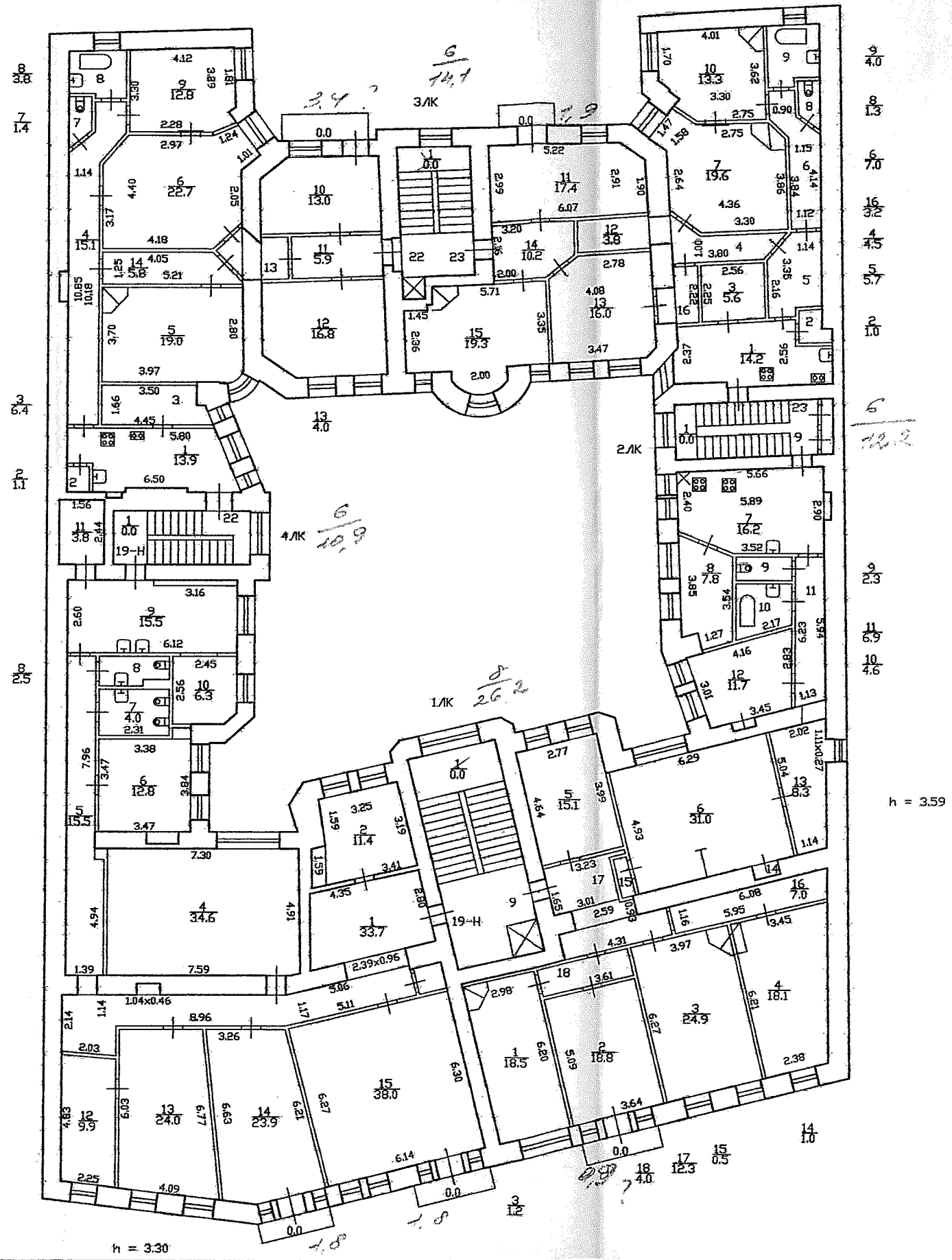
План 6 этажа
