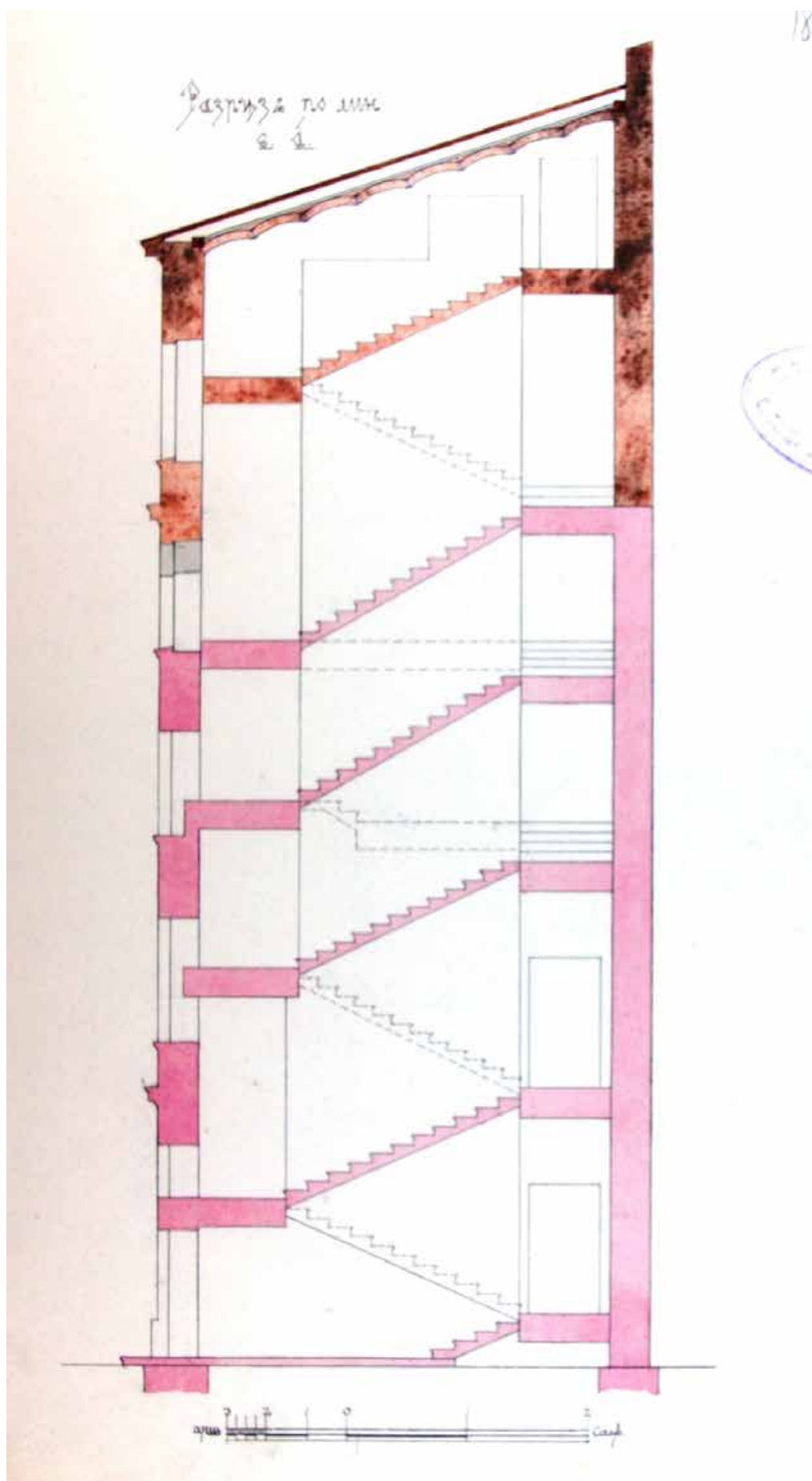
12. Разрез по линии в-в флигеля А дома князя Гагарина. Арх. Н. Л. Бенуа. 1898
