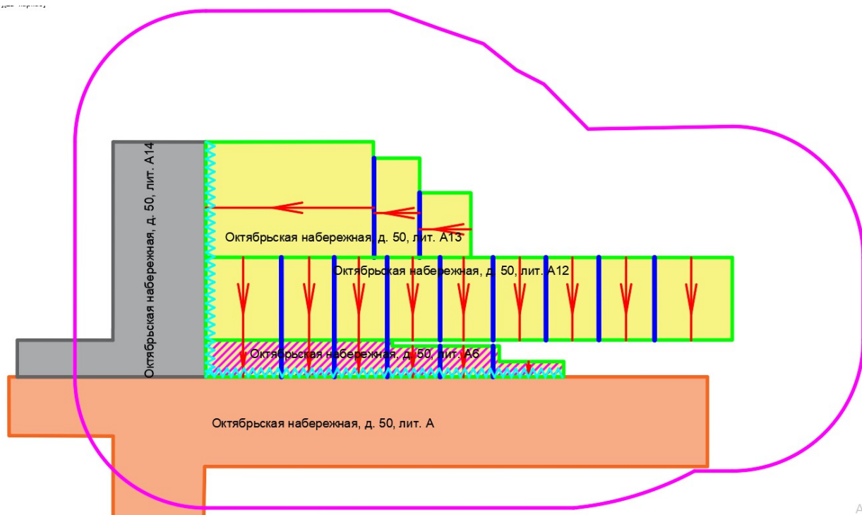
Илл. 3. Схема существующих зданий и сооружений с предварительной зоной влияния и схемой последовательности демонтажа строительных конструкций.
