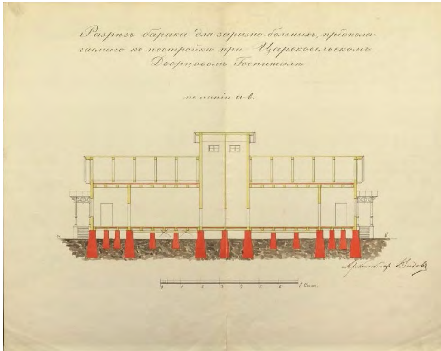
Илл. 8. Царскосельский дворцовый госпиталь. Разрез барака. Арх. Видов Александр Фомич. Период создания: 1887 г. // Источник: Государственный каталог Музейного фонда Российской Федерации. Номер в Госкаталоге: 5616318. Электронный адрес: https://goskatalog.ru/portal/#/collections?id=5769315 .
