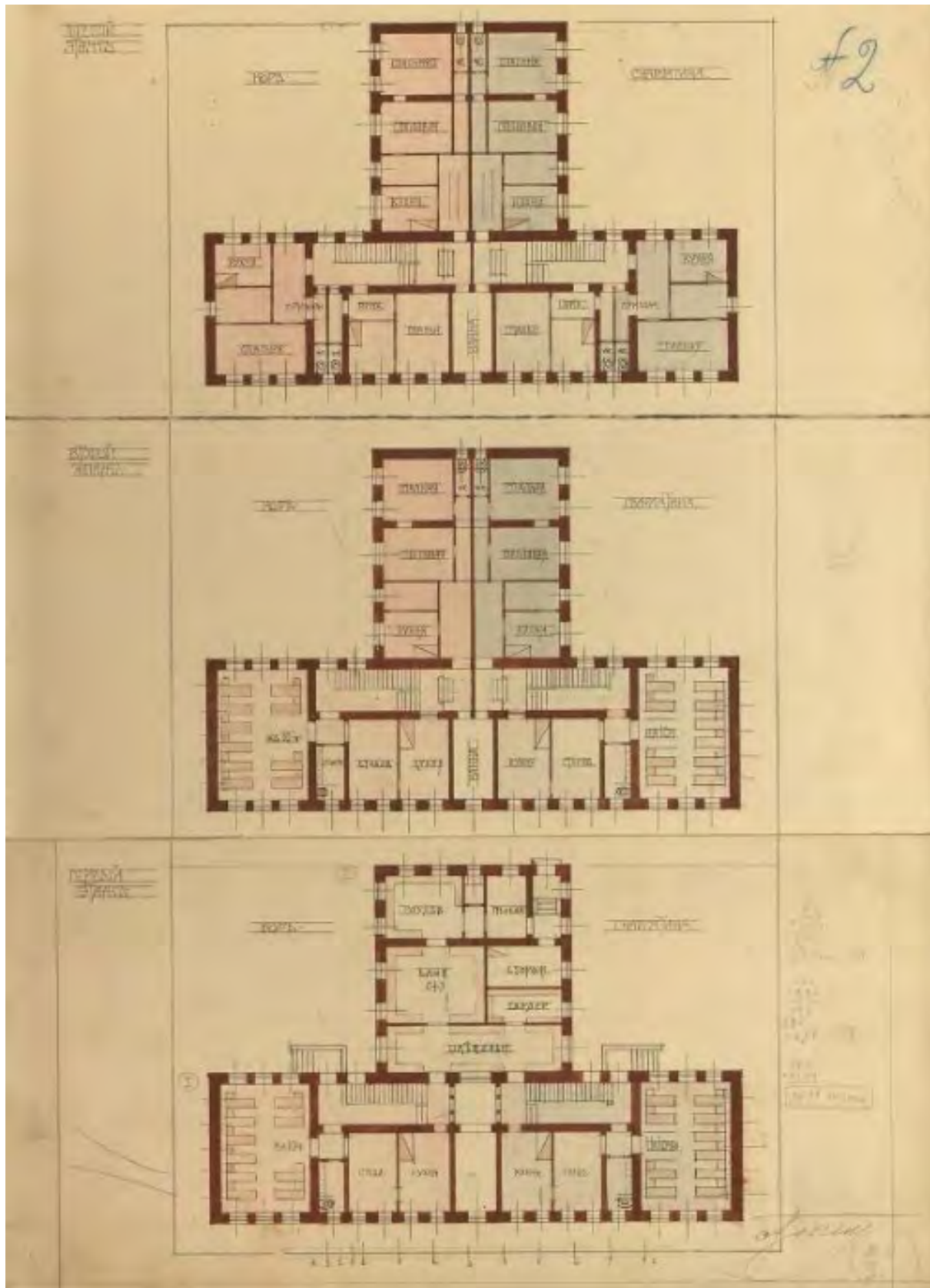
Илл. 12. Царскосельский дворцовый госпиталь. План № 2 павильона для заразных. Неизвестный архитектор. Период создания: конец XIX века. // Источник: Государственный каталог Музейного фонда Российской Федерации. Номер в Госкаталоге: 5616353. Электронный адрес: https://goskatalog.ru/portal/#/collections?id=5769280 .
