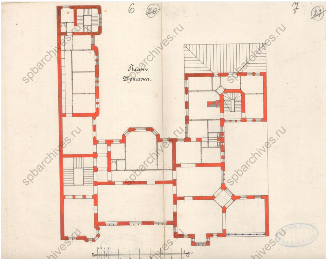
Илл.5 План 2-го этажа. ЦГИА СПб. Ф.513 Оп.102 Д.1544. Чертежи дома на участке, принадлежавшем П.П. Форостовскому по 4-й линии В.О., 9. 1900 г.
