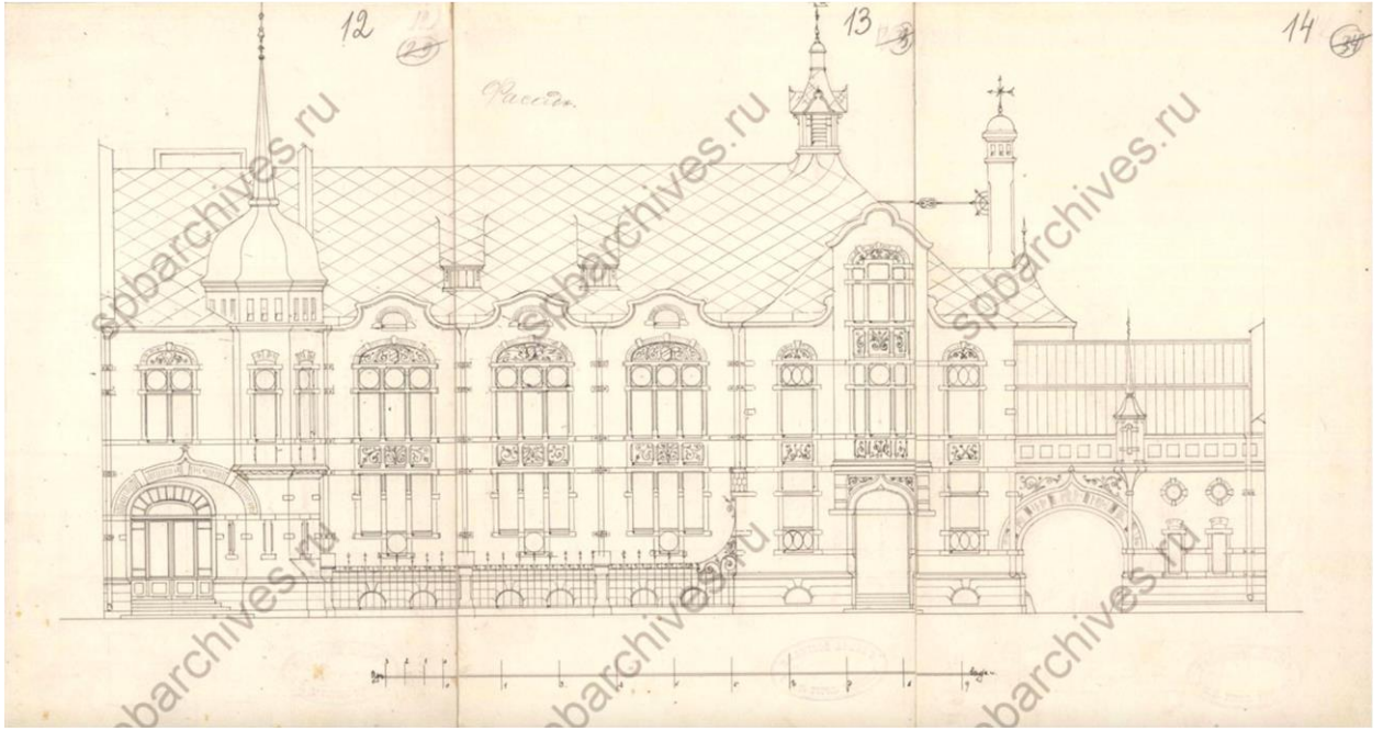
Илл.9 Фасад. ЦГИА СПб. Ф.513 Оп.102 Д.1544. Чертежи дома на участке, принадлежавшем П.П. Форостовскому по 4-й линии В.О., 9. 1900 г.
