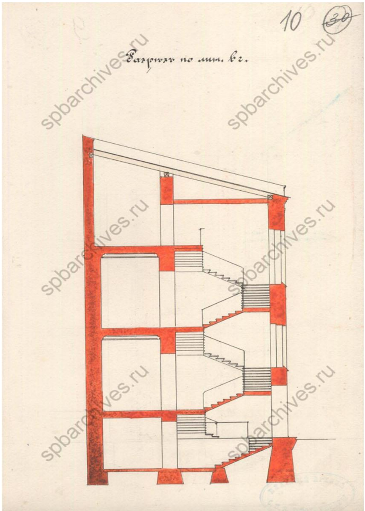
Илл.7 Разрез в-г. ЦГИА СПб. Ф.513 Оп.102 Д.1544. Чертежи дома на участке, принадлежавшем П.П. Форостовскому по 4-й линии В.О., 9. 1900 г.
