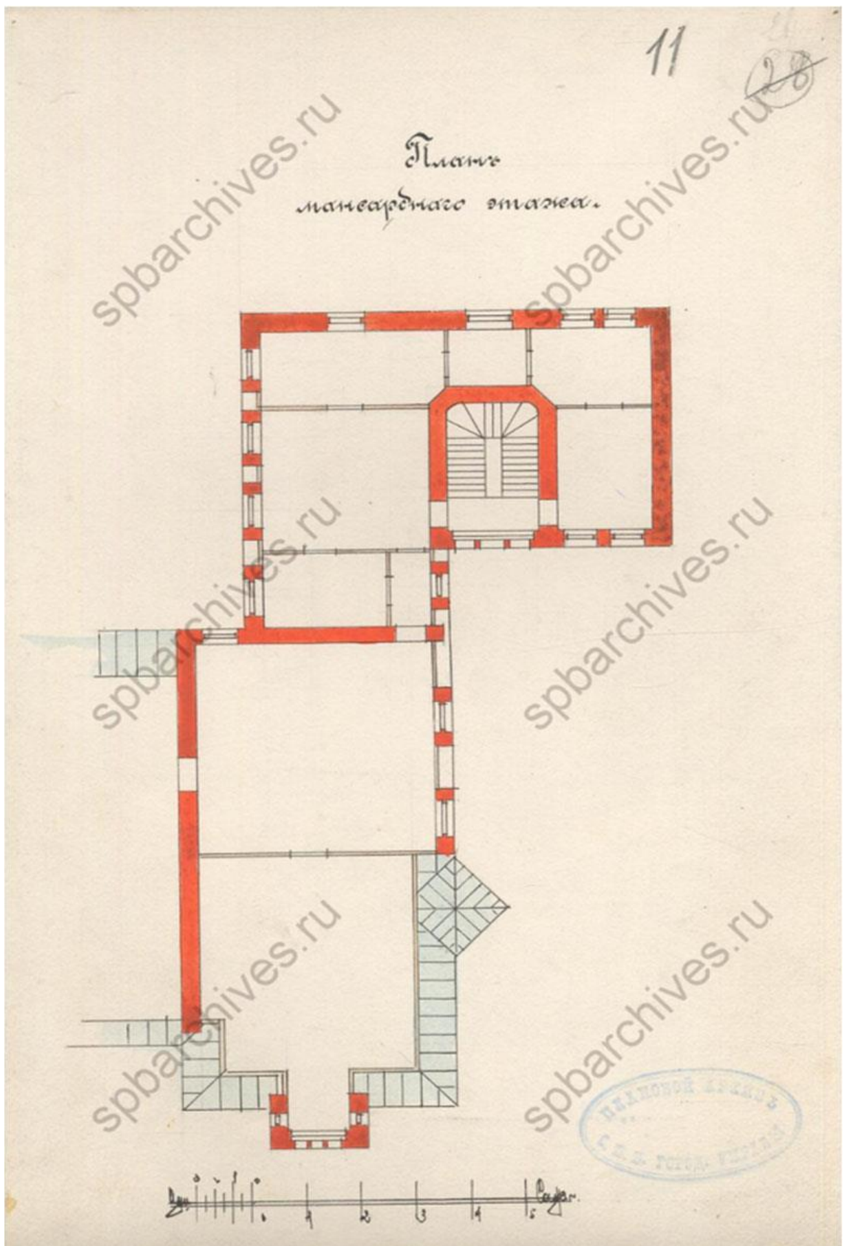
Илл.8 План мансардного этажа. ЦГИА СПб. Ф.513 Оп.102 Д.1544. Чертежи дома на участке, принадлежавшем П.П. Форостовскому по 4-й линии В.О., 9. 1900 г.
