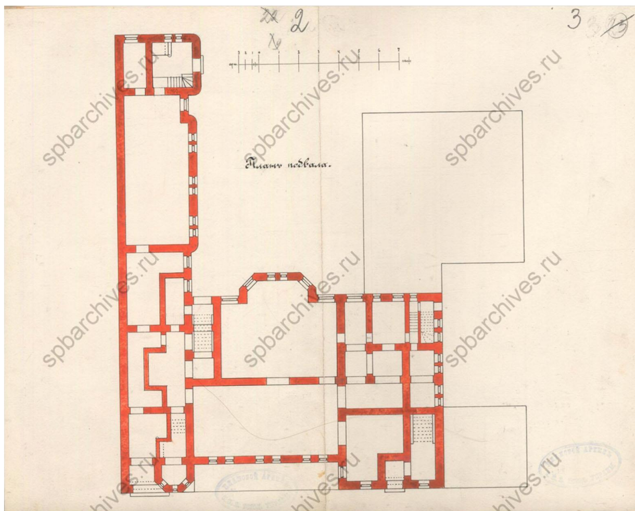
Илл. 3. План подвала. ЦГИА СПб. Ф.513 Оп.102 Д.1544. Чертежи дома на участке, принадлежавшем П.П.Форостовскому по 4-й линии В.О., 9. 1900 г.
