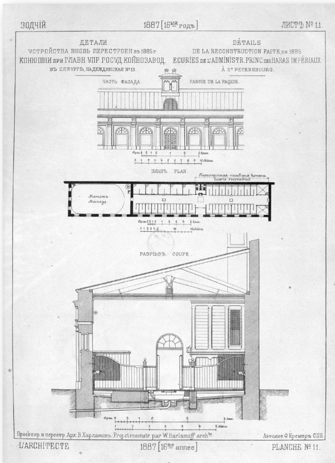
15. Здание аукционной конюшни. План, деталь фасада, разрез. Архитектор В.Ф. Харламов. 1887г. Зодчий. 1887г. Табл. 11.
