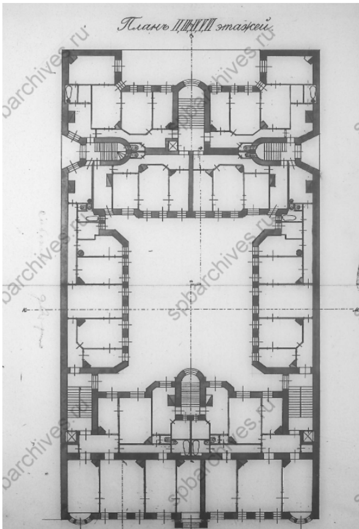
4. План 2-го этажа дома №8 на Конной улице. Арх. Л. Наткин. 1911 // ЦГИА СПб. Фонд 513. Опись 102. Дело 9099. Чертежи дома на участке, принадлежавшем М.В. Плотникову, Н.Г. Павлову, Т.П. Павловой по Конной ул., 8. 1845–1912. Л. 31-32
