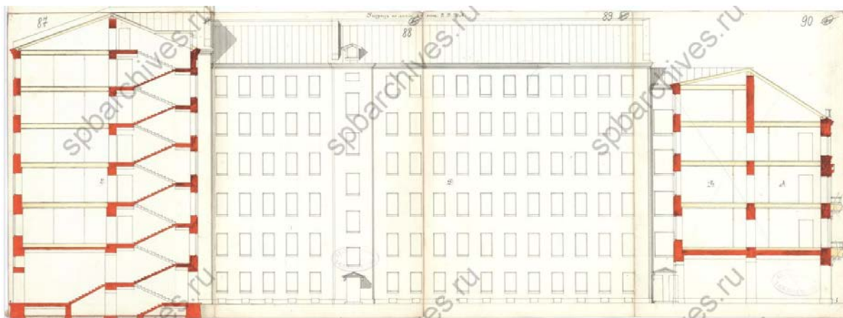
Илл. 29. Разрез по линии е-ј лит.Е, D, В, А. // ЦГИА СПб. Фонд 513. Опись 102. Дело 4249.
