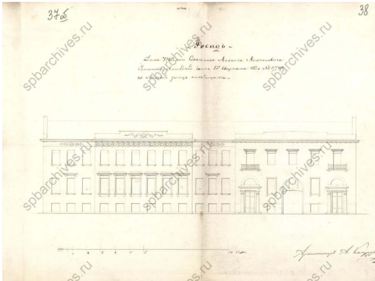
Илл. 15. Фасад Дома Тайного Советника Михаила Михайловича Устинова, Литейной части 1-го квартала под № 57, по Моховой улице. // ЦГИА СПб. Фонд 513. Опись 102. Дело 4249.
