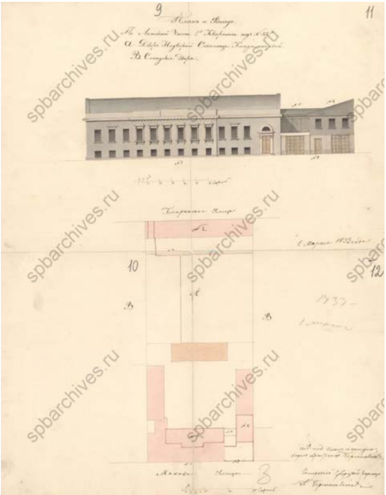
Илл. 7. План и Фасад по Литейной части 1-го Квартала под № 55. 1 марта 1833 года. // ЦГИА СПб. Фонд 513. Опись 102. Дело 4249.
