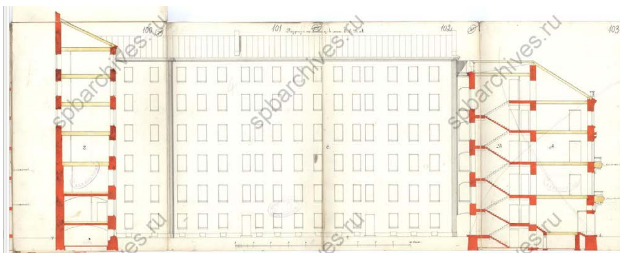
Илл. 32. Разрез по линии g-h лит. Е, С, В, А. // ЦГИА СПб. Фонд 513. Опись 102. Дело 4249.
