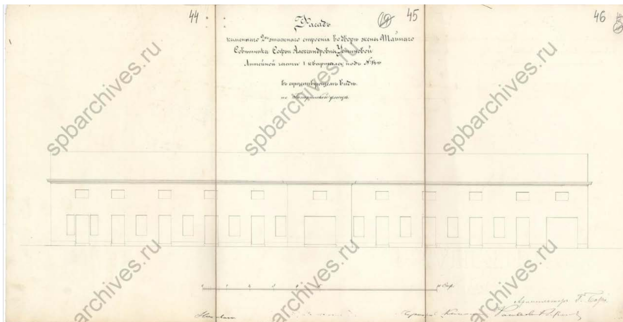
Илл. 18. Фасад каменного 2-х этажного строения во дворе жены Тайного Советника Софьи Александровны Устиновой Литейной части 1 квартала под № 14 в существующем виде по Гагаринской улице. // ЦГИА СПб. Фонд 513. Опись 102. Дело 4249.
