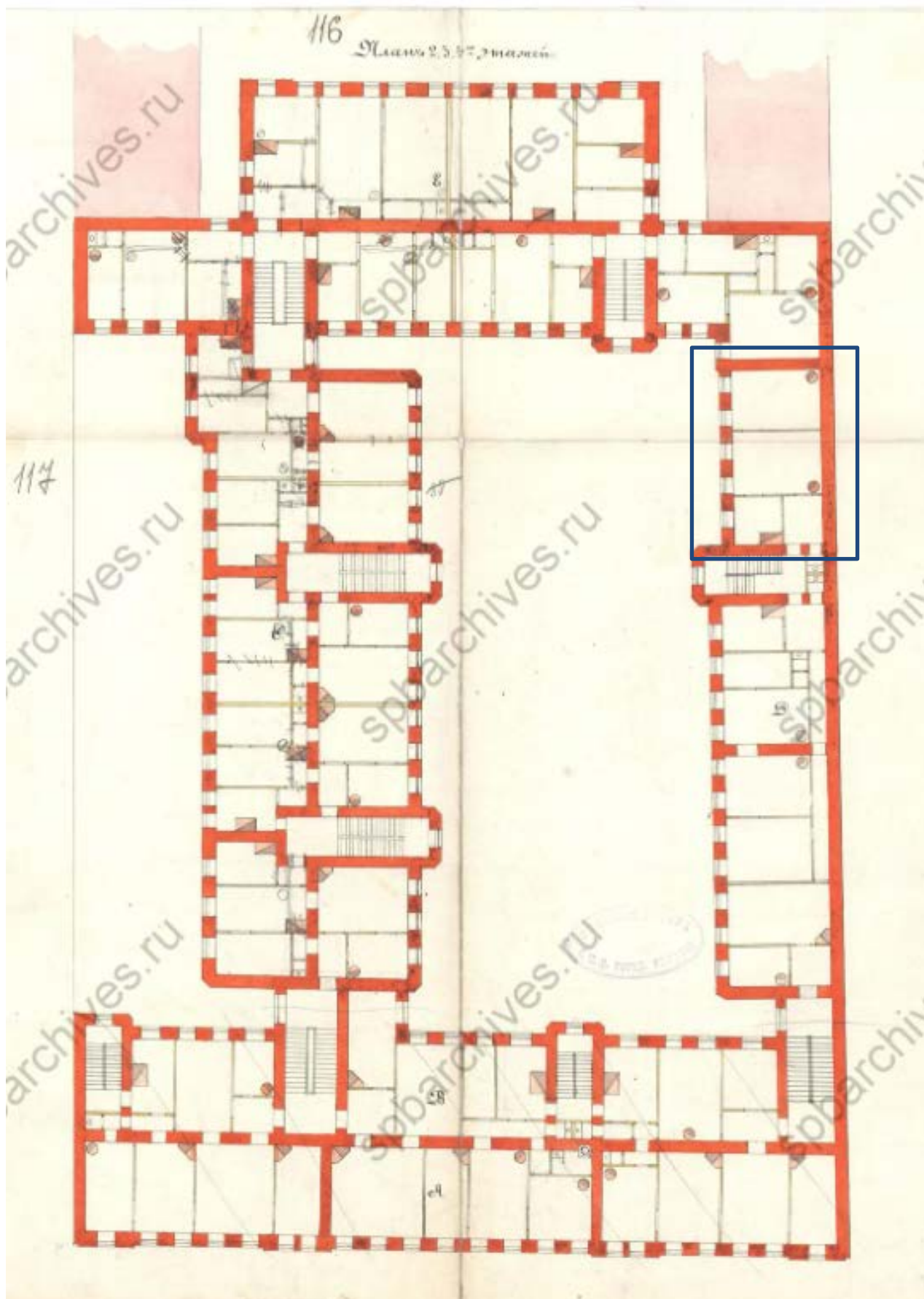
Илл. 36. План 2-го, 3-го, 4-го этажей. // ЦГИА СПб. Фонд 513. Опись 102. Дело 4249.
