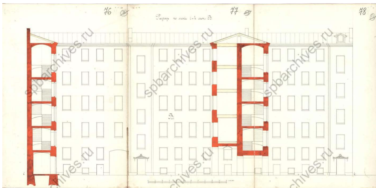
Илл. 26. Разрез по линии i-k лит. В. // ЦГИА СПб. Фонд 513. Опись 102. Дело 4249.
