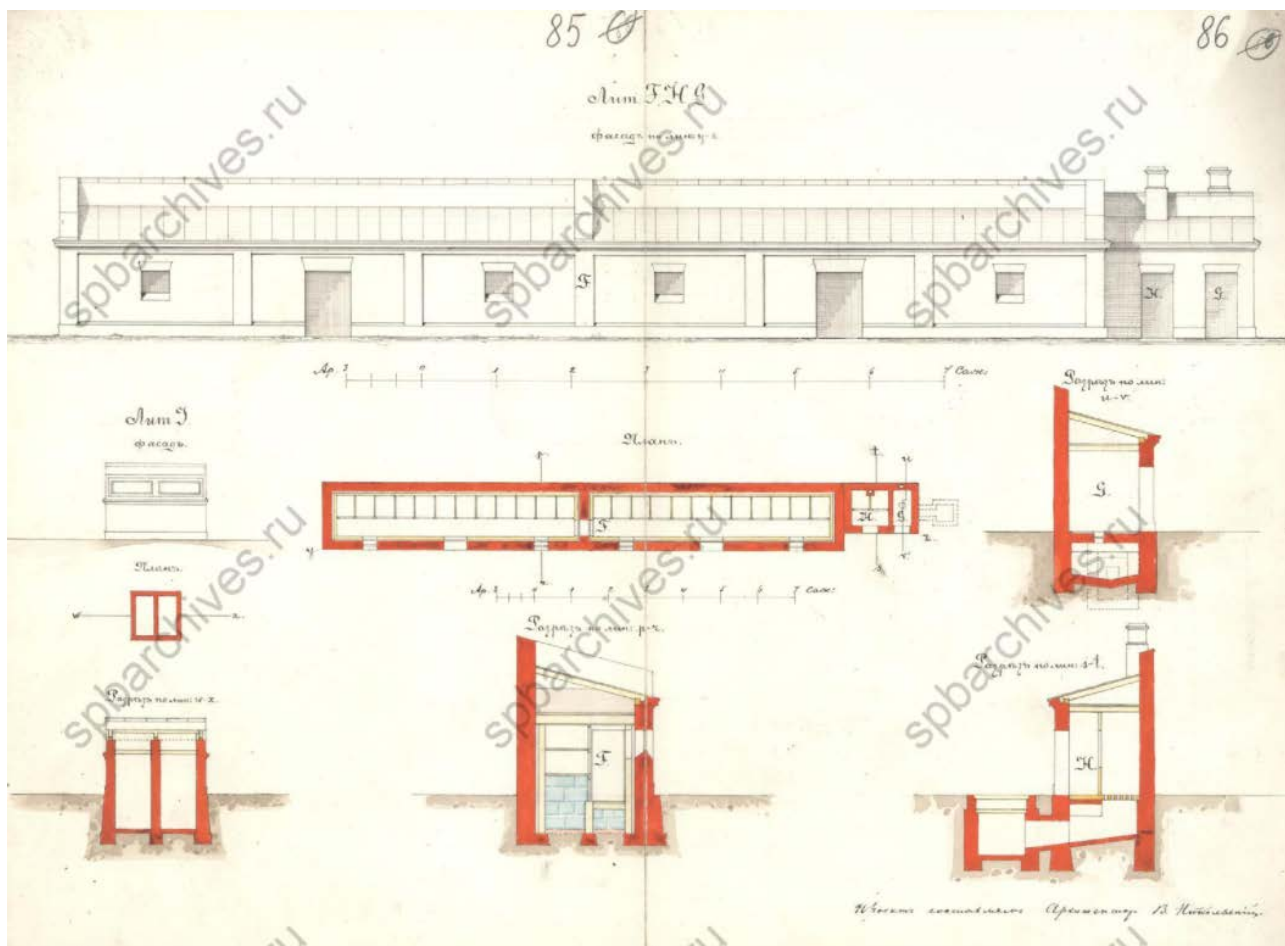
Илл. 28. Фасады, планы и разрезы лит. F, H, G // ЦГИА СПб. Фонд 513. Описание 102. Дело 4249.
