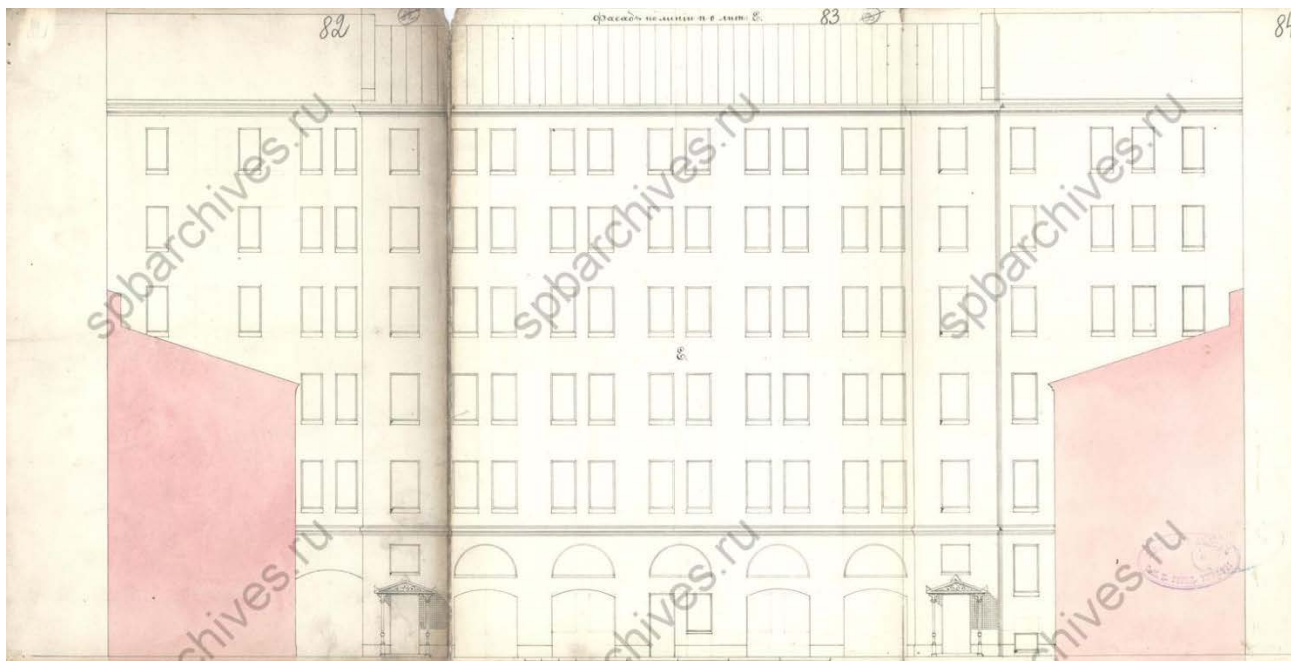
Илл. 27. Разрез по линии п-о лит. Е. // ЦГИА СПб. Фонд 513. Описание 102. Дело 4249.
