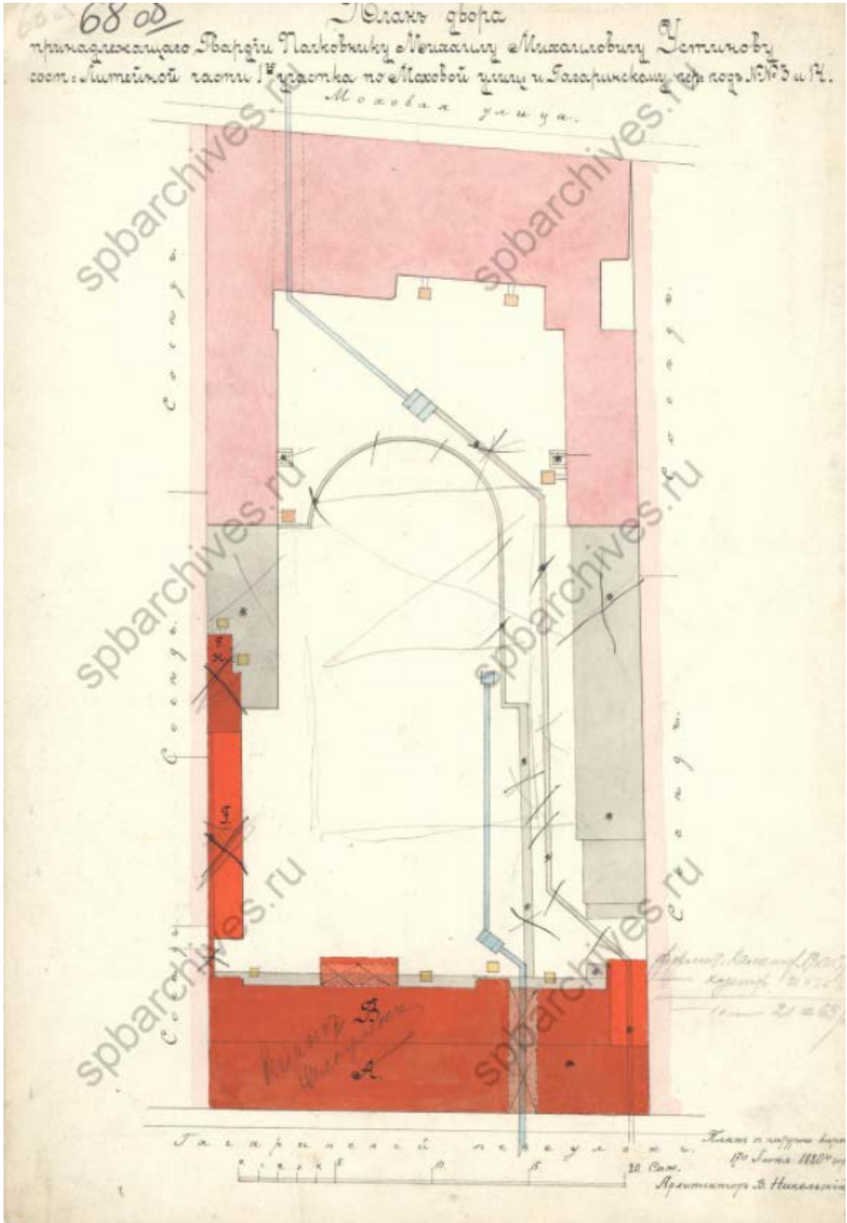
Илл. 22. План двора, принадлежащего Гвардии Полковнику Михаилу Михайловичу Устинову сост. Литейной части 1-го участка по Моховой улице и Гагаринскому пер. под №№ 3 и 14. 17 июня 1880 г. Архитектор В. Никольский. // ЦГИА СПб. Фонд 513. Описание 102. Дело 4249.
