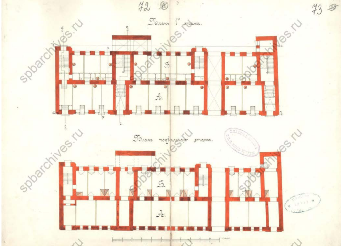
Илл. 24. План подвального этажа. План 1-го этажа. // ЦГИА СПб. Фонд 513. Опись 102. Дело 4249.
