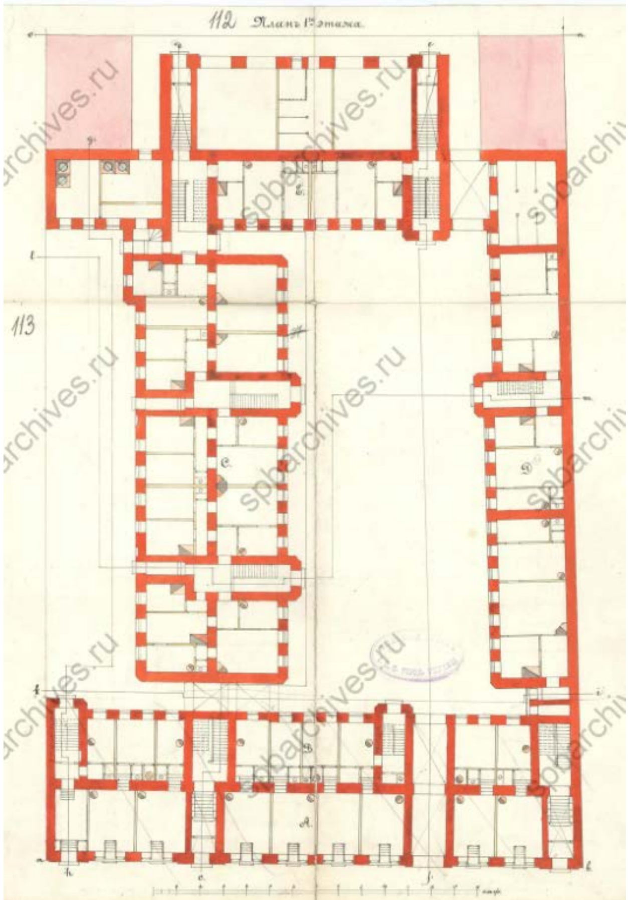
Илл. 35. План 1-го этажа. // ЦГИА СПб. Фонд 513. Опись 102. Дело 4249.
