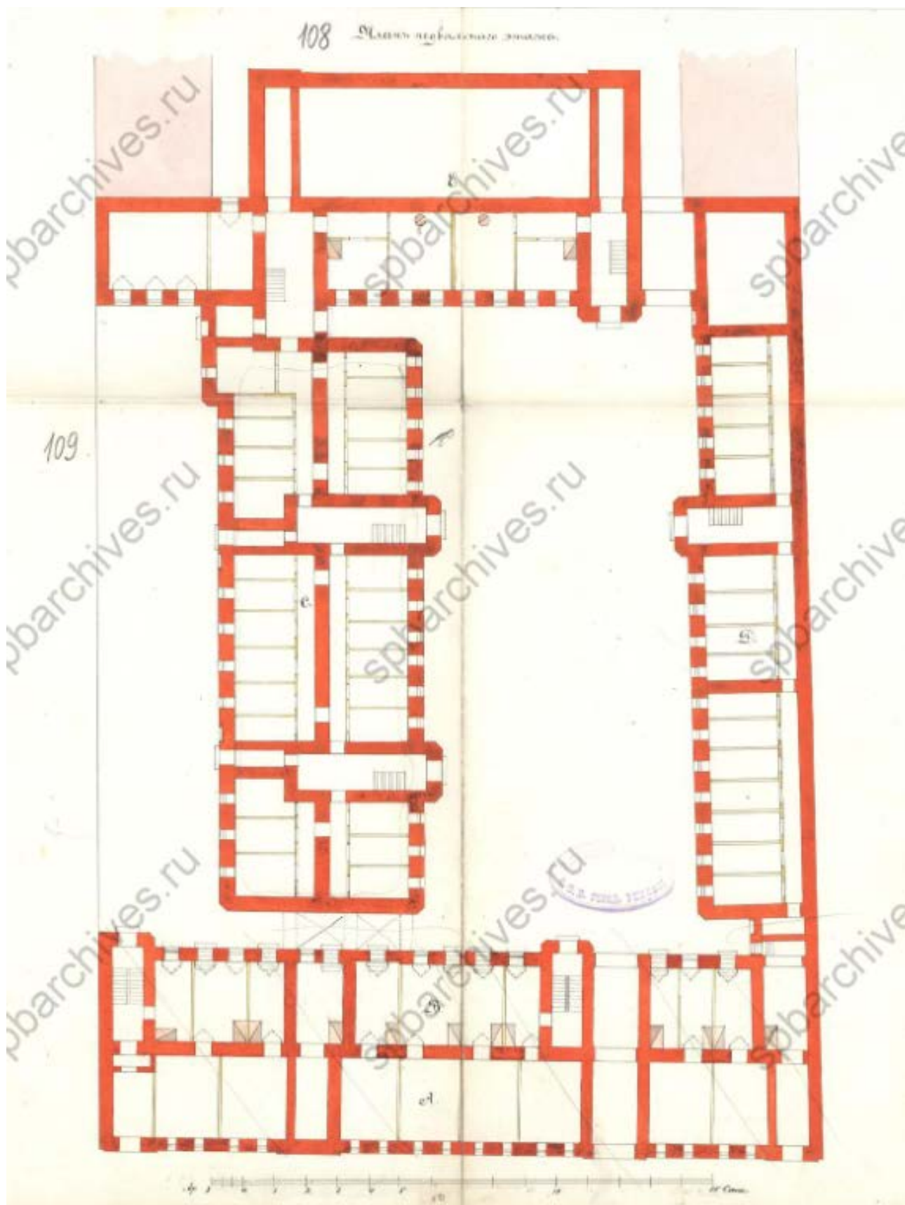
Илл. 34. План подвального этажа. // ЦГИА СПб. Фонд 513. Опись 102. Дело 4249.
