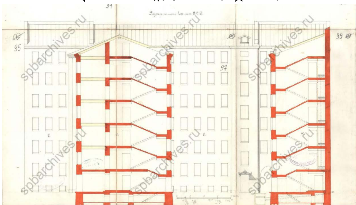
Илл. 31. Разрез по линии l-m лит Е, С, D. // ЦГИА СПб. Фонд 513. Опись 102. Дело 4249.
