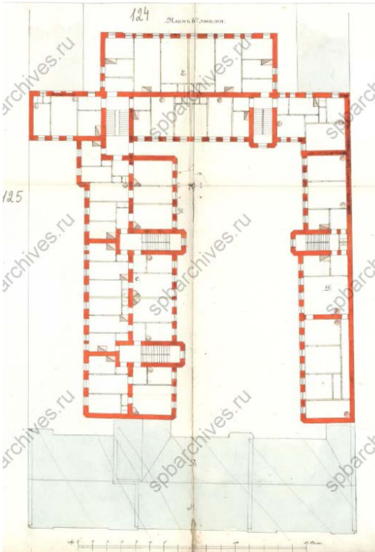
Илл. 38. План 6-го этажа. // ЦГИА СПб. Фонд 513. Опись 102. Дело 4249.
