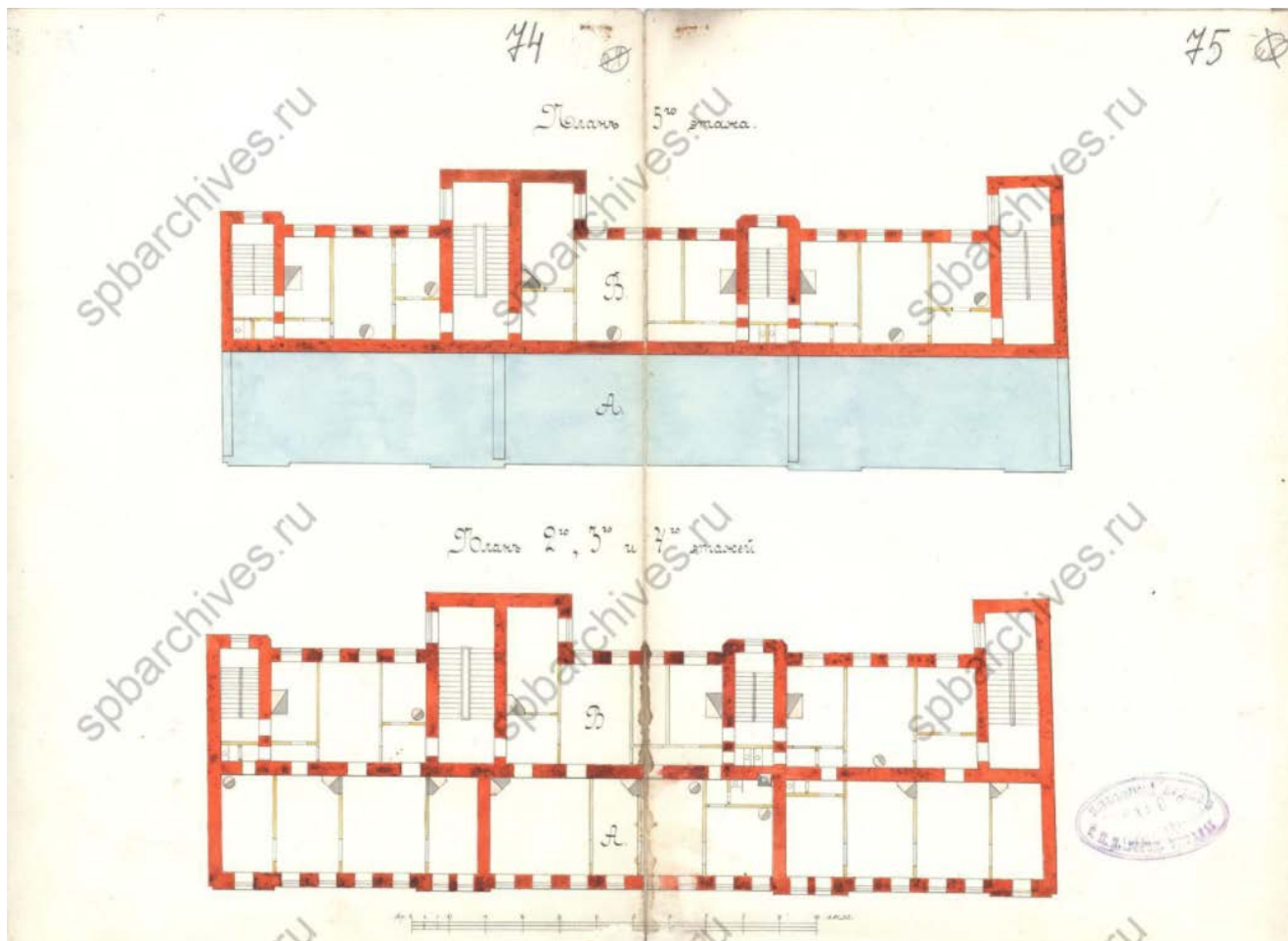
Илл. 25. План 2-го, 3-го, 4-го этажей. План 5-го этажа. // ЦГИА СПб. Фонд 513. Опись 102. Дело 4249.
