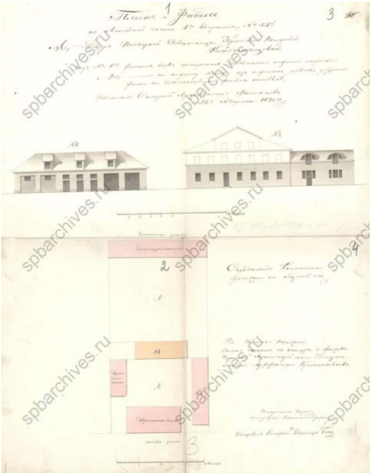
Илл. 5. План и фасады по Литейной части 1-го квартала № 55. А Двор Надворной Советницы Прасковьи Петровой Кандалицевой. 1830 г. // ЦГИА СПб. Фонд 513. Опись 102. Дело 4249.
