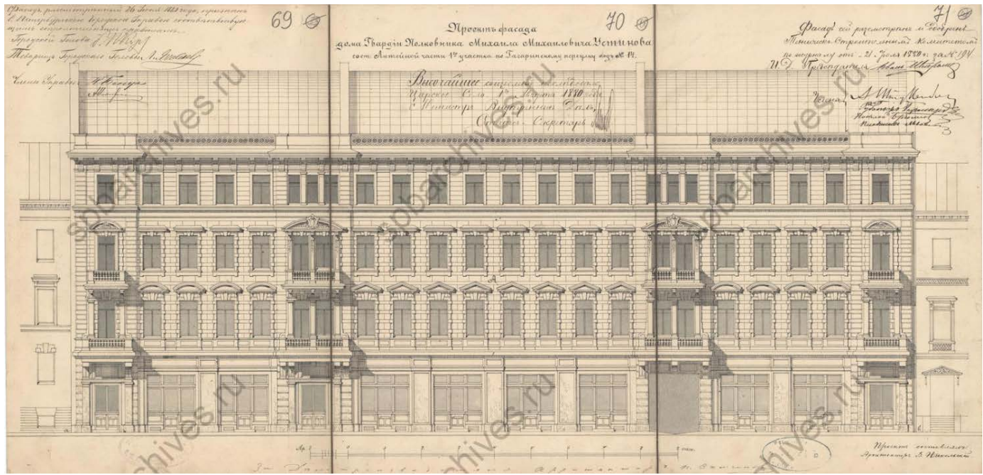
Илл. 23. Проект фасада дома Гвардии Полковнику Михаилу Михайловичу Устинову сост. Литейной части 1-го участка по Гагаринскому переулку под № 14.26 июня 1880 г. Архитектор В. Никольский. // ЦГИА СПб. Фонд 513. Опись 102. Дело 4249.
