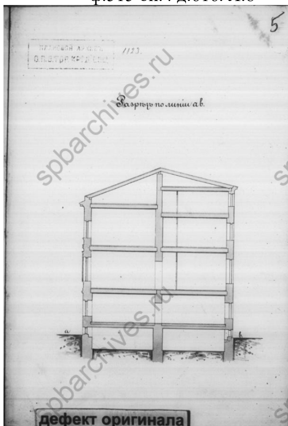
11. Разрез по линии ав. 1898 г. Чертежи дома С.Г.Степанова, Н.В.Дмитриева по Гагаринской ул.,16. ЦГИА СПб ф.515 оп.4 д.616. Л.9
