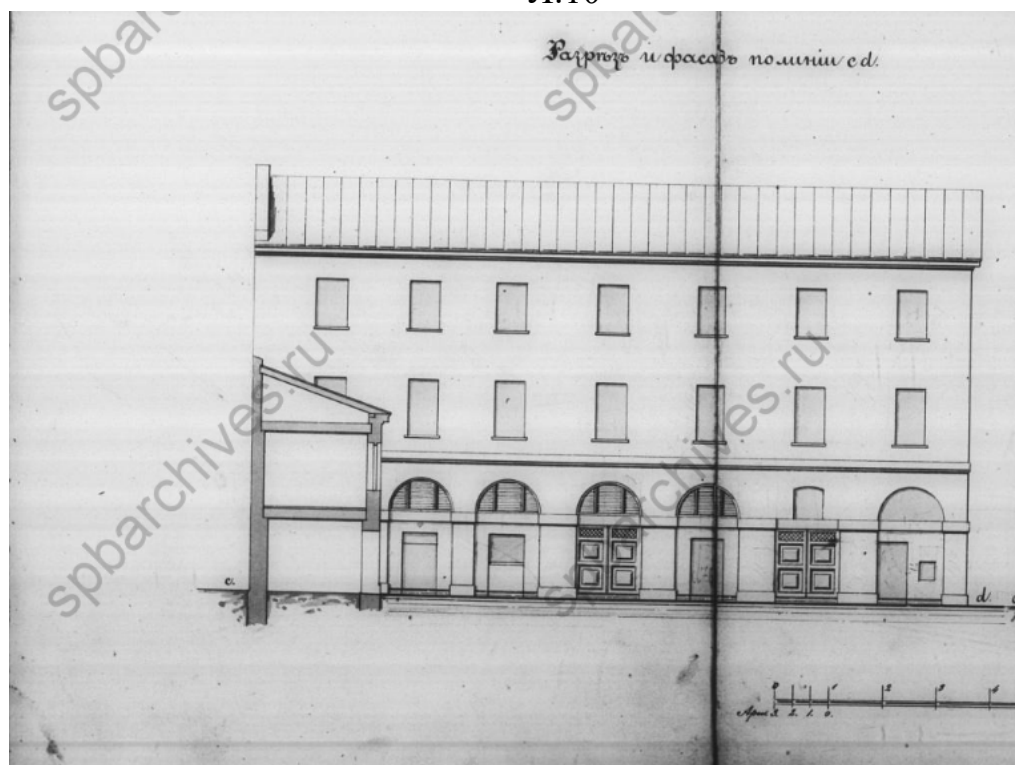
13. Разрез и фасад по линии cd. 1898 г. Чертежи дома С.Г. Степанова, Н.В. Дмитриева по Гагаринской ул., 16. ЦГИА СПб ф.515 оп.4 д.616. Л.11
