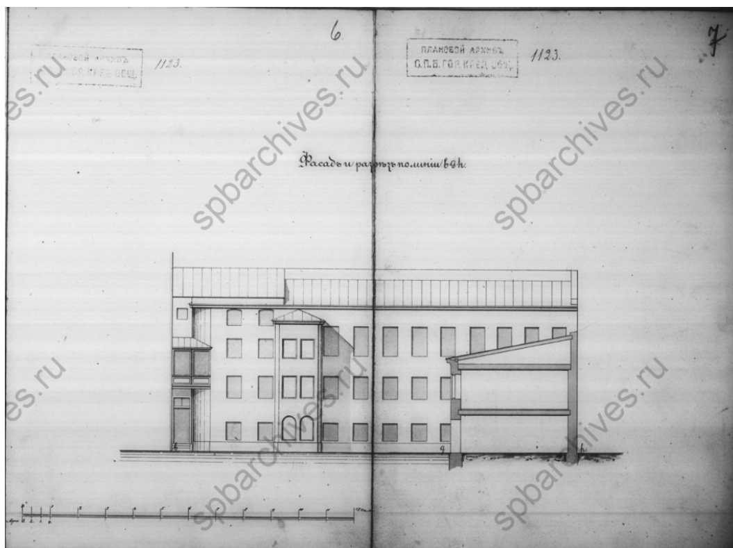
12. Фасад и разрез по линии bgh. 1898 г. Чертежи дома С.Г. Степанова, Н.В. Дмитриева по Гагаринской ул., 16. ЦГИА СПб ф.515 оп.4 д.616. Л.10
