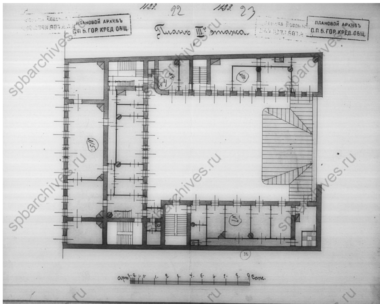
23. План 3-го этажа. 1909 г. Чертежи дома С.Г.Степанова, Н.В.Дмитриева по Гагаринской ул.,16. ЦГИА СПб ф.515 оп.4 д.616. Л.22
