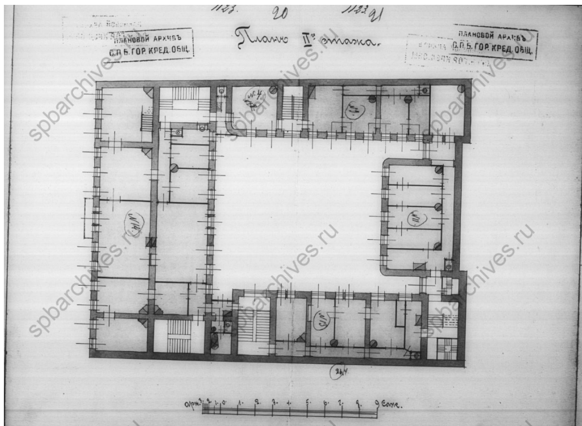
22. План 2-го этажа. 1909 г. Чертежи дома С.Г. Степанова, Н.В. Дмитриева по Гагаринской ул., 16. ЦГИА СПб ф.515 оп.4 д.616. Л.21
