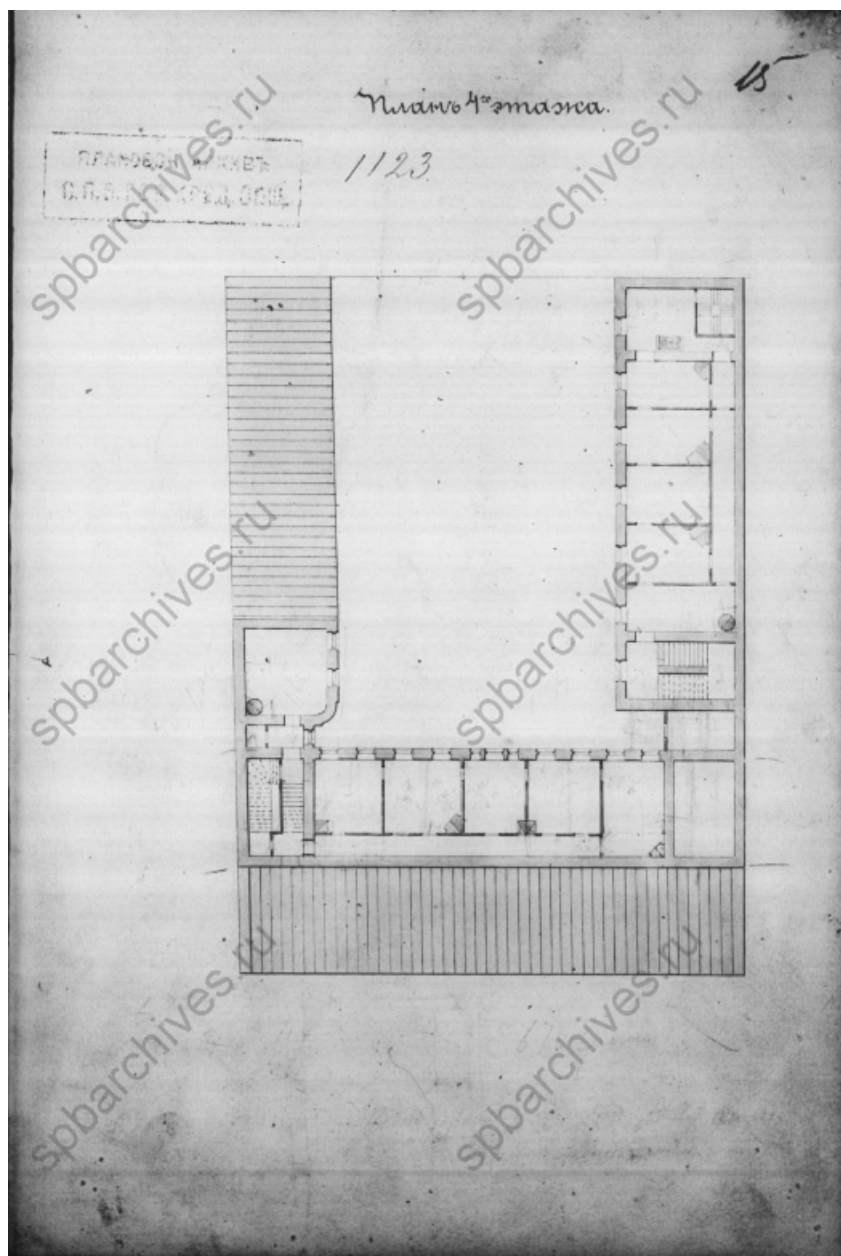
19. План 4-го этажа. 1898 г. Чертежи дома С.Г. Степанова, Н.В. Дмитриева по Гагаринской ул., 16. ЦГИА СПб ф.515 оп.4 д.616. Л.17
