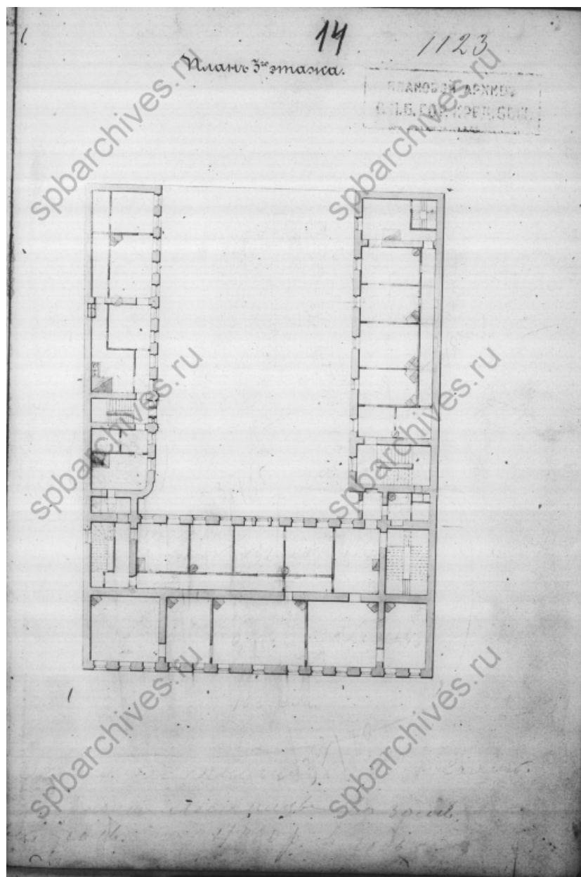
18. План 3-го этажа. 1898 г. Чертежи дома С.Г.Степанова, Н.В.Дмитриева по Гагаринской ул.,16. ЦГИА СПб ф.515 оп.4 д.616. Л.16
