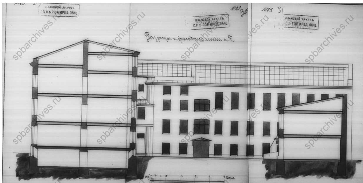
26. Разрез по линии аб. План 4-го этажа. 1909 г. Чертежи дома С.Г. Степанова, Н.В. Дмитриева по Гагаринской ул., 16. ЦГИА СПб ф.515 оп.4 д.616. Л.27-28
