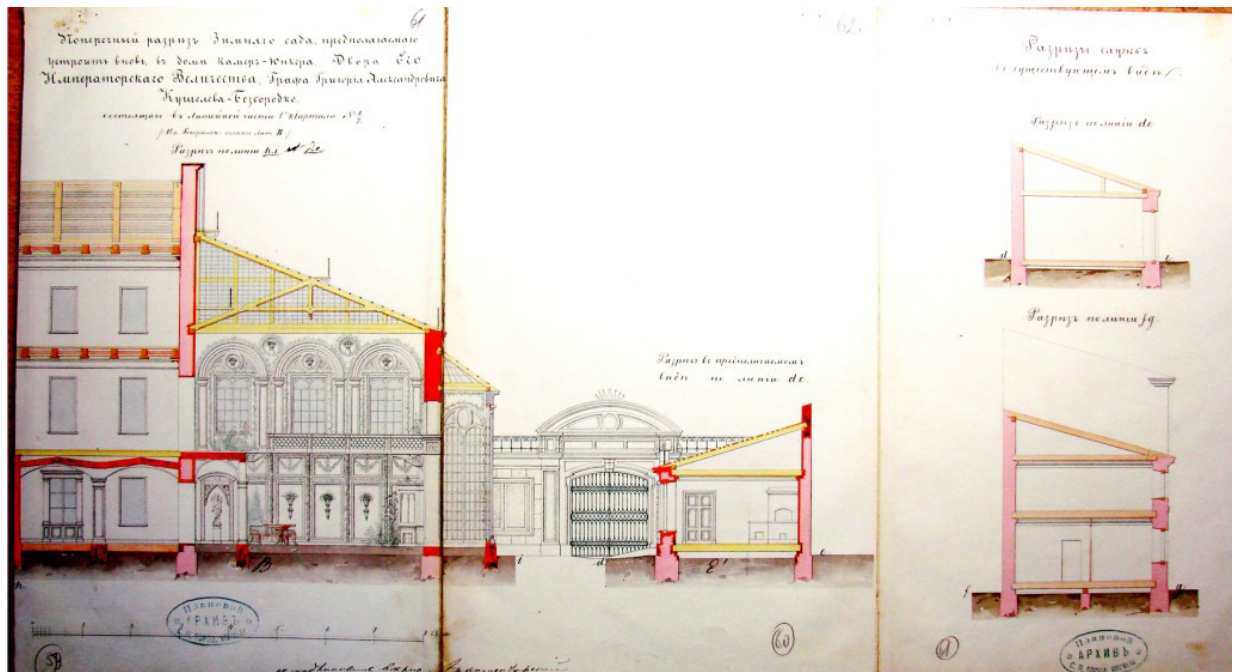
Илл. 13. Разрез дворовых флигелей дома графа А.Г.Кушелева-Безбородко с показанием вновь предполагаемого зимнего сада. Арх. Р.Р.Генрихсен. 1857 г. ЦГИА СПб. Ф. 513. Оп. 102. Д. 3989. Л. 61-63.
