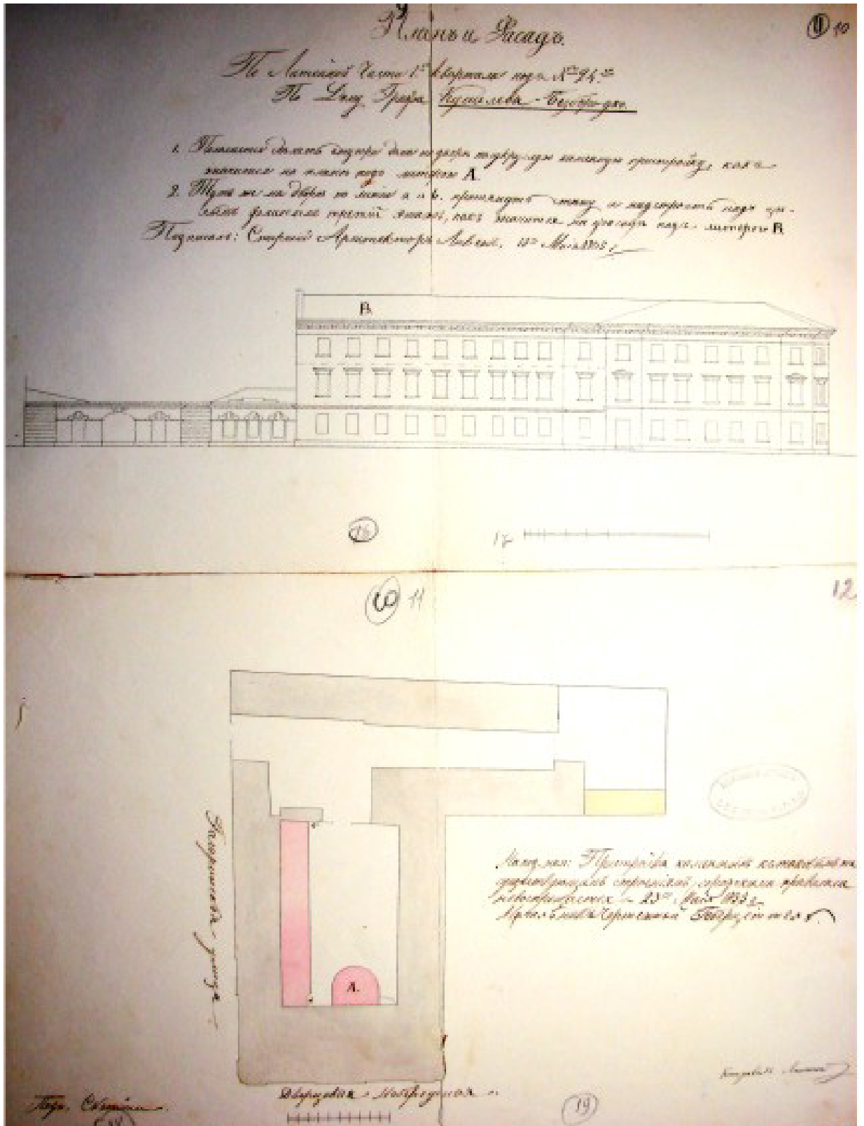
Илл. 6. План двора и фасад дома графа А.Г.Кушелева-Безбородко. Арх. И.П.Скотти. 1835 г. ЦГИА СПб. Ф. 513. Оп. 102. Д. 3989. Л. 9-12.
