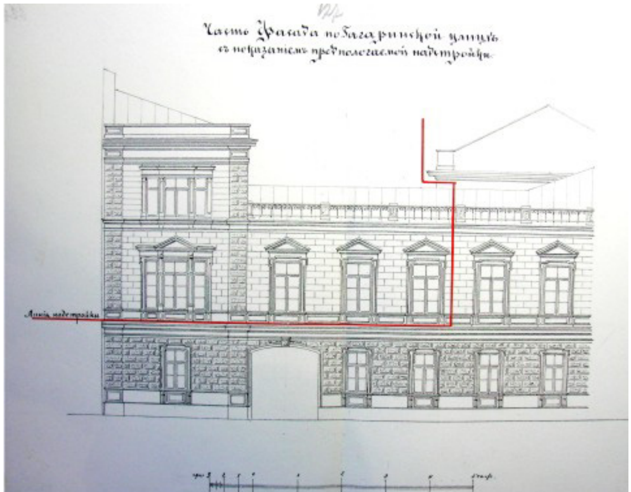
Илл. 17. Проект надстройки 2-го этажа на месте проездных ворот дома купца А.Г.Елисеева. Фасад. Арх. А.К.Гаммерштедт. 1893 г. ЦГИА СПб. Ф. 513. Оп. 102. Д. 3989. Л. 132-133.
