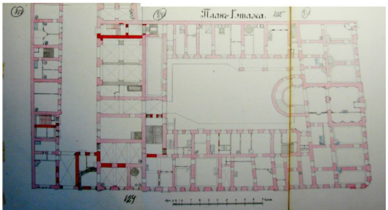
Илл. 18. Проект надстройки 2-го этажа на месте проездных ворот дома купца А.Г.Елисеева. Фрагмент плана 1-го этажа. Арх. А.К.Гаммерштедт. 1893 г. ЦГИА СПб. Ф. 513. Оп. 102. Д. 3989. Л. 123-126.
