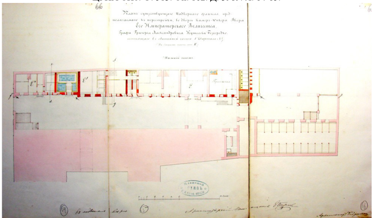
Илл. 12. План нижнего этажа перестраиваемого южного дворового флигеля дома графа А.Г.Кушелева-Безбородко с показанием вновь предполагаемых оранжерей. Арх. Р.Р.Генрихсен. 1857 г. ЦГИА СПб. Ф. 513. Оп. 102. Д. 3989. Л. 66-68.
