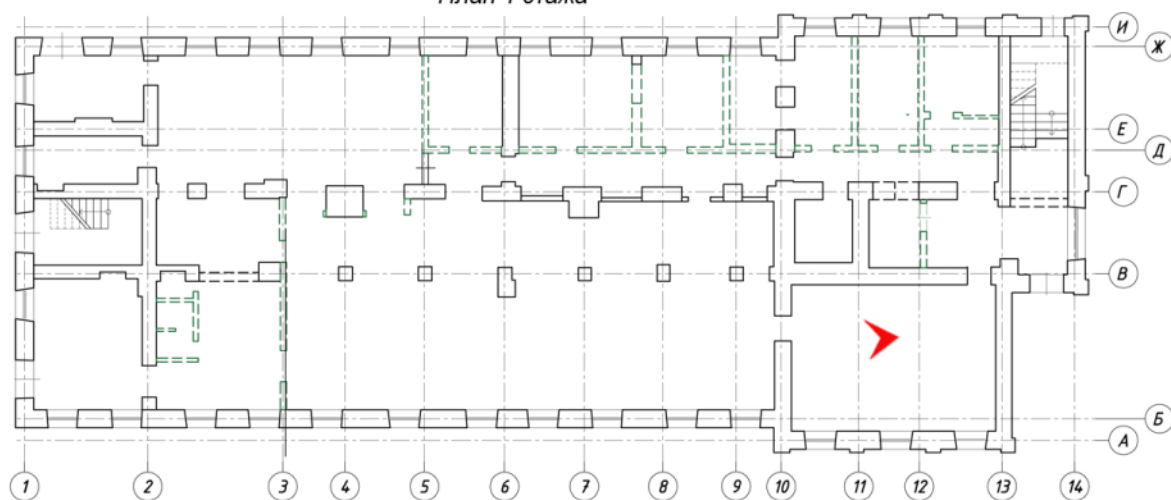
План 1 этажа
