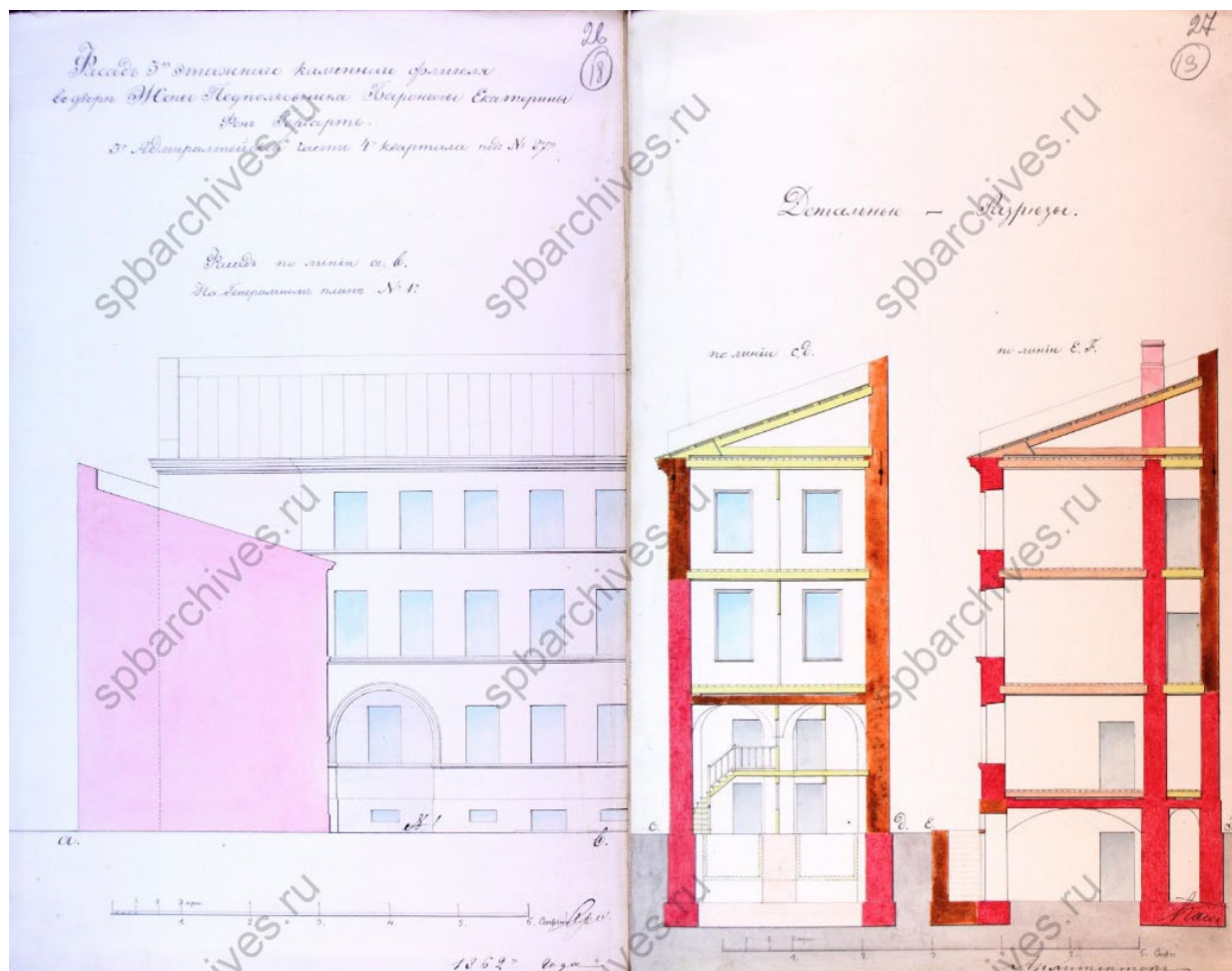
16. Фасад по линии а.в., детальные разрезы. Чертежи дома на участке, принадлежавшем Д.Колотушкину, А.Колотушкину, Е.Герварт, Н.Ф.Заремба, П.Н.Глаголеву по наб.р.Фонтанки, 103. ЦГИА СПб. Фонд 513. Опись 102. Дело 9949. 1826–1912 гг. л. 26-27;
