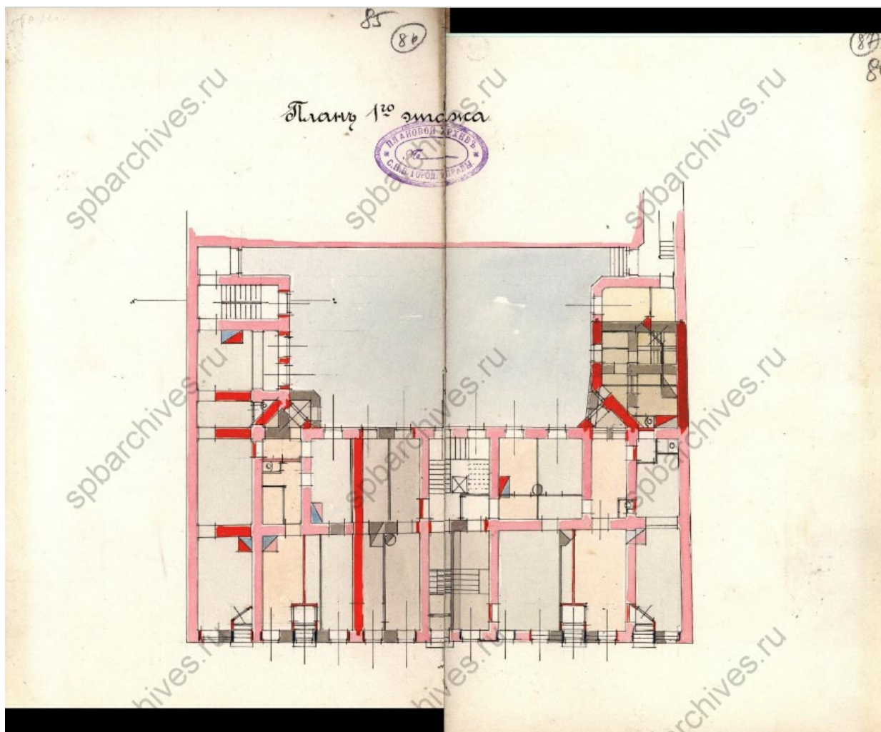
32. План 1-го этажа. Чертежи дома на участке, принадлежавшем Д. Колотушкину, А. Колотушкину, Е. Герварт, Н. Ф. Заремба, П. Н. Глаголеву по наб. р. Фонтанки, 103. ЦГИА СПб. Фонд 513. Описание 102. Дело 9949. 1826–1912 гг. л. 85-86;
