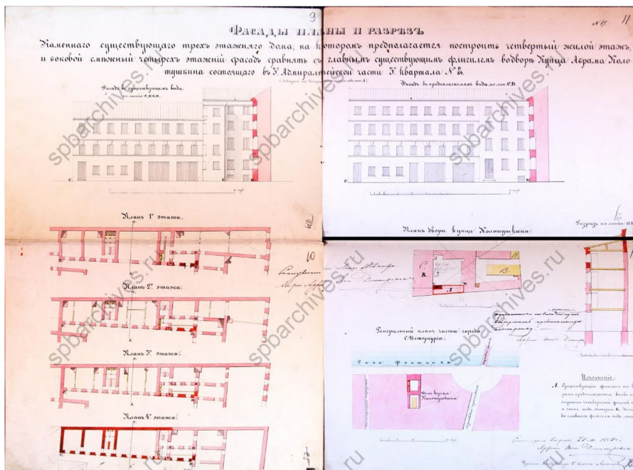
9. Фасады, планы и разрез. Чертежи дома на участке, принадлежавшем Д.Колотушкину, А.Колотушкину, Е.Герварт, Н.Ф.Заремба, П.Н.Глаголеву по наб.р.Фонтанки, 103. ЦГИА СПб. Фонд 513. Опись 102. Дело 9949. 1826–1912 гг. л. 9-12;
