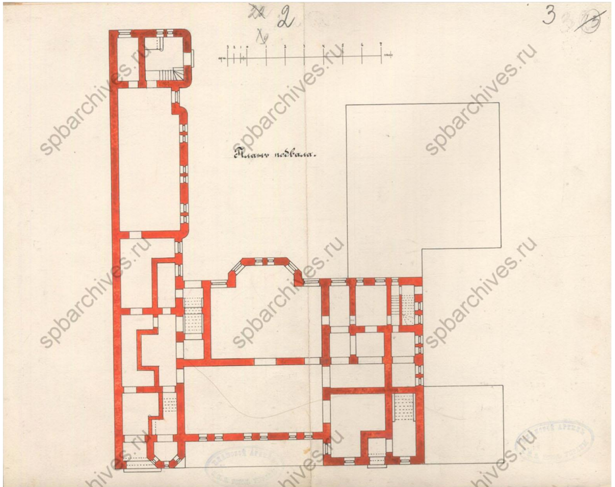
Илл. 3. План подвала. ЦГИА СПб. Ф.513 Оп.102 Д.1544. Чертежи дома на участке, принадлежавшем П.П.Форостовскому по 4-й линии В.О., 9. 1900 г.
