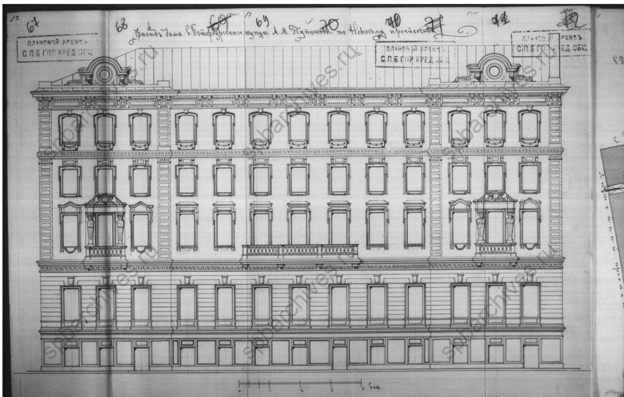
Илл.21. Фасад Санкт-Петербургского купца А.М. Тупикова. ЦГИА СПб. Фонд 515. Описание 4. Дело 3916.1895 г. Чертежи дома А.М.Тупикова по Невскому пр.,78 и Литейному пр.,64
