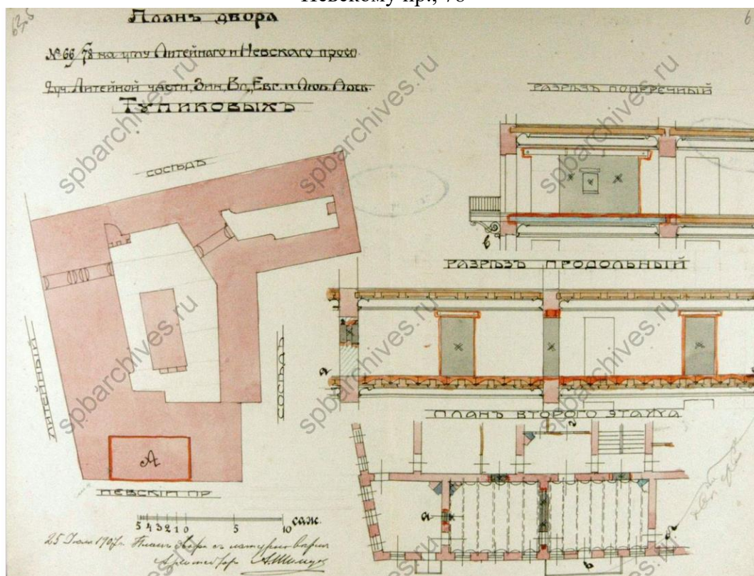
Илл.26. План двора 1907 г. ЦГИА СПб: Фонд 513, опись 102, дело 4241 "Чертежи дома на участке, принадлежавшем Кокореву, А.М.Тупикову, наследникам Тупиковым, совладельцам З.В.Четыркиной, Е.А.Карпинской и Л.А.Марковой по Литейному пр., 64 и Невскому пр., 78"
