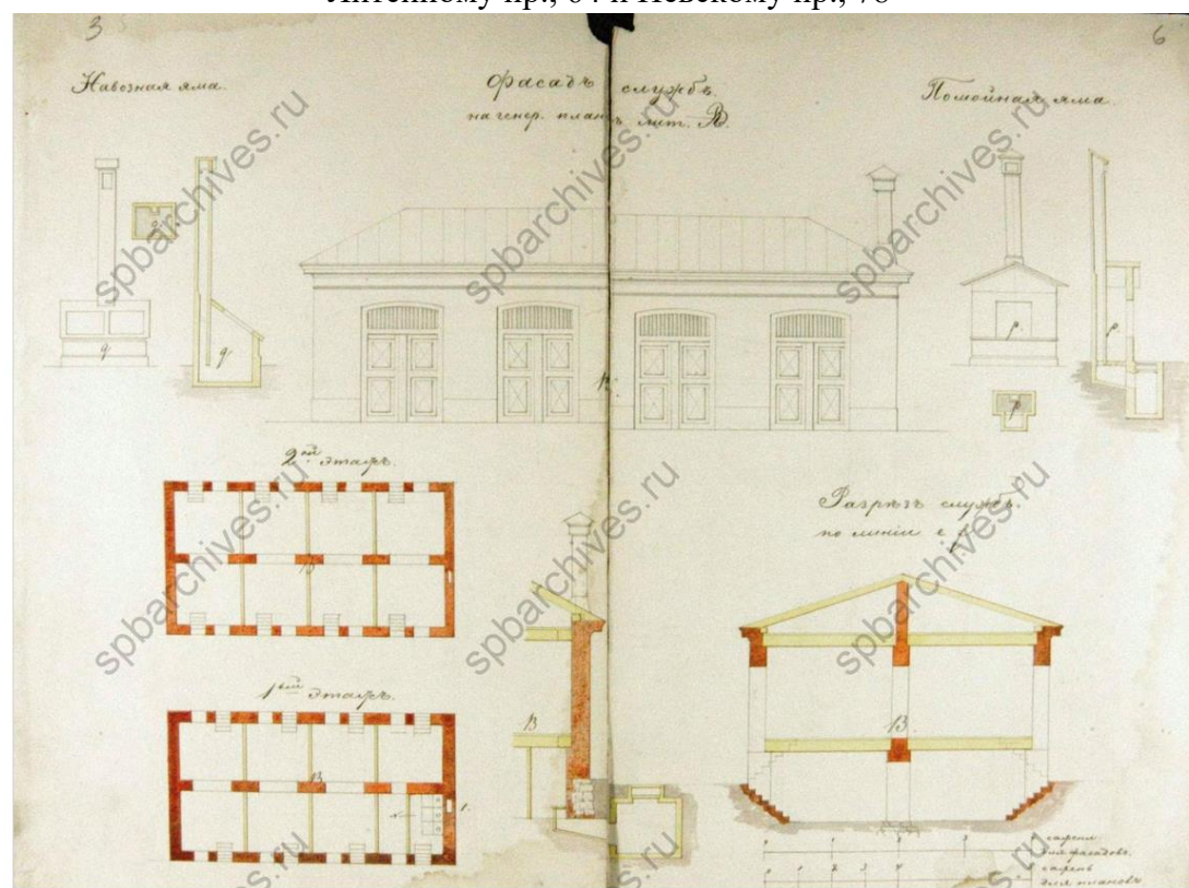
Илл.10. Фасад службы. Лит. В ЦГИА СПб: Фонд 513, опись 102, дело 4241 "Чертежи дома на участке, принадлежавшем Кокореву, А.М.Тупикову, наследникам Тупиковым, совладельцам З.В.Четыркиной, Е.А.Карпинской и Л.А.Марковой по Литейному пр., 64 и Невскому пр., 78"
