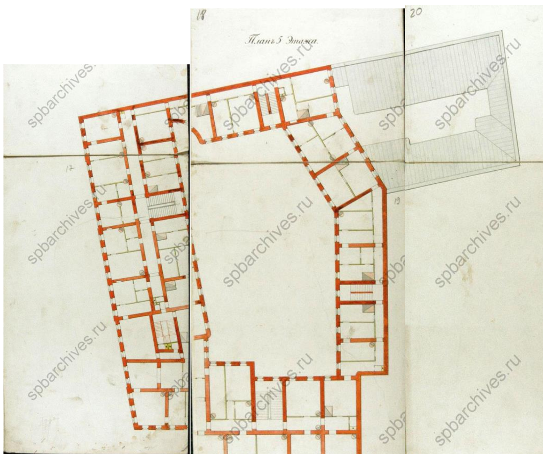
Илл. 17. План 5 – го этажа. 1874 г. ЦГИА СПб: Фонд 513, опись 102, дело 4241 "Чертежи дома на участке, принадлежавшем Кокореву, А.М.Тупикову, наследникам Тупиковым, совладельцам З.В.Четыркиной, Е.А.Карпинской и Л.А.Марковой по Литейному пр., 64 и Невскому пр., 78"
