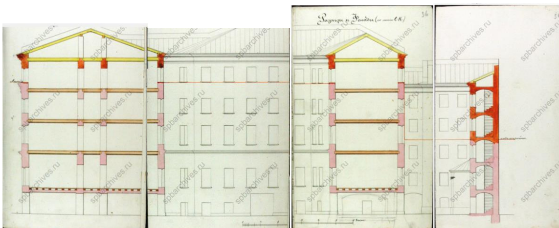
Илл. 16. Разрезы по дворовым фасадам.. 1874 г. ЦГИА СПб: Фонд 513, опись 102, дело 4241 "Чертежи дома на участке, принадлежавшем Кокореву, А.М.Тупикову, наследникам Тупиковым, совладельцам З.В.Четыркиной, Е.А.Карпинской и Л.А.Марковой по Литейному пр., 64 и Невскому пр., 78"
