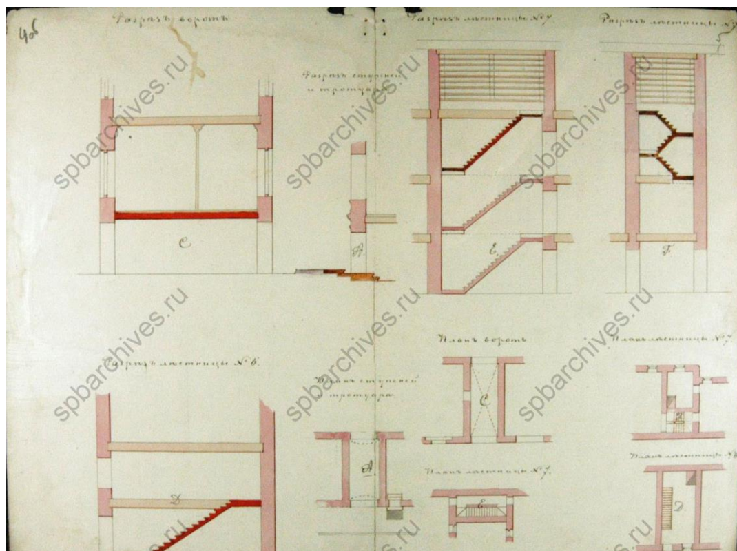
Илл. 9 Фрагменты разрезов здания. ЦГИА СПб: Фонд 513, опись 102, дело 4241 "Чертежи дома на участке, принадлежавшем Кокореву, А.М.Тупикову, наследникам Тупиковым, совладельцам З.В.Четыркиной, Е.А.Карпинской и Л.А.Марковой по Литейному пр., 64 и Невскому пр., 78"
