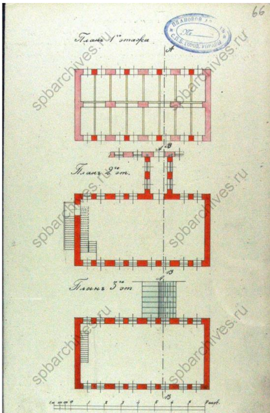
Илл.28. Устройство пристройки. План здания. Начало XX века. ЦГИА СПб: Фонд 513, опись 102, дело 4241 "Чертежи дома на участке, принадлежавшем Кокореву, А.М.Тупикову, наследникам Тупиковым, совладельцам З.В.Четыркиной, Е.А.Карпинской и Л.А.Марковой по Литейному пр., 64 и Невскому пр., 78"
