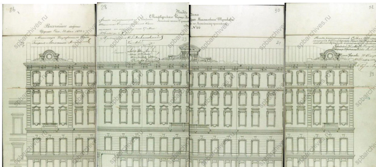
Илл.13. Лицевой фасад здания по Литейному проспекту. 1874 г. ЦГИА СПб: Фонд 513, опись 102, дело 4241 "Чертежи дома на участке, принадлежавшем Кокореву, А.М.Тупикову, наследникам Тупиковым, совладельцам З.В.Четыркиной, Е.А.Карпинской и Л.А.Марковой по Литейному пр., 64 и Невскому пр., 78"
