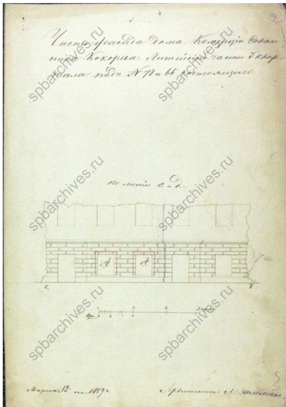
Илл.8. Фрагмент фасада здания дома Тупикова 1839 г. ЦГИА СПб: Фонд 513, опись 102, дело 4241 "Чертежи дома на участке, принадлежавшем Кокореву, А.М.Тупикову, наследникам Тупиковым, совладельцам З.В.Четыркиной, Е.А.Карпинской и Л.А.Марковой по Литейному пр., 64 и Невскому пр., 78"
