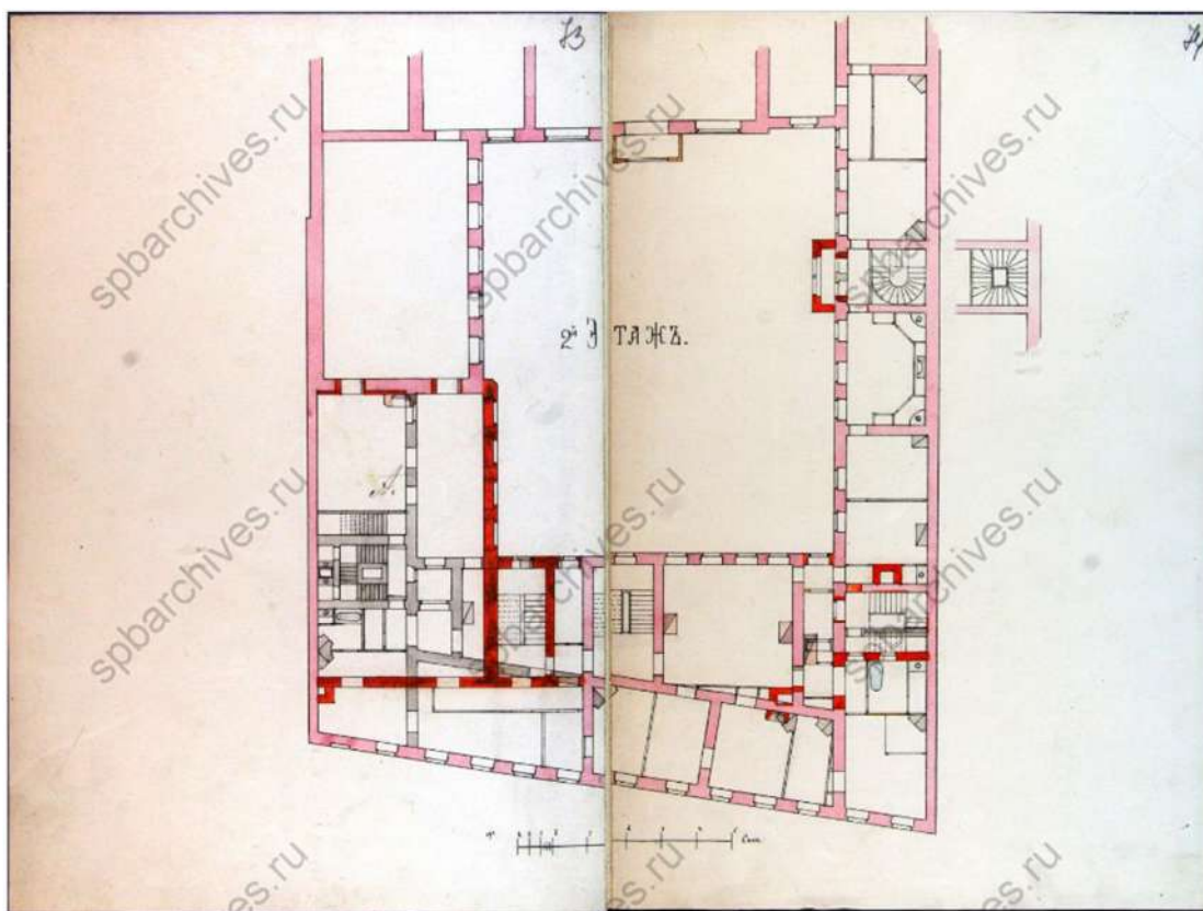
Илл. 27. Месмахер М.Е. Проект перестройки. План 2-3 этажа. 1887 г. ЦГИА СПб
