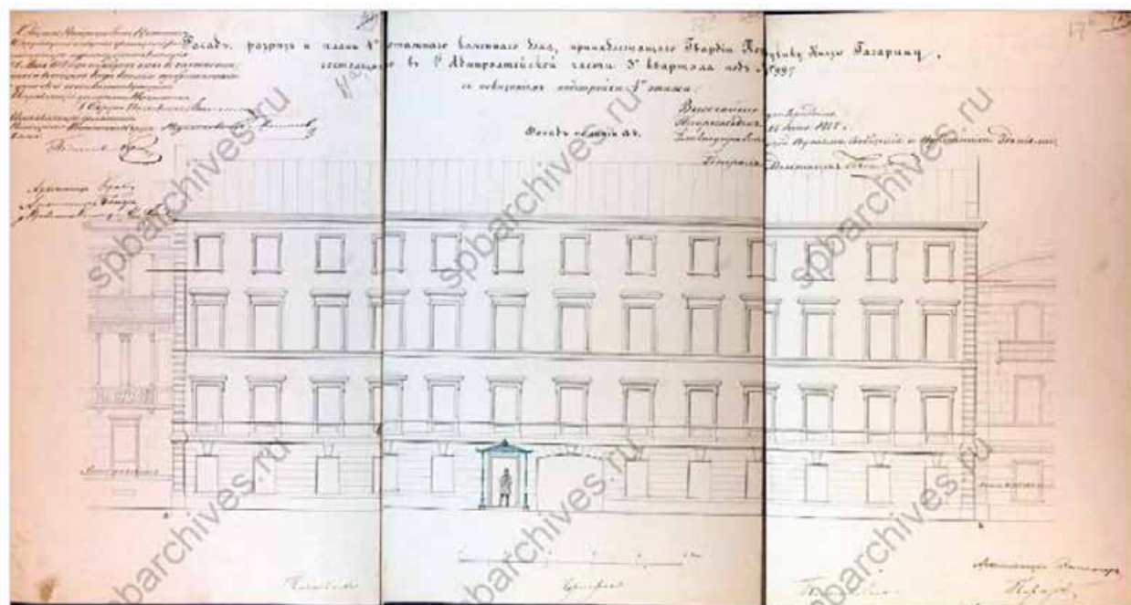
Илл. 11. Эппингер Ф.И. Проект надстройки дома № 99 на набережной Мойки. 1858 г. ЦГИА СПб
