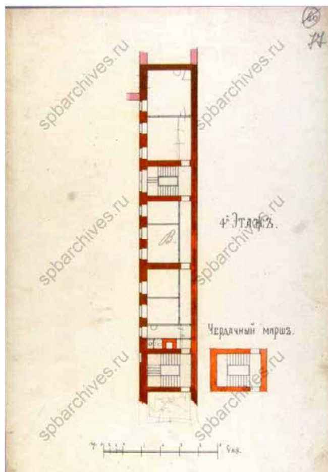
Илл. 29. Месмахер М.Е. Проект перестройки. План 4 этажа и чердачный марш. 1887 г. ЦГИА СПб
