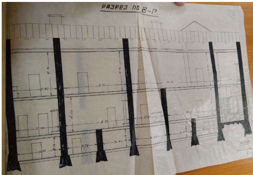
Илл. 67. Разрез по оси В-Г (восток-запад). 1934 г. Фрагмент. ЦГА СПб
