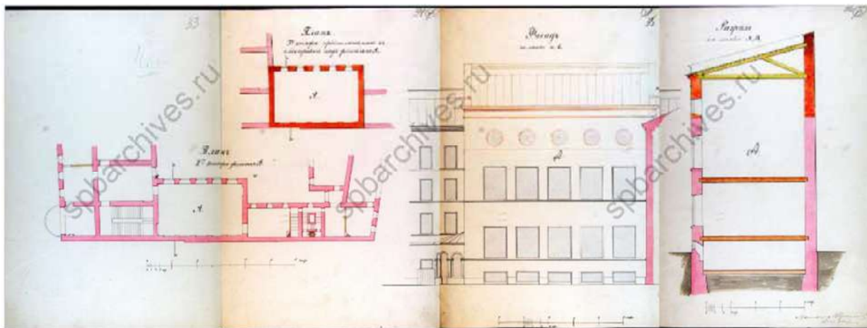
Илл. 16. Брюллов Н.Ф. План надстройки третьим этажом дворового флигеля. 1870 г. ЦГИА СПб
