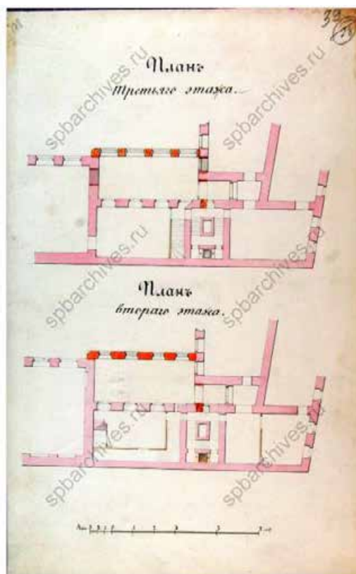
Илл. 19. Брюллов Н.Ф. План надстройки западного дворового флигеля. Второй и третий этаж. 1873 г.
