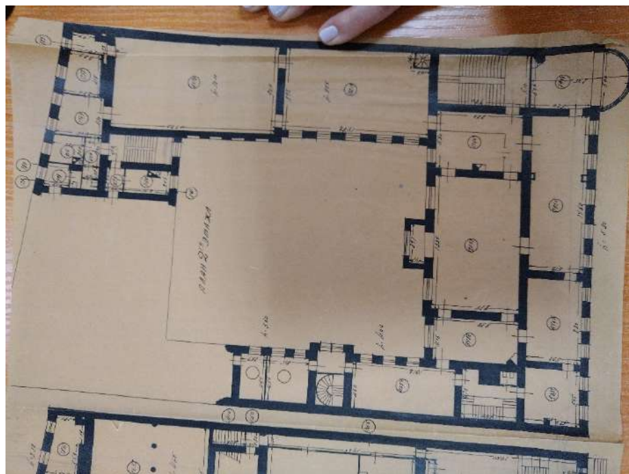
Илл. 63. План второго этажа. 1934 г. Фрагмент. ЦГА СПб
