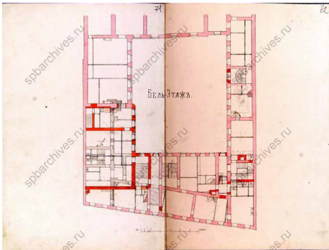
Илл. 26. Месмахер М.Е. Проект перестройки. План 1-2 этаж. 1887 г. ЦГИА СПб.
