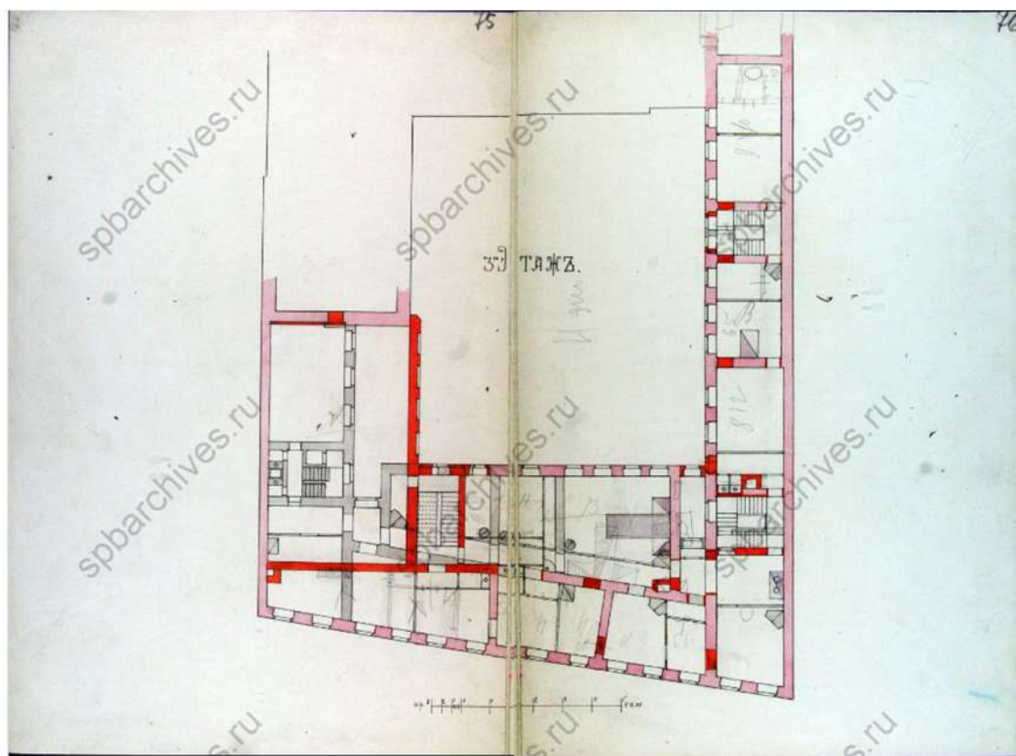
Илл. 28. Месмахер М.Е. Проект перестройки. План 3-4 этажа. 1887 г. ЦГИА СПб.
