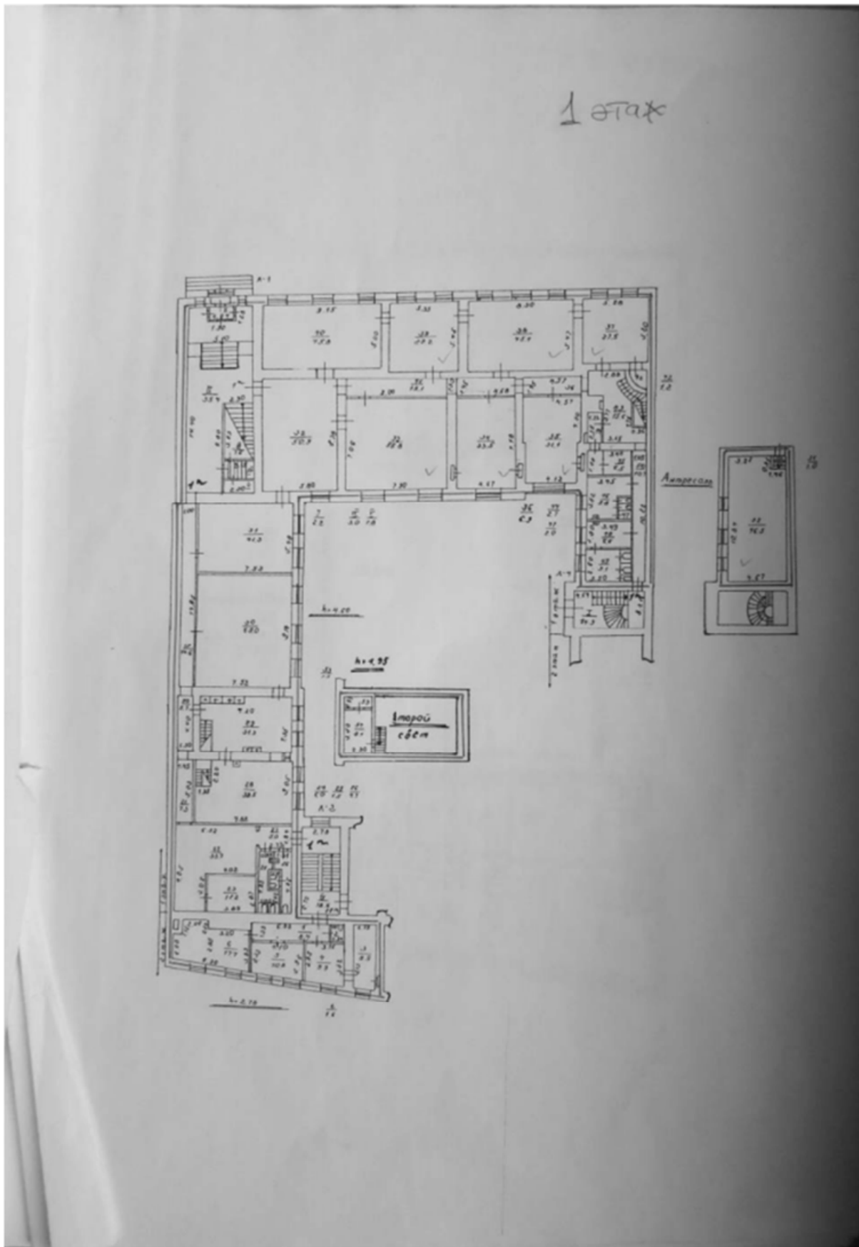
Илл.82. План 1 этажа. 2005 г. Архив ГУИОН ПИБ Адмиралтейского района.
