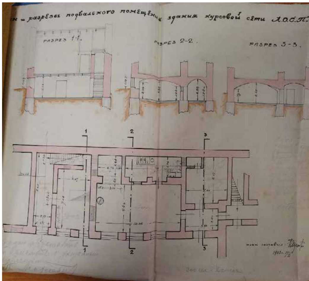
Илл. 55. Разрез подвально помещения здания курсовой сети. 1932 г. ЦГА СПб
