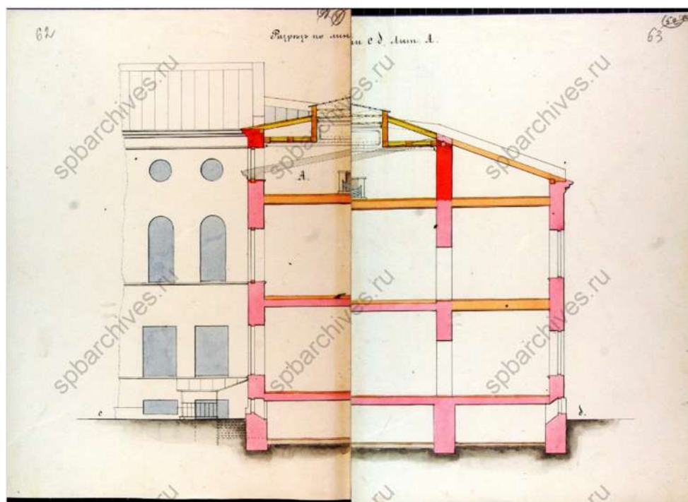
Илл.23. Петерсон Л.Л. План надстройки чердачного этажа корпуса по Большой морской улице. 1875 г. ЦГИА СПб
