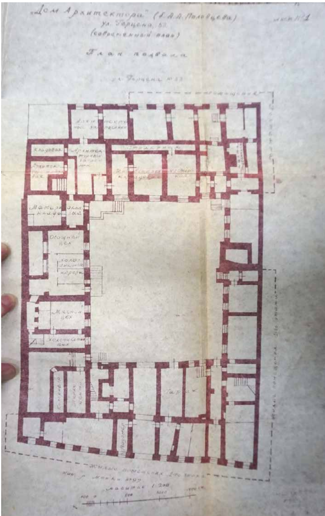
Илл. 76. План подвала. 1973 г. Архив КГИОП.
