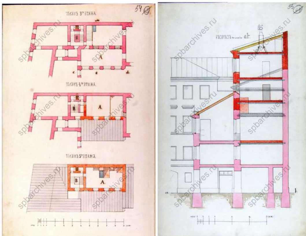
Илл. 21. Петерсон Л.Л. Проект надстройки пятым этажом части дворового корпуса. План. Разрез. 1875 г. ЦГИА СПб
