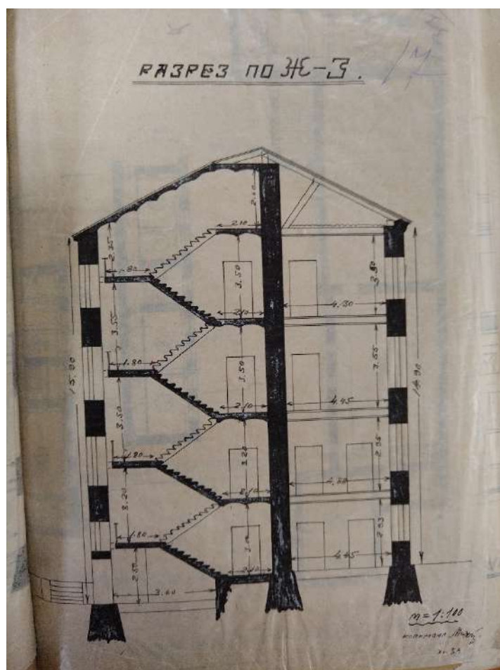
Илл.68. Западный флигель. Разрез по оси Ж-З (восток-запад). 1934 г. ЦГА СПб
