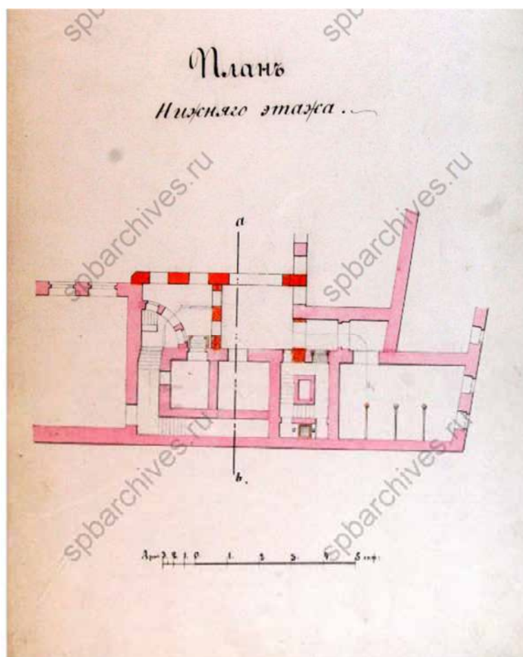
Илл. 18. Брюллов Н.Ф. План надстройки западного дворового флигеля. Нижний этаж. 1873 г.
