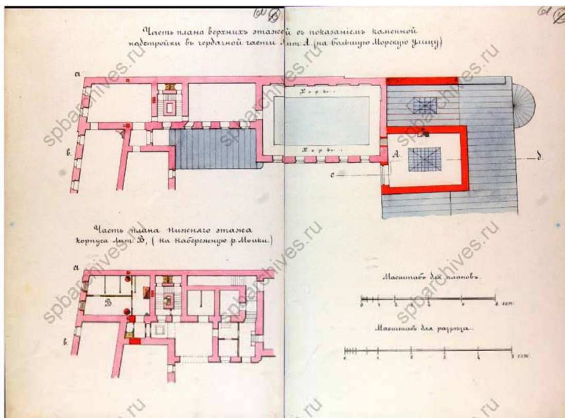
Илл. 22. Петерсон Л.Л. План надстройки чердачного этажа корпуса по Большой морской улице. 1875 г. ЦГИА СПб
