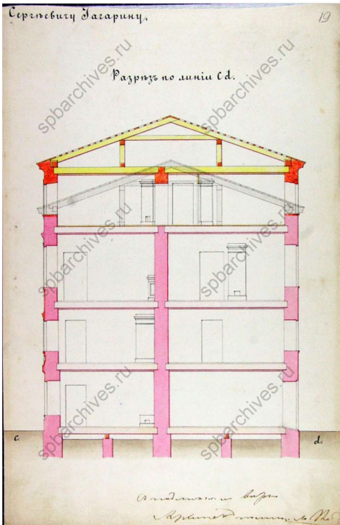
Илл. 13. Эпшингер Ф.И. Проект надстройки 4-м этажом. 1858 г. ЦГИА СПб
