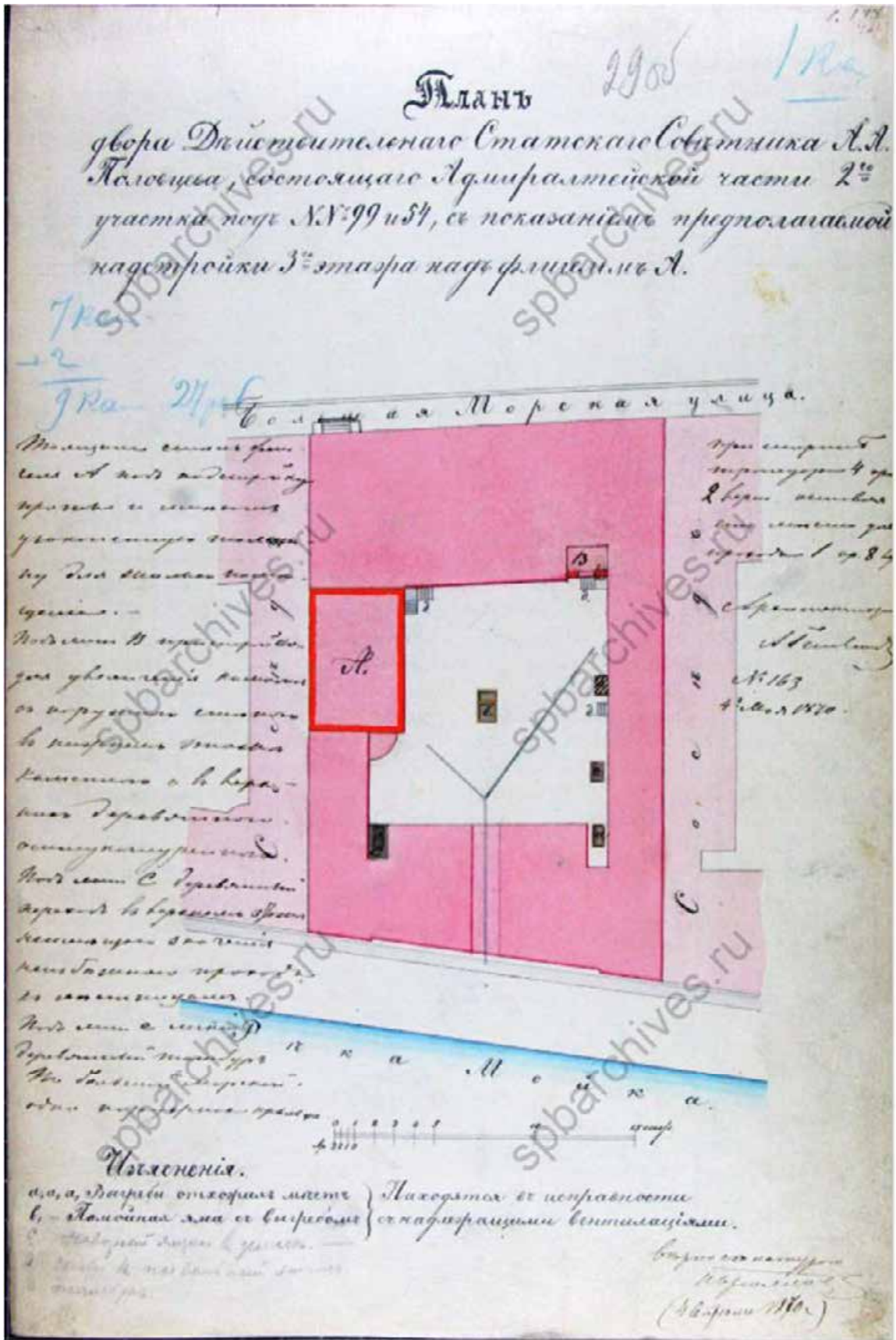
Илл. 15. Брюллов Н.Ф. Проект надстройки 3-м этажом. 1870 г. ЦГИА СПб
