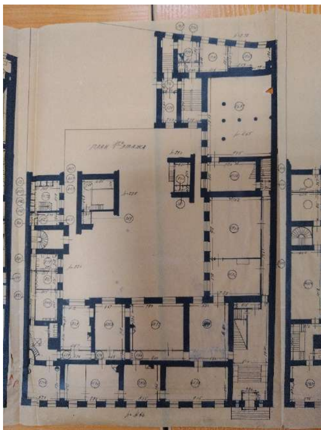
Илл. 62. План первого этажа. 1934 г. Фрагмент. ЦГА СПб
