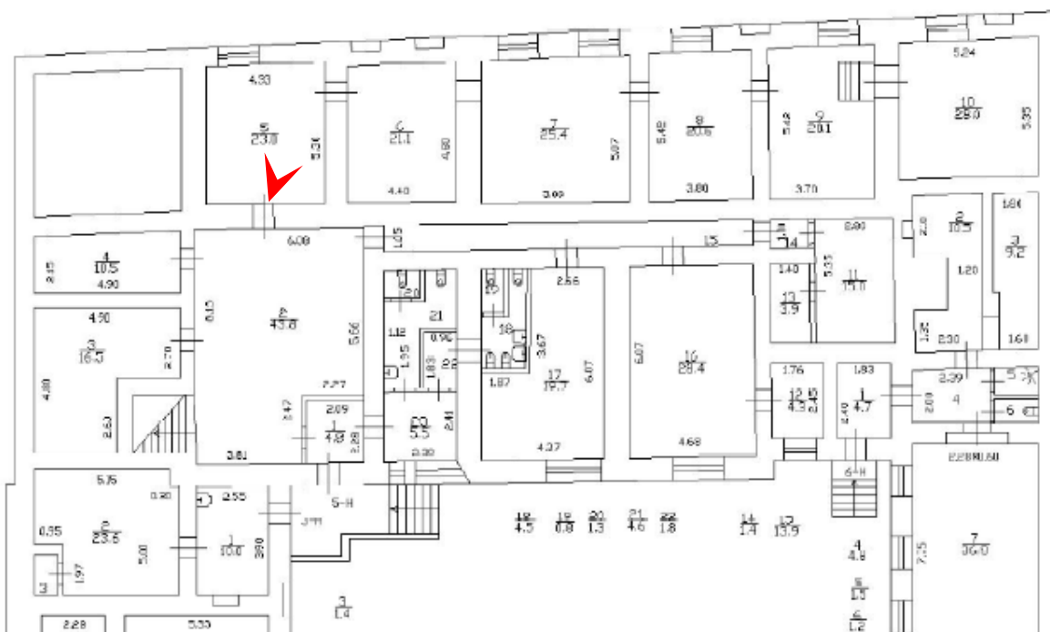
24. «Дом Половцова А.А. с дворовыми флигелями» - объект культурного наследия федерального значения по адресу: Санкт-Петербург, Большая Морская ул., 52, р.Мойки наб., 97 План подвала и 1-го этажей Помещение 5-Н (5) Дата съемки: 20 августа 2023 года
