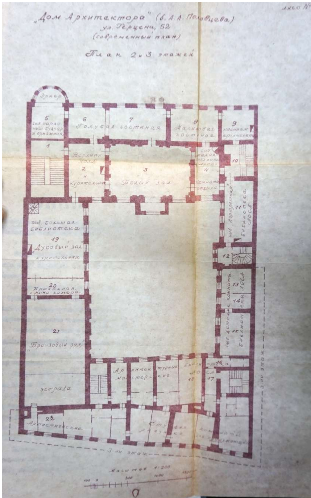
Илл.78. План 2 и 3 этажей. 1973 г. Архив КГИОП.
