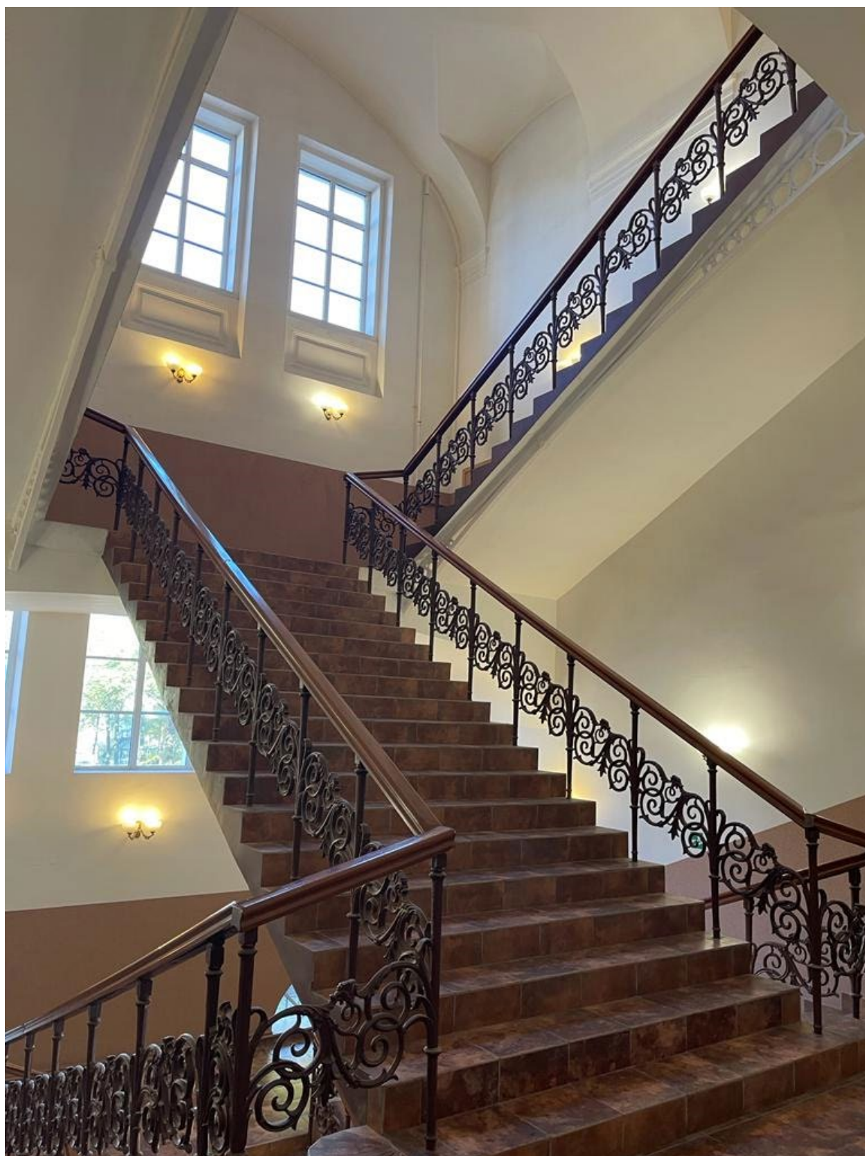
Фото 10. Марш на площадку между вторым и третьим этажами. Косоуры.
