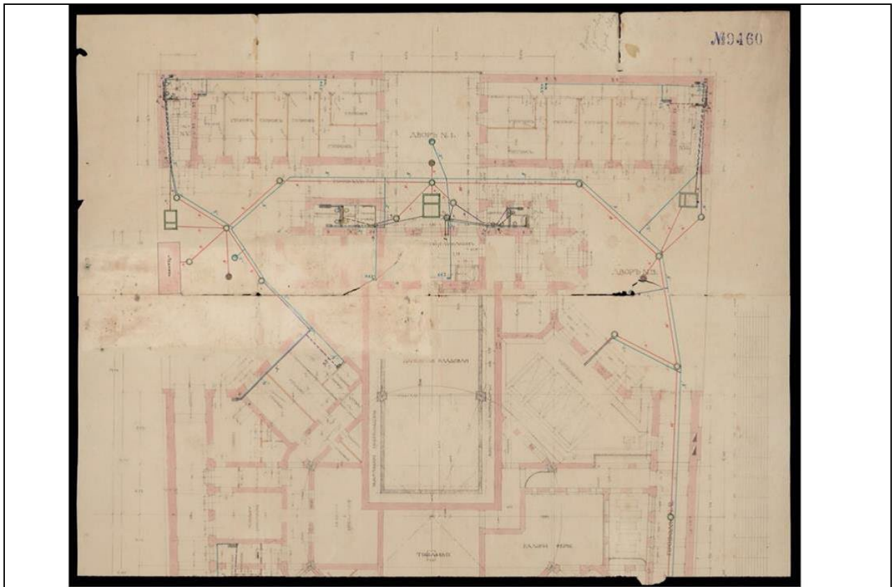
3. Здание Главного Казначейства в СПб. План первого этажа. 1914 г. РГИА. Ф. 565. Оп. 2. Д. 5630. Л. 6. Фрагмент
