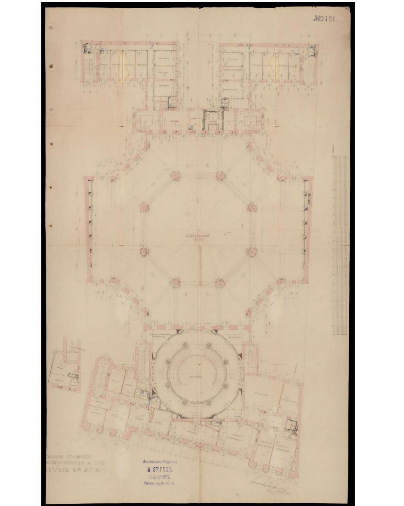
5. Здание Главного Казначейства в СПб. План второго этажа. 1914 г. РГИА. Ф. 565. Оп. 2. Д. 5630. Л. 8
