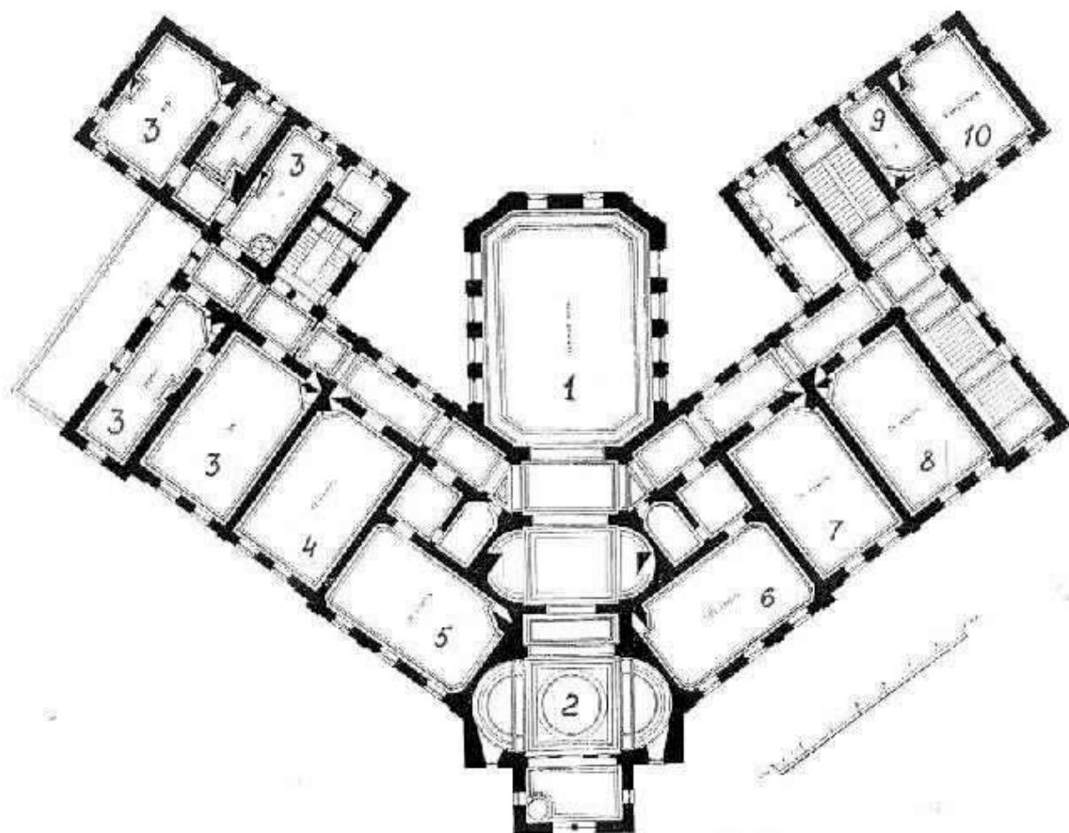
5. План второго этажа Николаевской гимназии. 1895 год. Под № 2 – Церковь.
