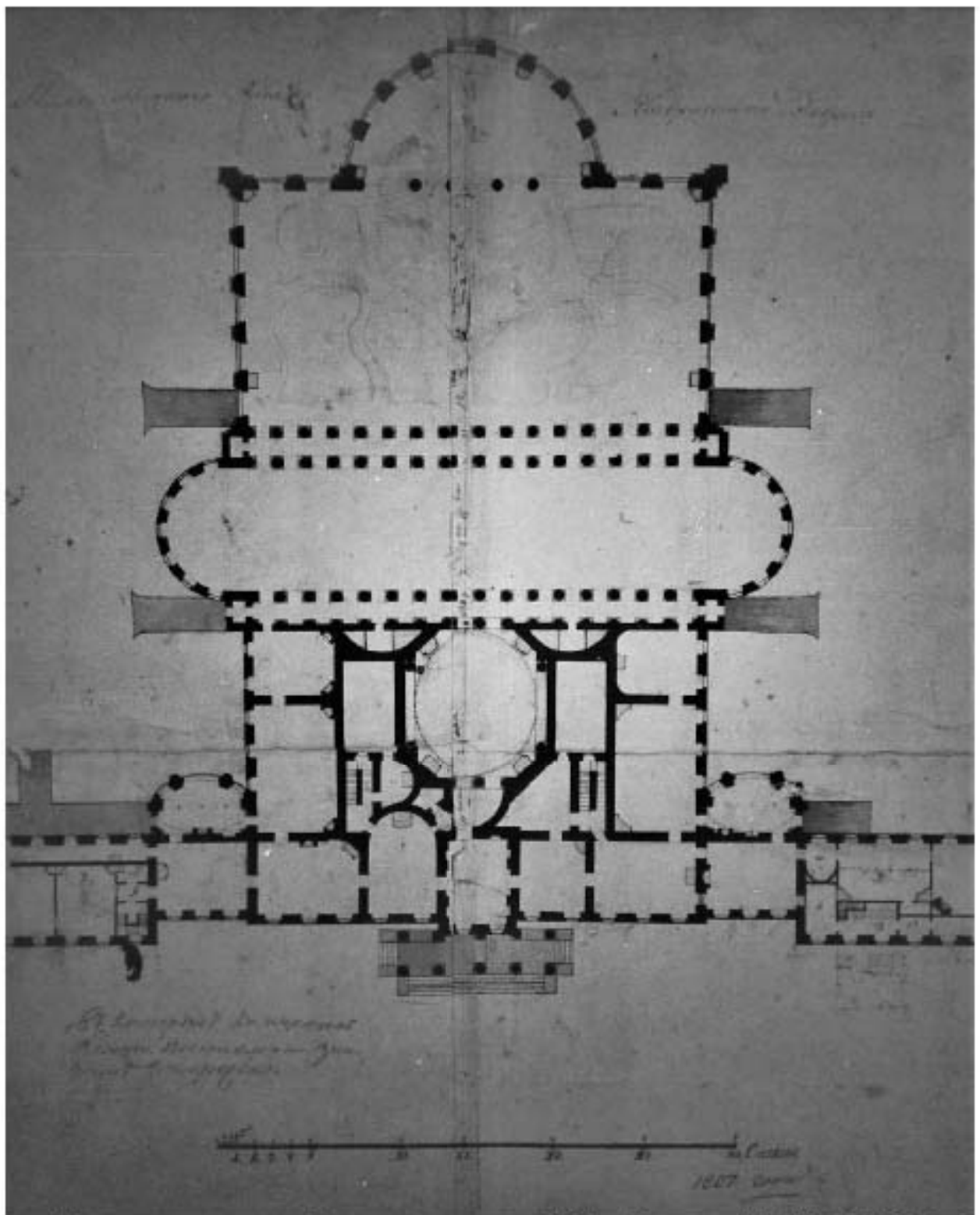
6. План нижнего этажа Таврического дворца. 1807 г. Фрагмент // РГИА. Ф. 485. Оп. 2. Д. 804. Л.
