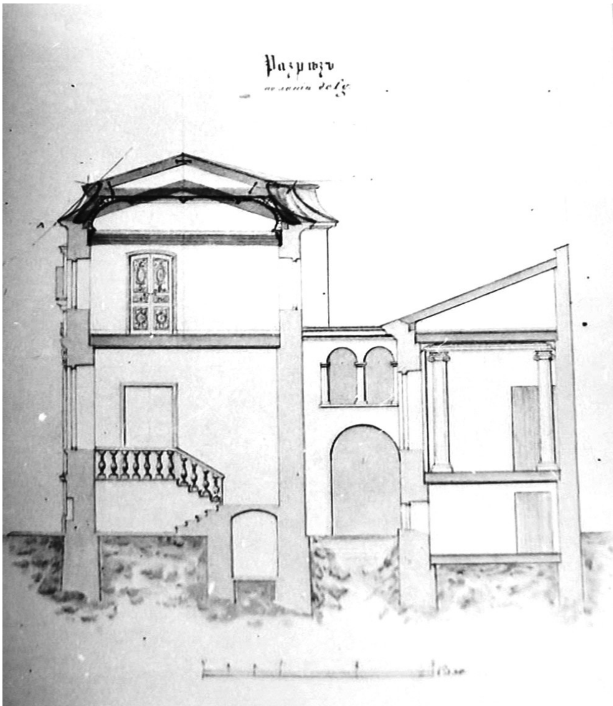
67. Дом жены тайного советника А. К. Ламанской. Разрез жилого дома. 1887г. ЦГИА СПб, ф. 513, оп. 102, д. 3389, л. 22.
