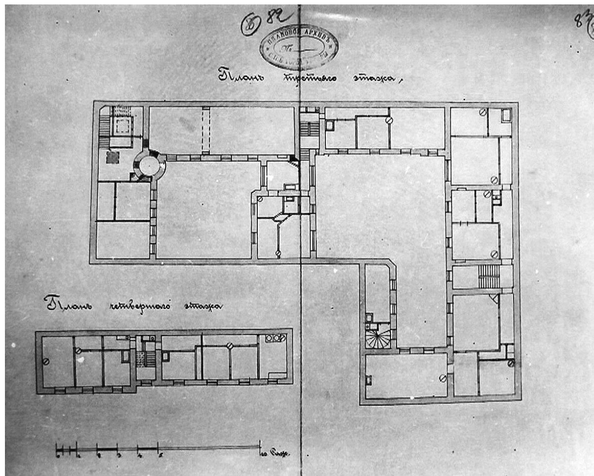
52. Дом Я. В. Ратькова-Рожнова. План третьего этажа. План четвертого этажа. 1910 г. Архитектор В. П. Цейдлер. ЦГИА СПб, ф. 513, оп. 102, д. 3388, л. 82, 83.
