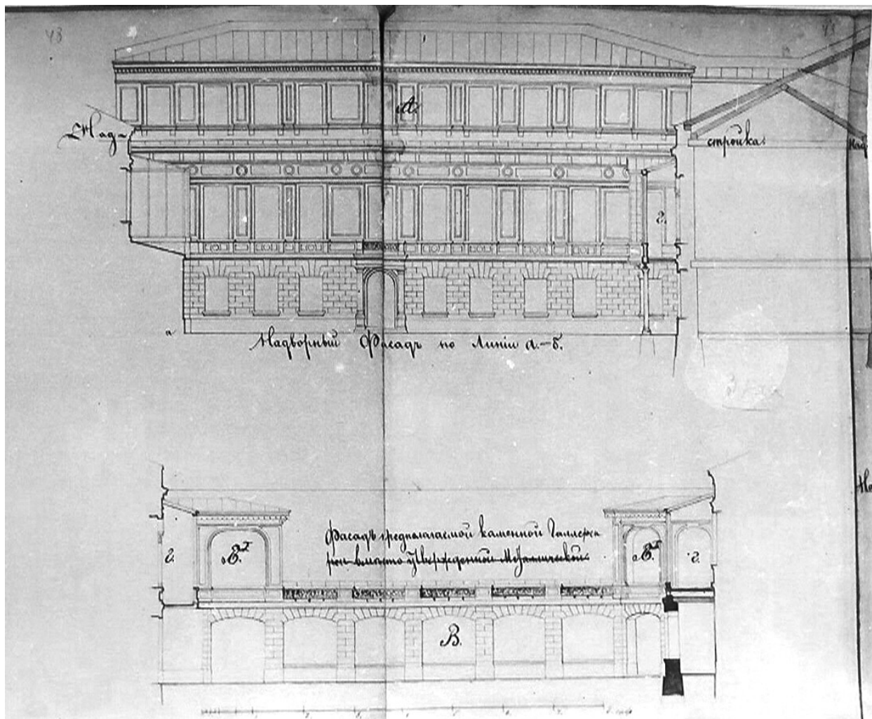
32. Дом В. И. Мятлева. Северный двор. Проект надстройки надворного фасада А третьим этажом по линии а-б. Фасад предполагаемой каменной галереи. 1870 г. Архитектор И. И. Цим. ЦГИА СПб, ф. 513, оп. 102, д. 3388, л. 43 - 45.
