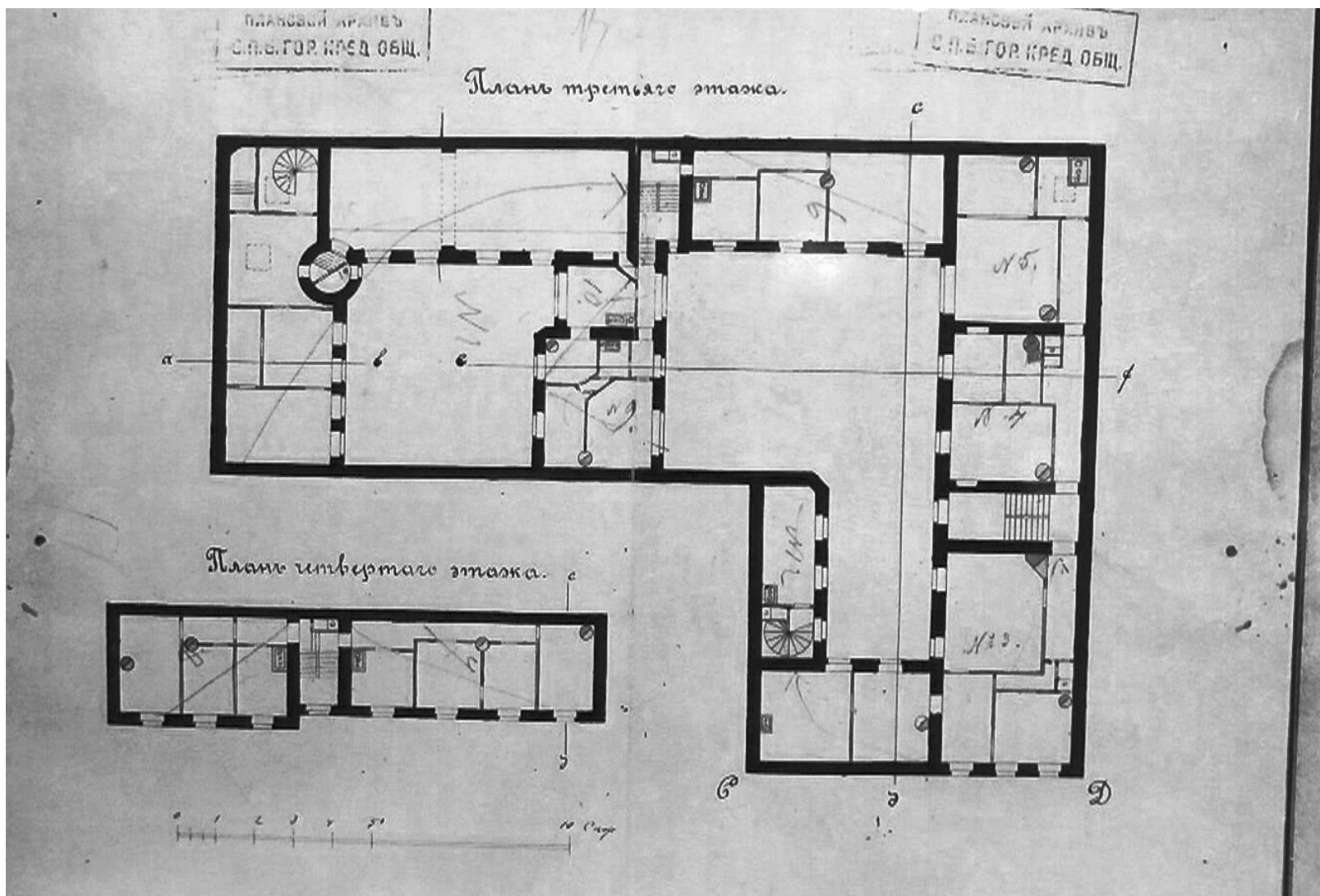
47. Дом графини Л. П. Бутурлиной. План III и IV этажей. 1904 г. ЦГИА СПб, ф. 515, оп. 4, д. 3524, л. 13 - 14.
