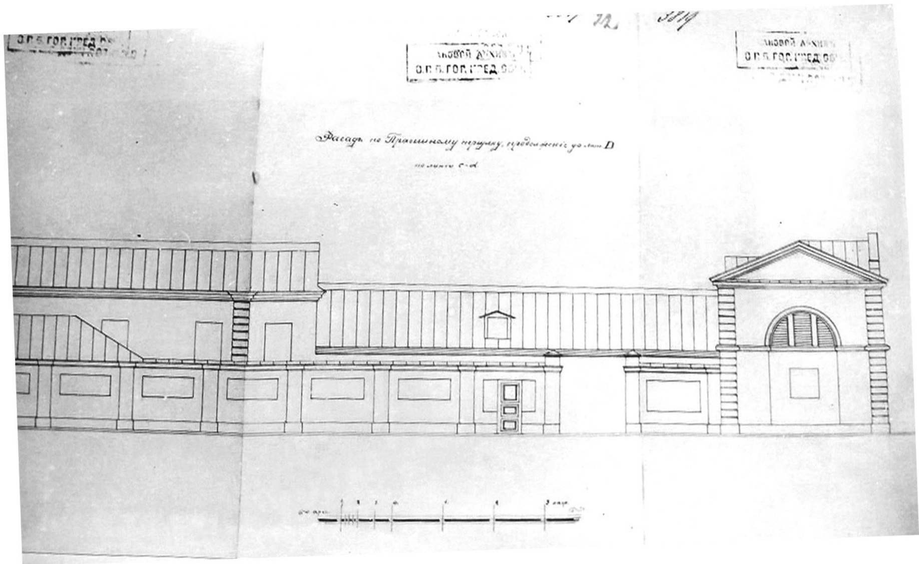
72. Дом А. Е. Бодиско. Фасад по Прачешному переулку (южная часть). 1913 г. ЦГИА СПб, ф. 515, оп. 4, д. 3525, л. 21, 22, 23.
