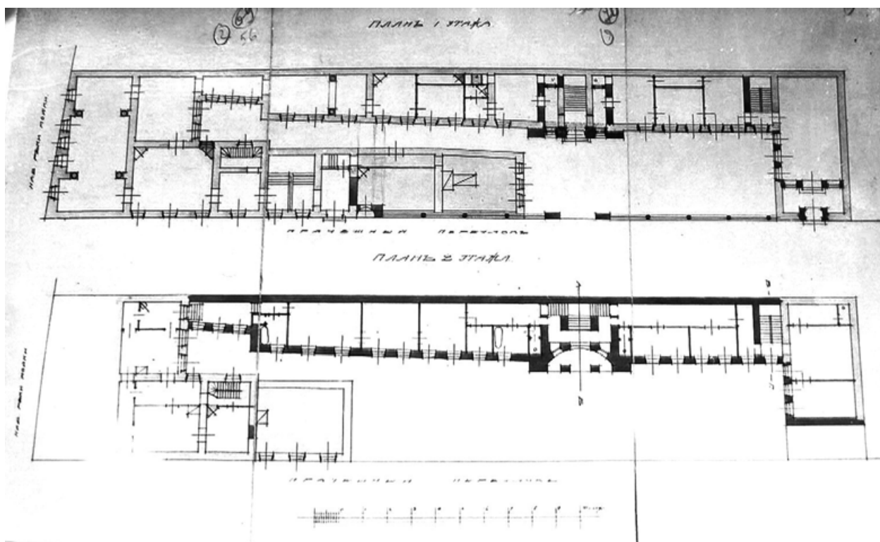
78. Дом Я. В. Ратькова-Рожнова, состоящий в Казанской части 3-го участка, по набережной реки Мойки и Прачешному переулку, № 88. 1917 г. План I этажа, проект переустройства. План II этажа, проект переустройства. Академик архитектуры М. С. Лялевич. ЦГИА СПб, ф. 513, оп. 102, д. 3389, л. 69, 70, 71.
