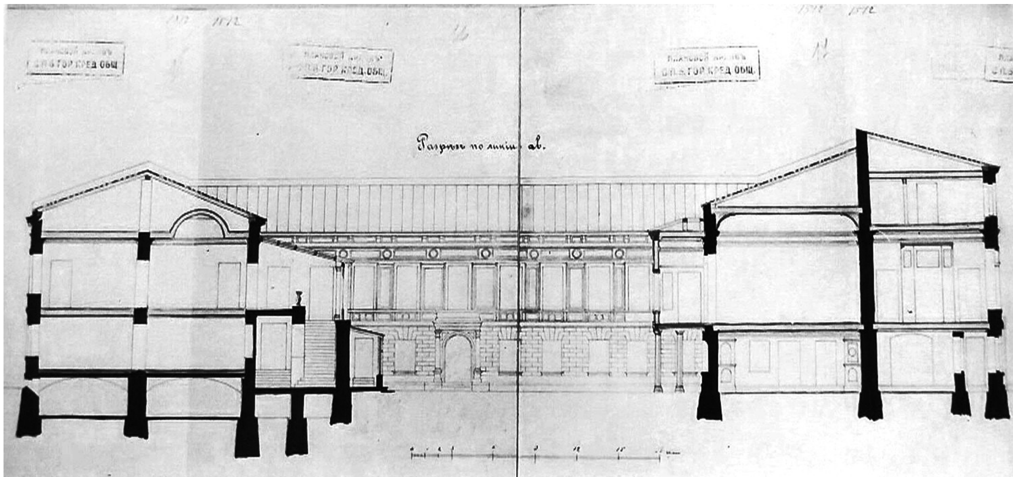
48. Дом графини Л. П. Бутурлиной. Северный двор. Разрез по линии А. 1904 г. ЦГИА СПб, ф. 515, оп. 4, д. 3524, л. 15 - 17.
