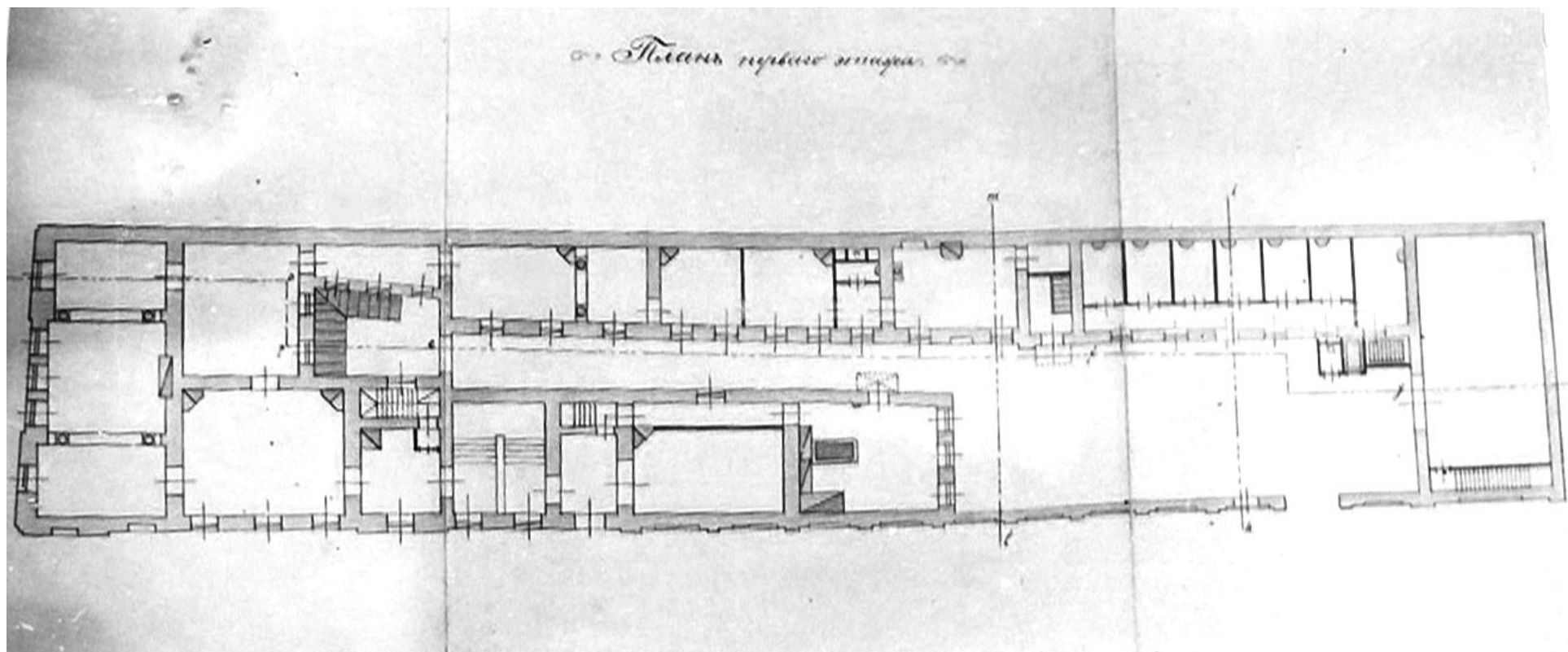
74. Дом А. Е. Бодиско. План первого этажа. 1913 г. ЦГИА СПб, ф. 515, оп. 4, д. 3525, л. 27, 28, 29.
