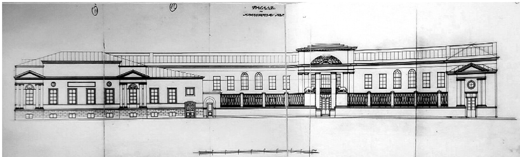
80. Дом Я. В. Ратькова-Рожнова, состоящий в Казанской части 3-го участка, по набережной реки Мойки и Прачешному переулку, № 88. 1917 г. Фасады по Прачешному переулку. Проект. Академик архитектуры М. С. Лялевич. ЦГИА СПб, ф. 513, оп. 102, д. 3388, л. 78-82.
