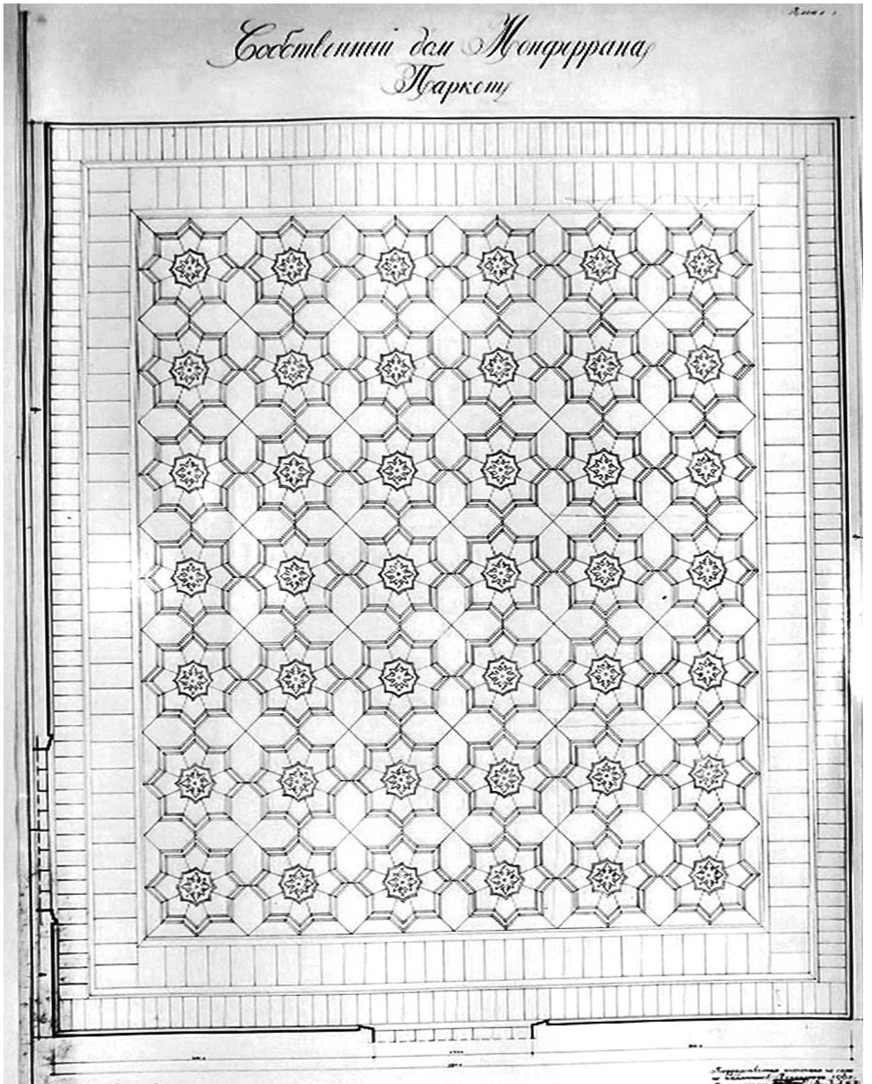
124. Наб. реки Мойки, 86-88. 2 этаж. Паркет в гостиной (рядом с эркером). Обмерный чертеж. КГИОП СПб, рег. 35437.
