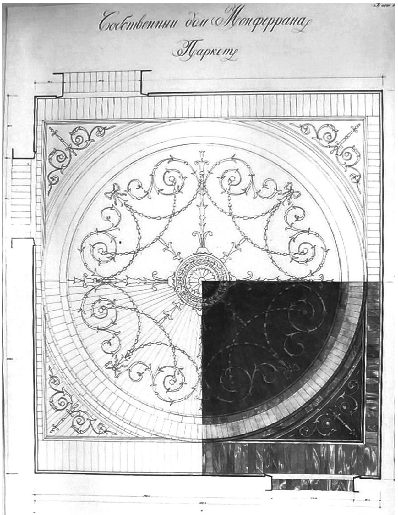
125. Наб. реки Мойки, 86-88. 2 этаж. Лицевая угловая комната. Паркет. Обмерный чертеж. КГИОП СПб, нег. 35438.
