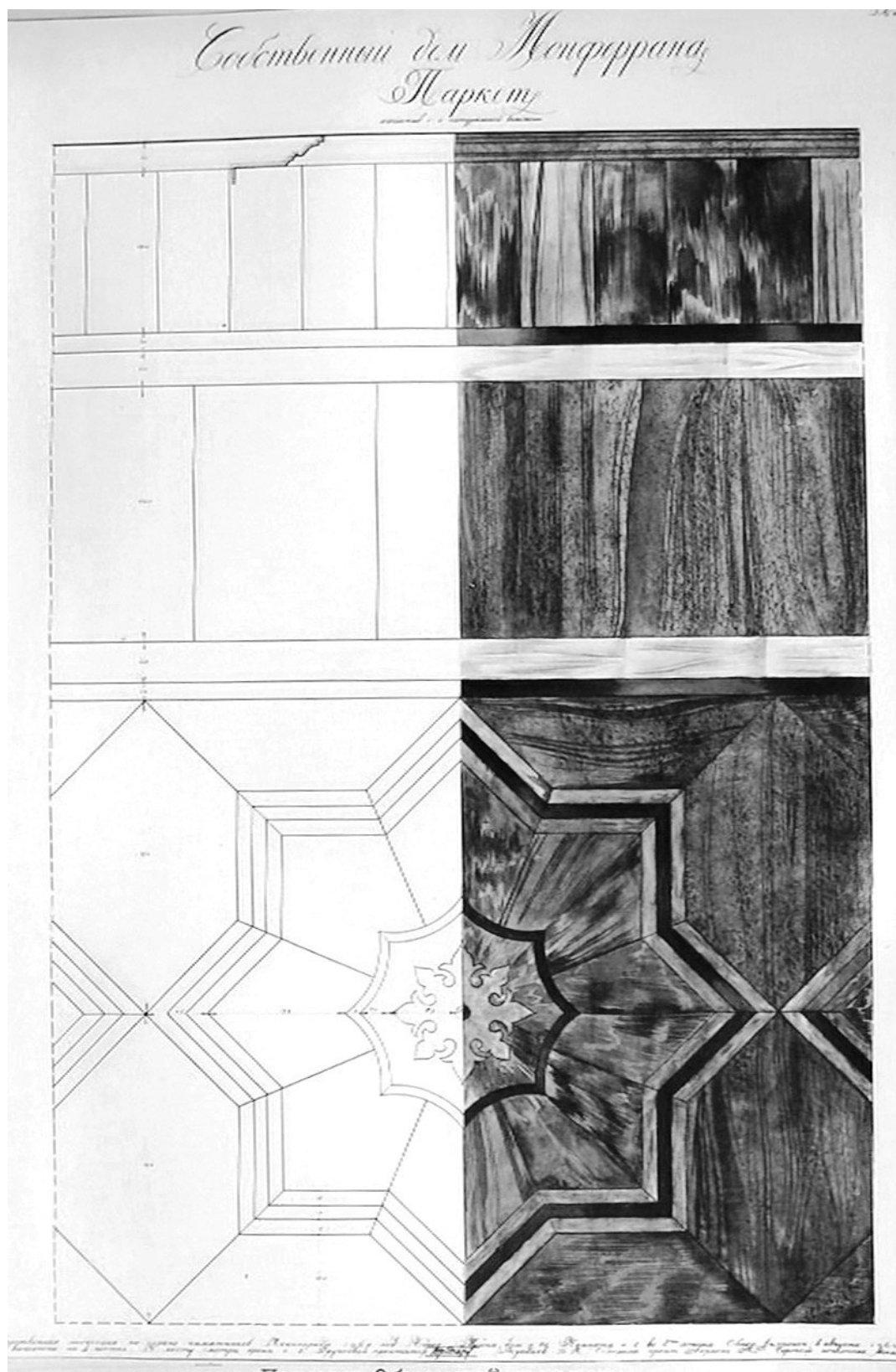
122. Наб. реки Мойки, 86-88. 2 этаж. Паркет в гостиной (рядом с эркером). Обмерный чертеж. КГИОП СПб, инв. 35435.
