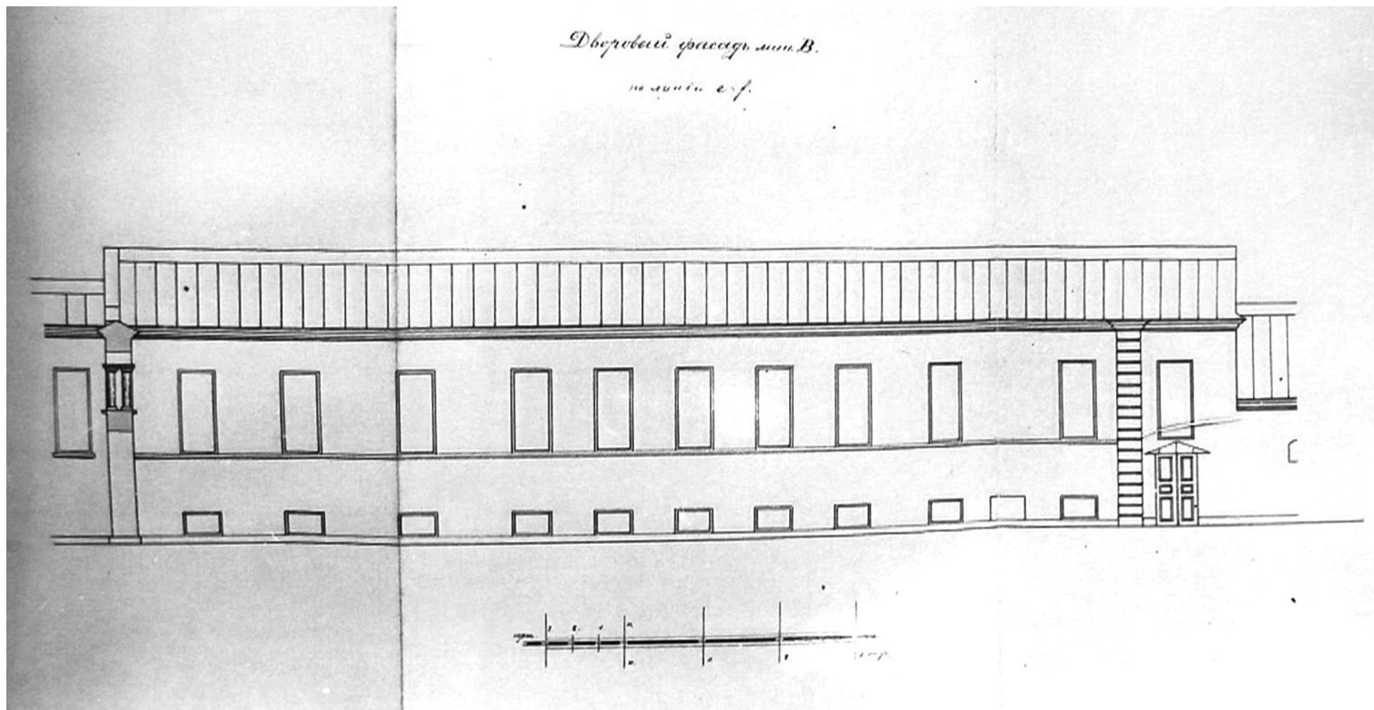
76. Дом А. Е. Бодиско. Дворовый фасад по линии В (служебный флигель). 1913 г. ЦГИА СПб, ф. 515, оп. 4, д. 3525, л. 33, 34, 35.
