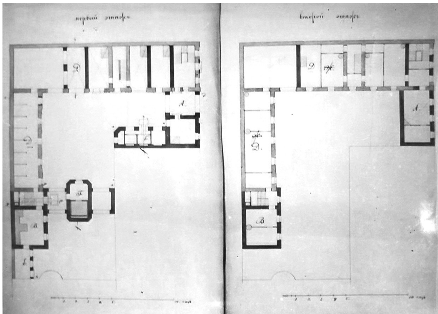
36. Дом коллежского советника В. И. Мятлева. Центральный и южный двор. План I этажа. План II этажа. 1871 г. Архитектор И. И. Цим. ЦГИА СПб, ф. 513, оп. 102, д. 3388, л. 35 - 36.
