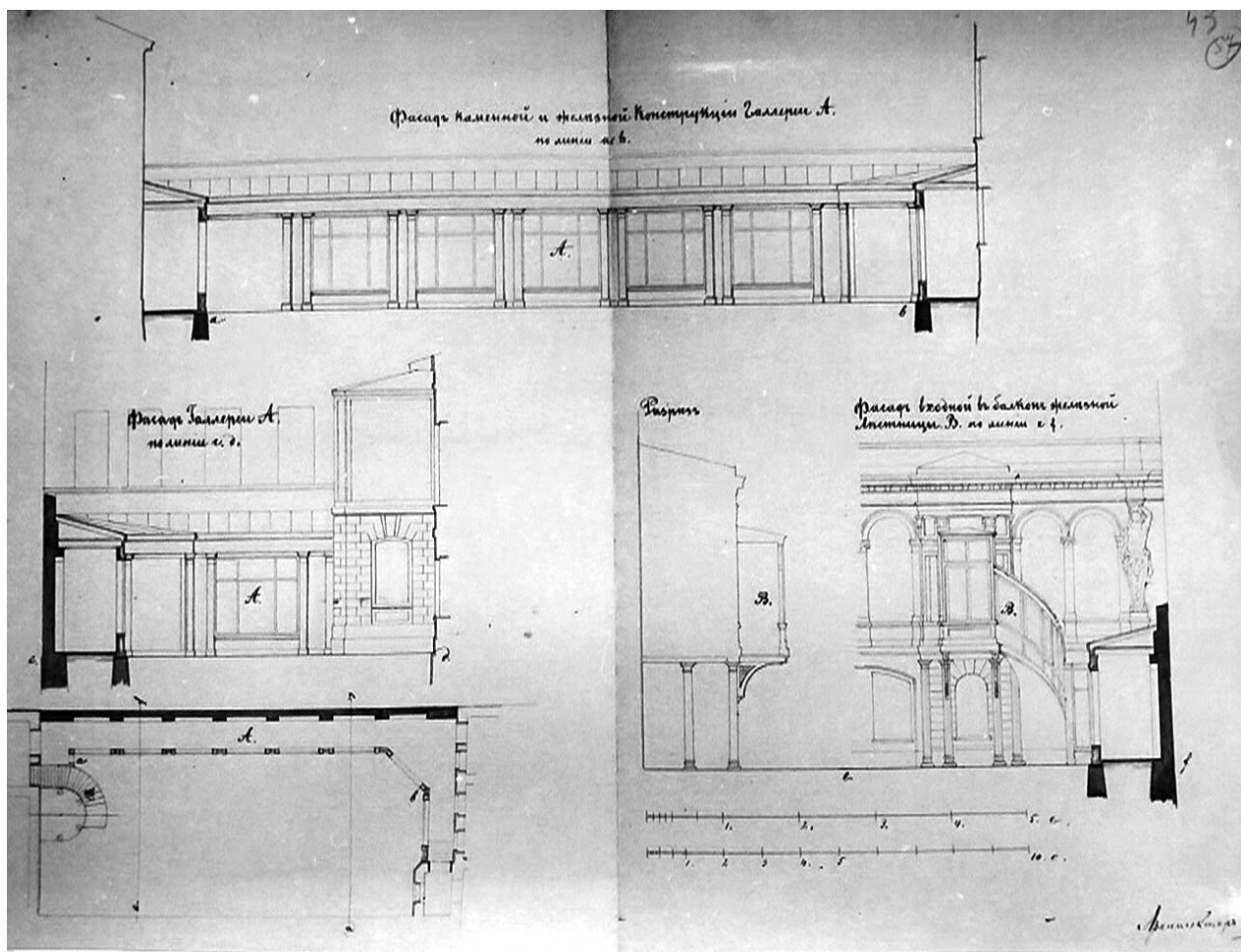
33. Дом В. И. Мятлева. Северный двор. Фасад каменной конструкции галереи А по линии а-в. Фасад галереи А по линии с-д. Фасад входной в балкон железной лестницы В по линии с-ф. Архитектор И. И. Цим. ЦГИА СПб, ф. 513, оп. 102, д. 3388, л. 57.
