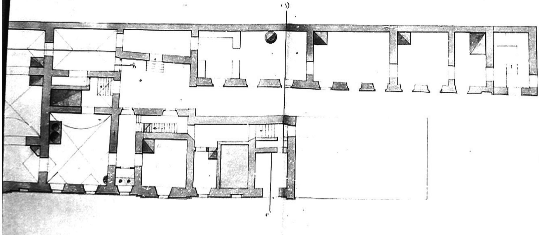
62. Дом Санкт-Петербургского I гильдии купца А. К. Кумберга. План подвального этажа. Июнь 1876 года. Архитектор Э. Г. Юргенс. ЦГИА СПб, ф. 515, оп. 4, д. 3525, л. 9, 10.
