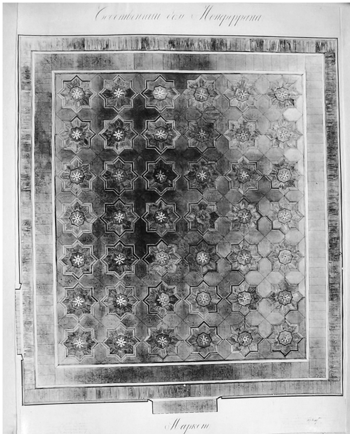
123. Наб. реки Мойки, 86-88. 2 этаж. Паркет в гостиной (рядом с эркером). Обмерный чертеж. КГИОП СПб, нег. 35436.
