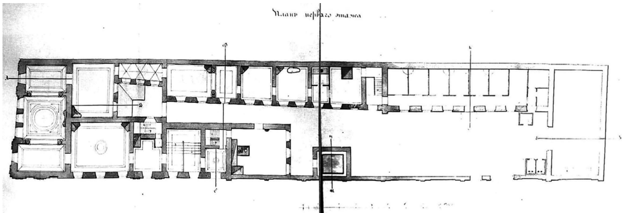
60. Дом Санкт-Петербургского I гильдии купца А. К. Кумберга. План I этажа. Июнь 1876 года. Архитектор Э. Г. Юргенс. ЦГИА СПб, ф. 515, оп. 4, д. 3525, л. 5, 6, 7, 8.
