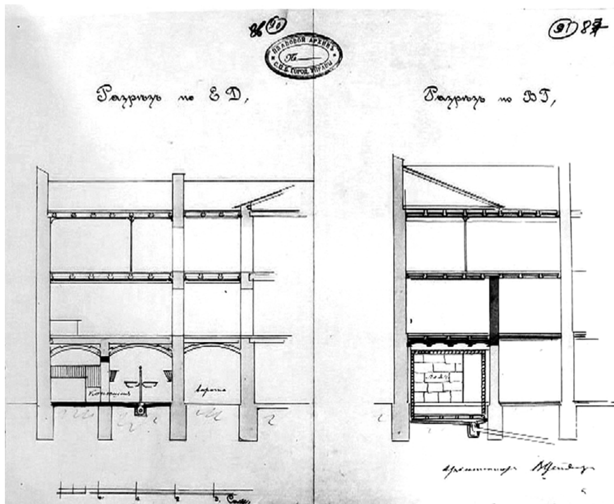
54. Дом Я. В. Ратькова-Рожнова. Разрез ледника и конюшни. Проект. 1910 г. Архитектор В. П. Цейдлер. ЦГИА СПб, ф. 513, оп. 102, д. 3388, л. 86, 87.
