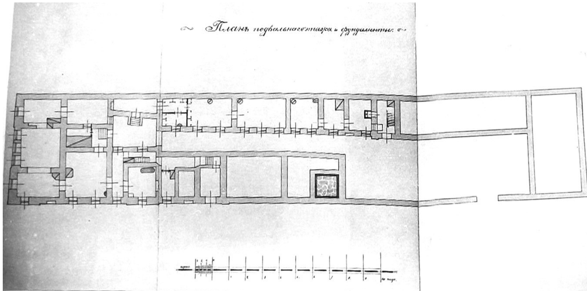
73. Дом А. Е. Бодиско. План подвального этажа и фундамента. 1913 г. ЦГИА СПб, ф. 515, оп. 4, д. 3525, л. 24, 25, 26.
