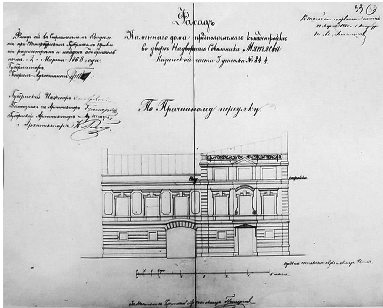
23. Фасад каменного дома, предполагаемого к надстройке во дворе надворного советника Мятлева, Казанской части 3 участка по набережной реки Мойки № 84, 4. По Прачешному переулку. Архитектор И. И. Цим. 1868 г. ЦГИА СПб, ф. 513, оп. 102, д. 3388, л. 32, 33.
