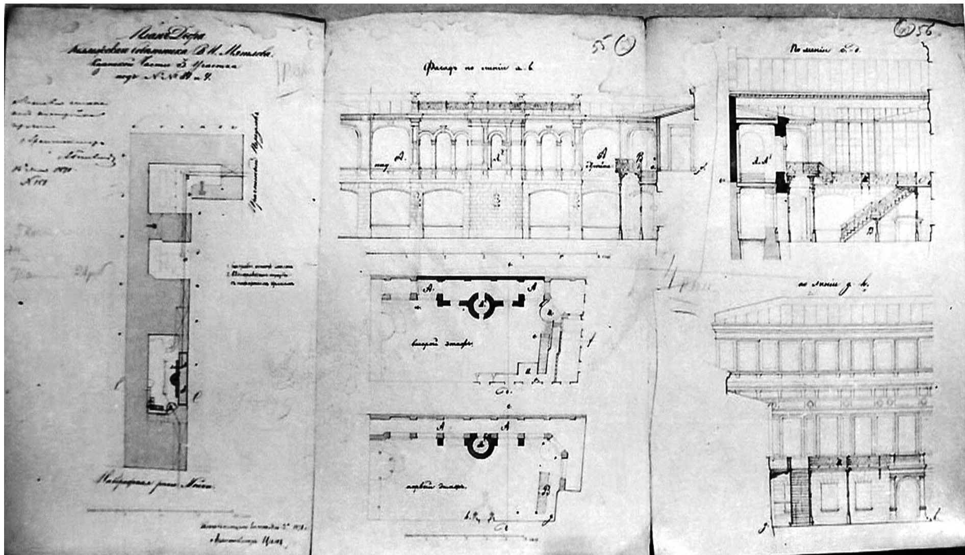
34. План двора коллежского советника В. И. Мятлева. Планы и фасады северного двора. 1871 г. Архитектор И. И. Цим. ЦГИА СПб, ф. 513, оп. 102, д. 3388, л. 59 - 61.
