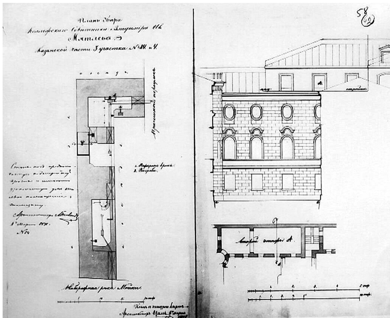
37. План двора коллежского советника Владимира Ивановича Мятлева. Казанской части 3-го участка № 84 и 4. «План с натурой верен. Архитектор И. И. Цим. 6 марта 1871 г.». ЦГИА СПб, ф. 513, оп. 102, д. 3388, л. 57, 58.
