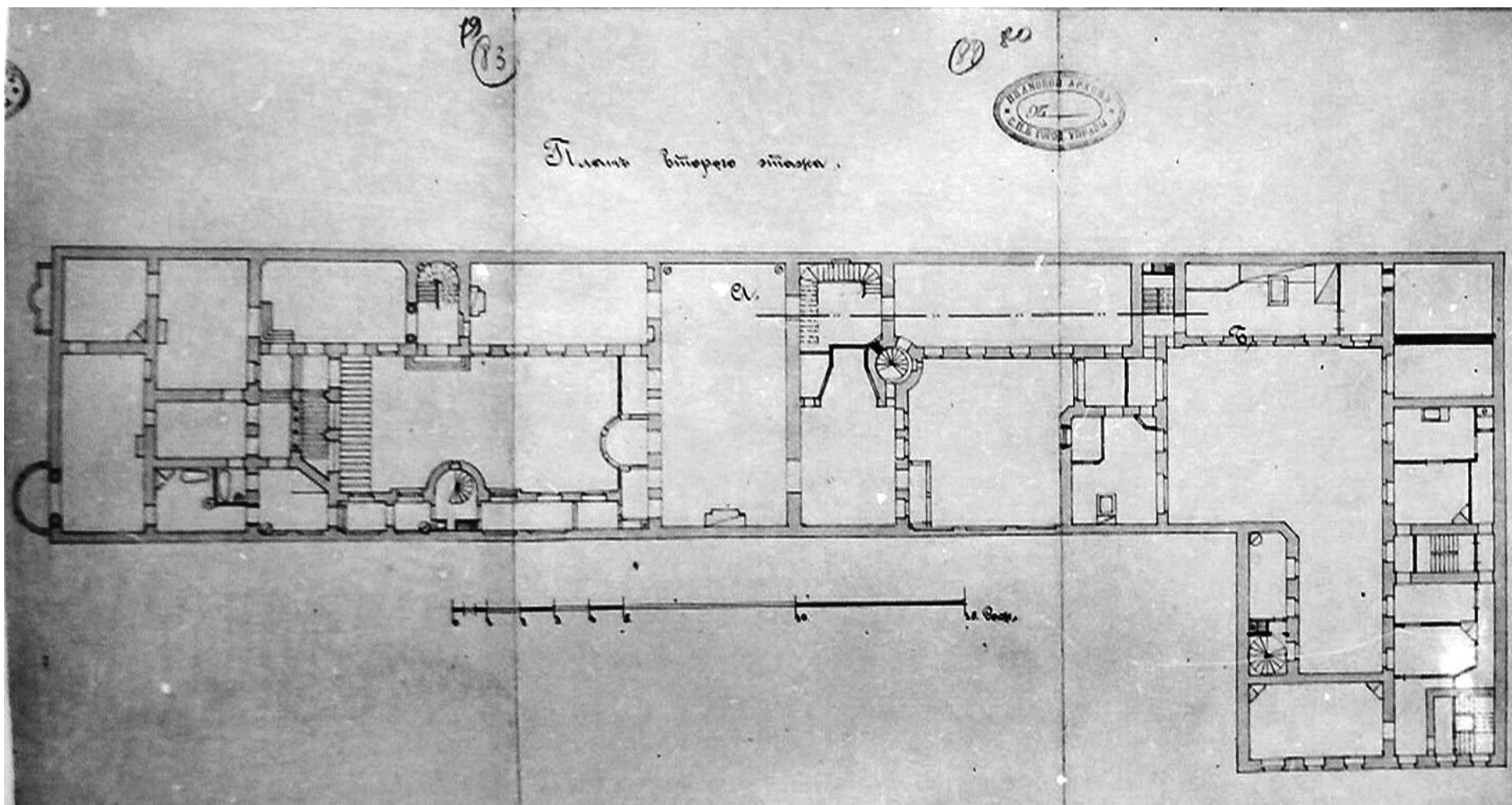
51. Дом Я. В. Ратькова-Рожнова. План второго этажа. 1910 г. Архитектор В. П. Цейдлер ЦГИА СПб, ф. 513, оп. 102, д. 3388, л. 79, 80, 81.
