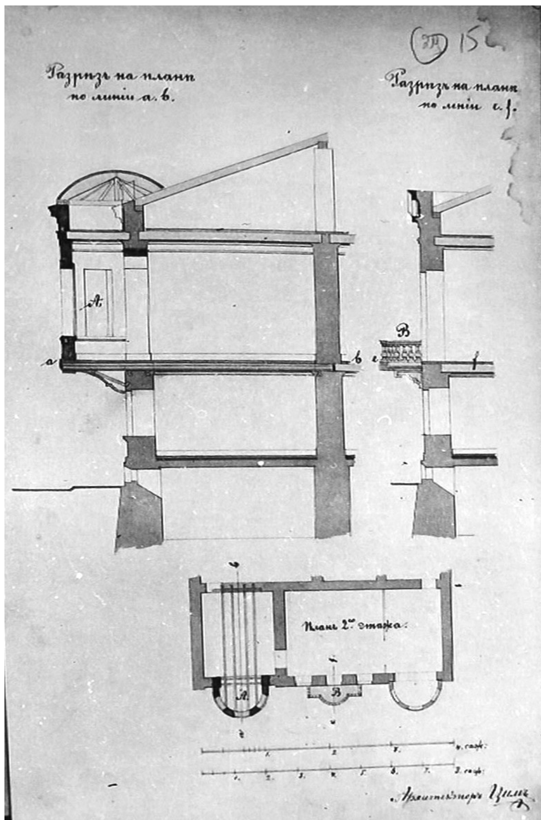
27. Дом В. И. Мятлева. Разрез и план северной части северного корпуса, выходящего на набережную реки Мойки. Проект устройства эркера лит. А и балкона лит. В. Архитектор И. И. Цим. 1868 г. ЦГИА СПб, ф. 513, оп. 102, д. 3388, л. 29.
