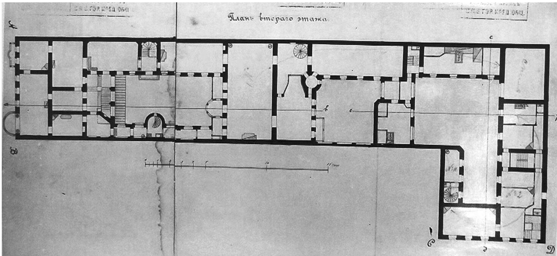
46. Дом графини Л. П. Бутурлиной. План II этажа. 1904 г. ЦГИА СПб, ф. 515, оп. 4, д. 3524, л. 10 - 12.
