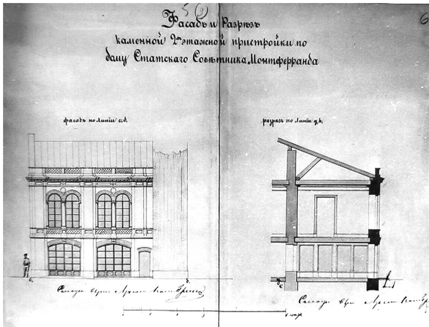
19. Фасад и разрез каменной двухэтажной пристройки по дому статского советника Монтерранда. Проект. «С натурою верно. Архитектор О. Пуаро». ЦГИА СПб, ф. 513, оп. 102, д. 3388, л. 5, 6.
