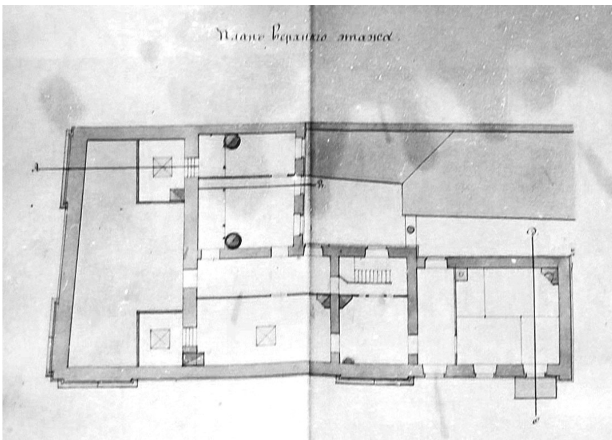
61. Дом Санкт-Петербургского I гильдии купца А. К. Кумберга. Планверхнего (II) этажа. Июнь 1876 года. Архитектор Э. Г. Юргенс. ЦГИА СПб, ф. 515, оп. 4, д. 3525, л. 11, 12.
