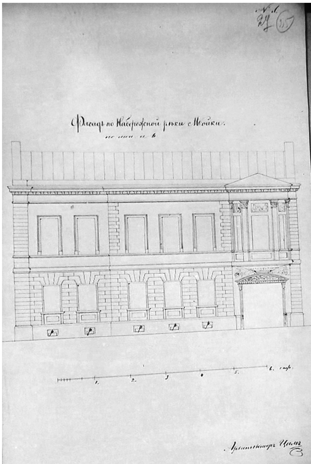
25. Фасад по набережной реки Мойки. Архитектор И. И. Цим. 1868 г. ЦГИА СПб, ф. 513, оп. 102, д. 3388, л. 25.
