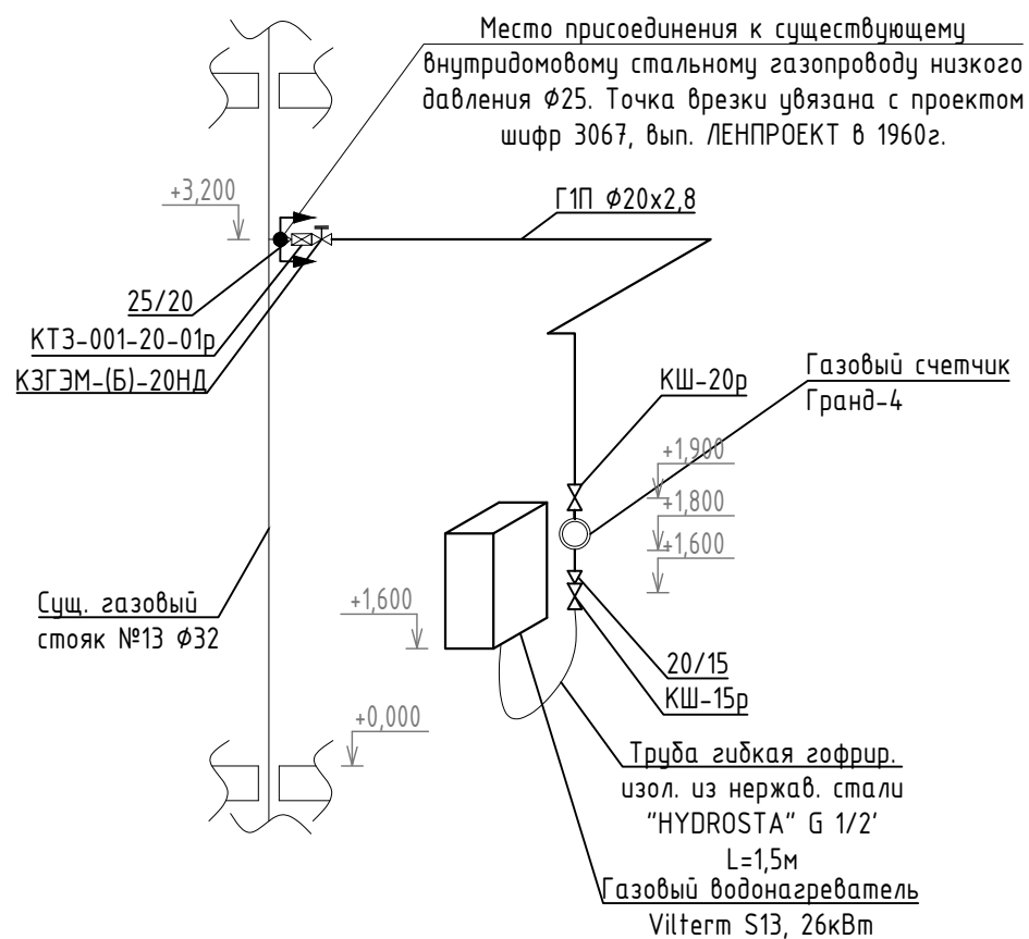
АксонOMETрическая схема газопровода в помещении кухни. Проектируемый газопровод.
