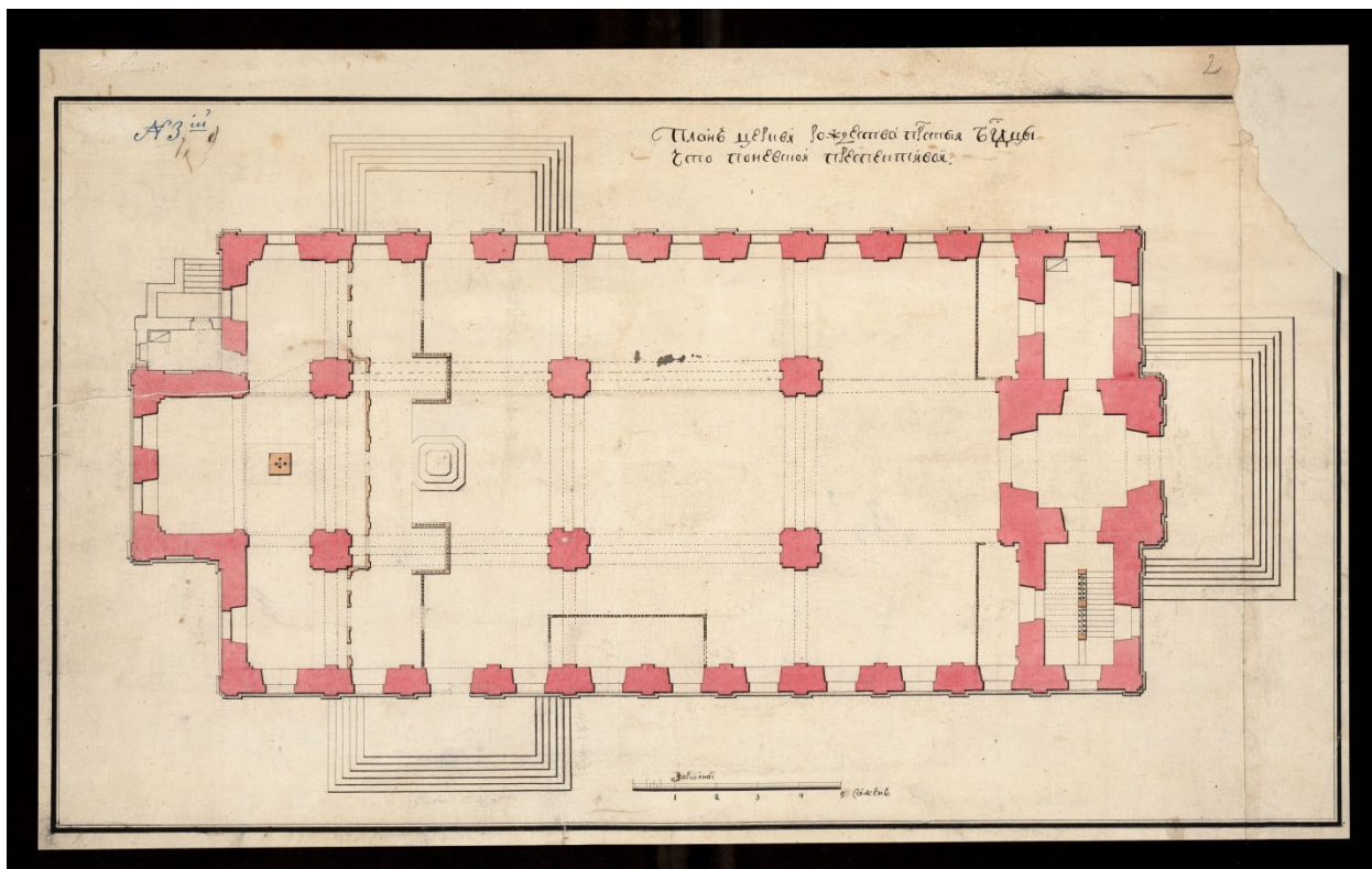
Ил. 7. Фиксационный план церкви Рождества Богородицы, середина XVIII в. Источник: РГИА. Ф. 485. Оп. 2. Д. 669. Л. 2
