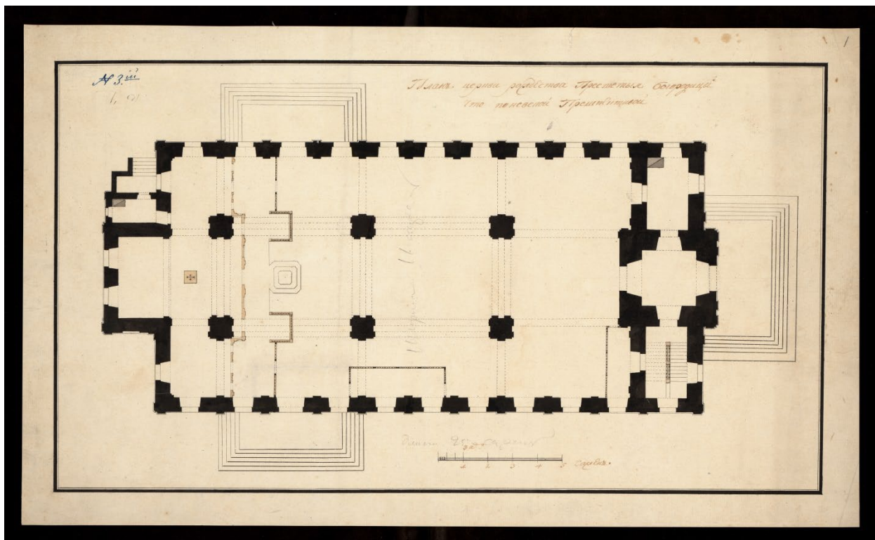
Ил. 6. Фиксационный план церкви Рождества Богородицы, середина XVIII в. Источник: РГИА. Ф. 485. Оп. 2. Д. 669. Л. 1
