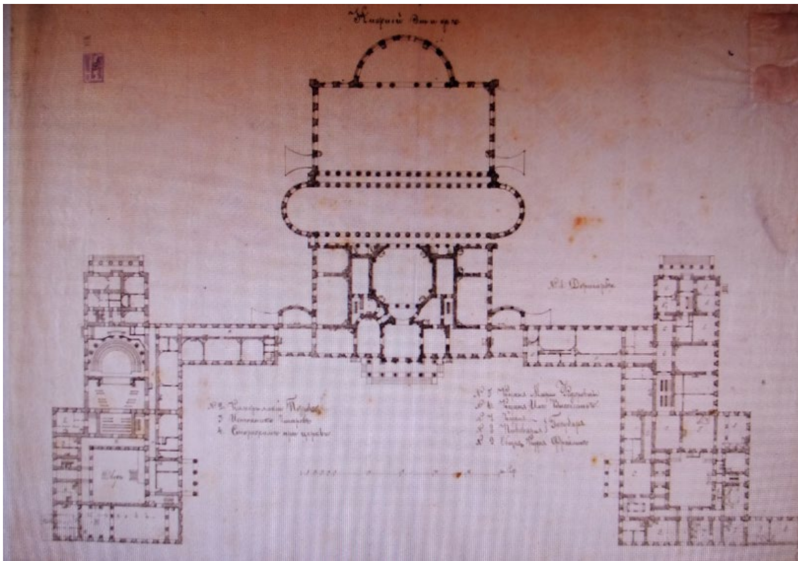
12. План 1-го этажа Таврическаго дворца. 1911 // НИМ РАХ А15019№ 20176
