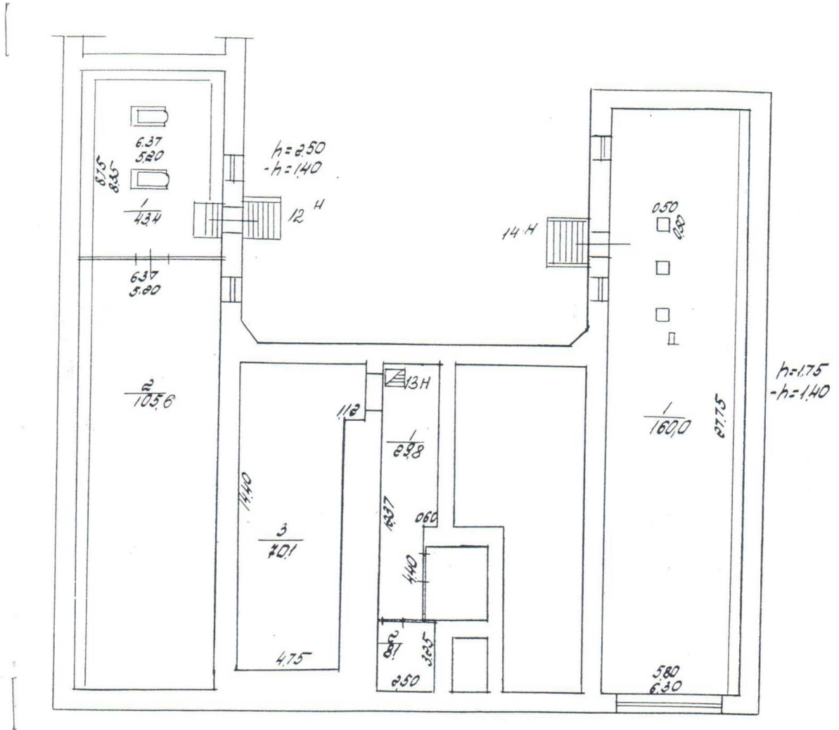
План подвала.
