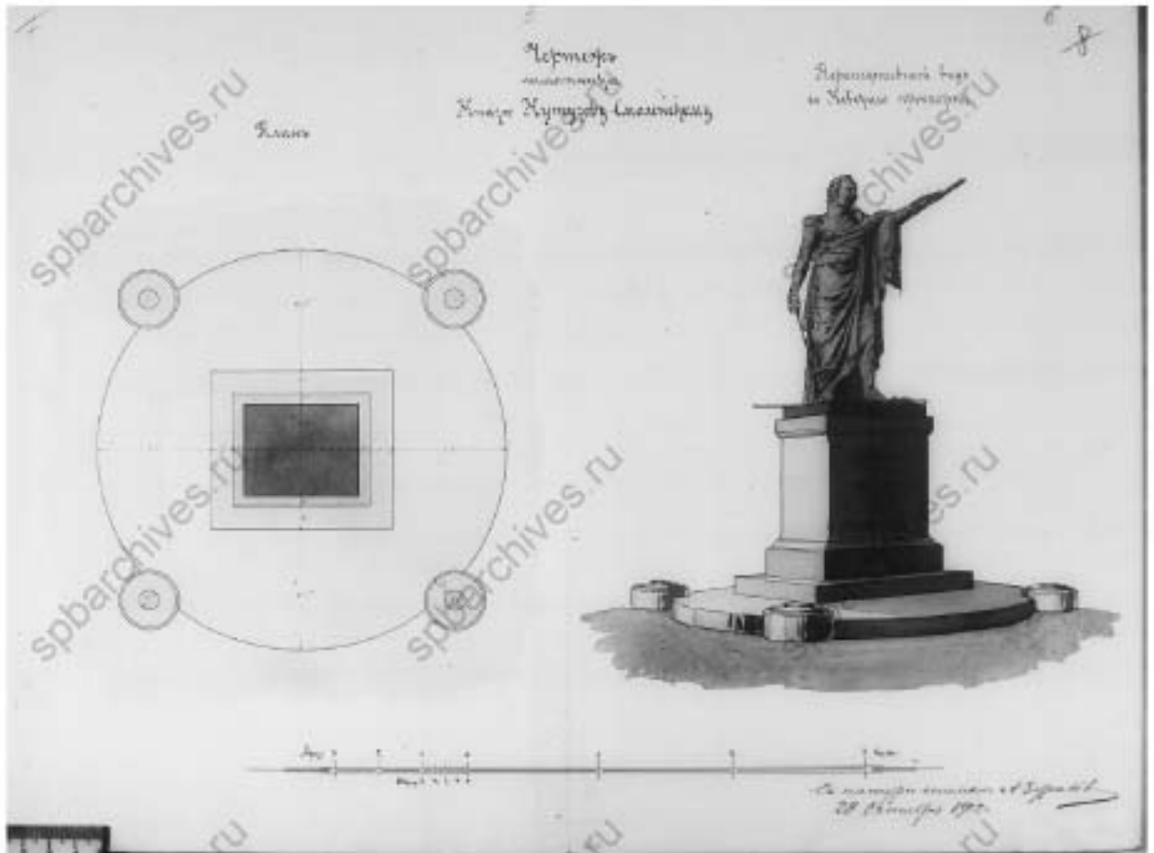
36. ЦГИА СПб. Фонд 513. Опись 101. Дело 301 Чертежи памятника фельдмаршалу М.И.Кутузову
