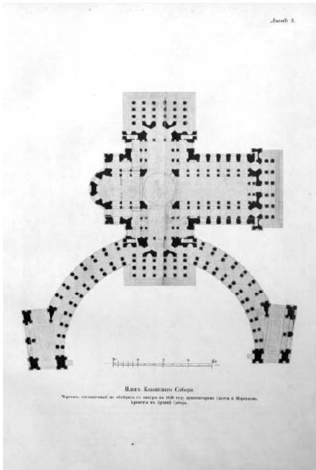
13. План Собора. Аплаксинъ А. 1911 "Казанскій соборъ" Аплаксин А. Казанскій собор: Историческое исследование о соборе и его описаніе. [Спб.], 1911.
