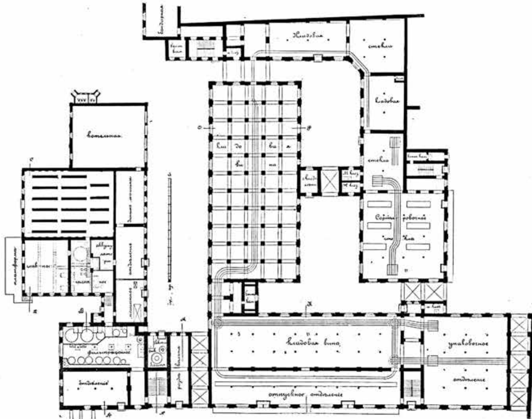
Чер. 198. Планъ 1-го этажа.
