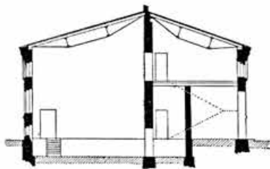
Чер. 216. Разрѣзъ угольнаго завода.
