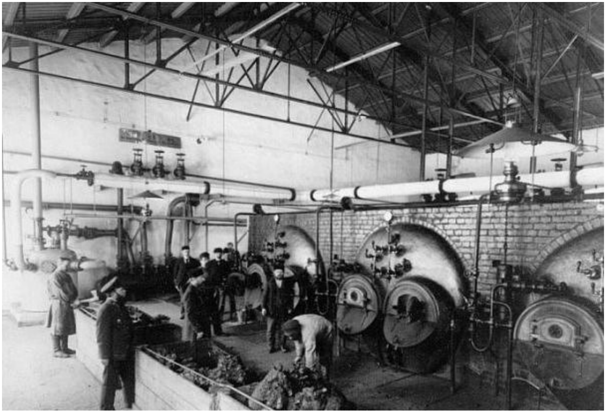
Илл. 14. Котельная Четвертого казенного винного склада. 1900-е гг. ЦГА КФФД. Е 14495.
