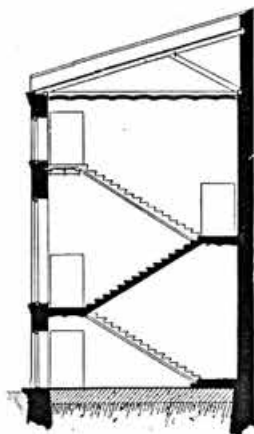
Чер. 212. Разрѣзъ лѣстницы склада ящиковъ.
