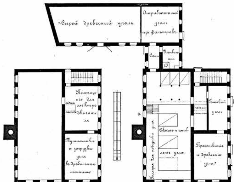
Чер. 214. Планъ 2-го этажа угольного завода.
