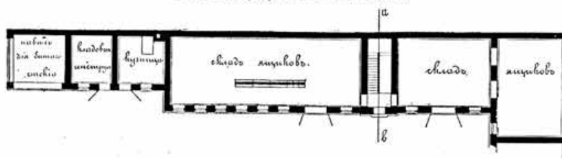
Чер. 211. Планъ 1, 2, 3 и 4-го этажей склада ящиковъ.
