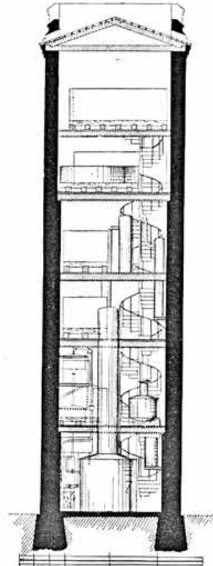
Чер. 210. Разрѣзъ ректификаціонной башни.
