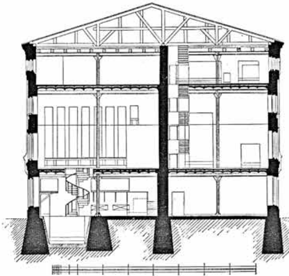
Чер. 209. Разрѣзъ фильтраціоннаго отдѣленія.
