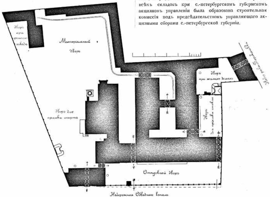
Чер. 193. Генеральный планъ.
