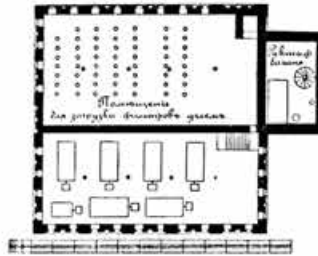
Чер. 205. Планъ 4-го этажа, фильтраціоннаго отд.
