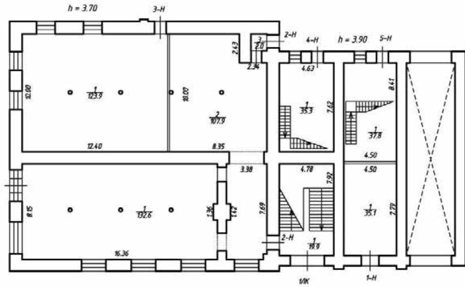
План 1 этажа
