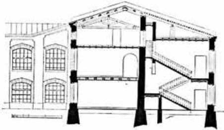
Чер. 208. Разрѣзъ по МН.
