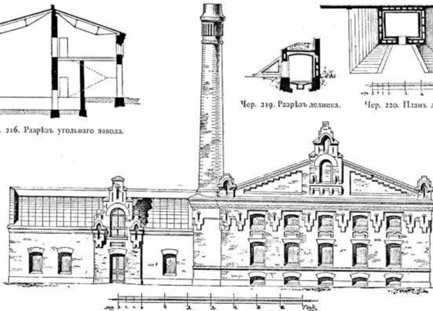
Чер. 217. Фасадъ угольнаго завода.
