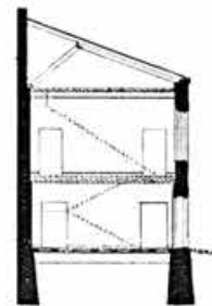
Чер. 201. Разрѣзъ столовой.
