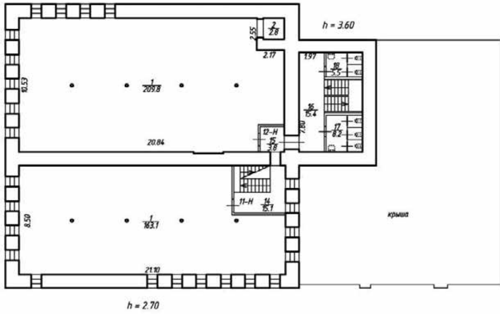
План 4 этажа
