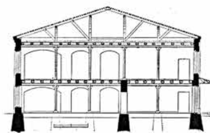
Чер. 213. Поперечный разрѣзъ розливного отдѣленія.
