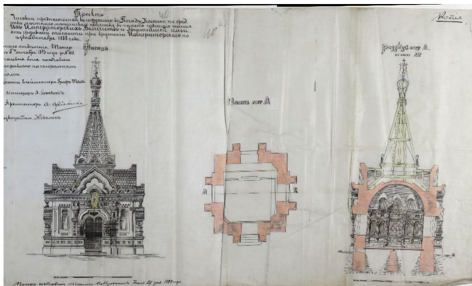
Илл.1. Фрагменты план границ территории объекта культурного наследия регионального значения Часовня во имя св. блгв. кн. Александра Невского Богадельни Колпинского Мещанского общества. 16 сентября 1893 г.
