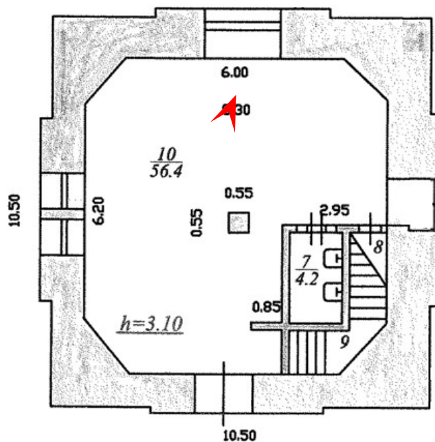
11. Объект культурного наследия регионального значения «Часовня св. Александра Невского» по адресу: Санкт-Петербург, г. Колпино, ул. Адмиралтейская, д.6, литер А (Санкт-Петербург, г. Колпино, улица Володарского, дом 6, литера А) Первый этаж Дата съемки: 11 марта 2024 года
