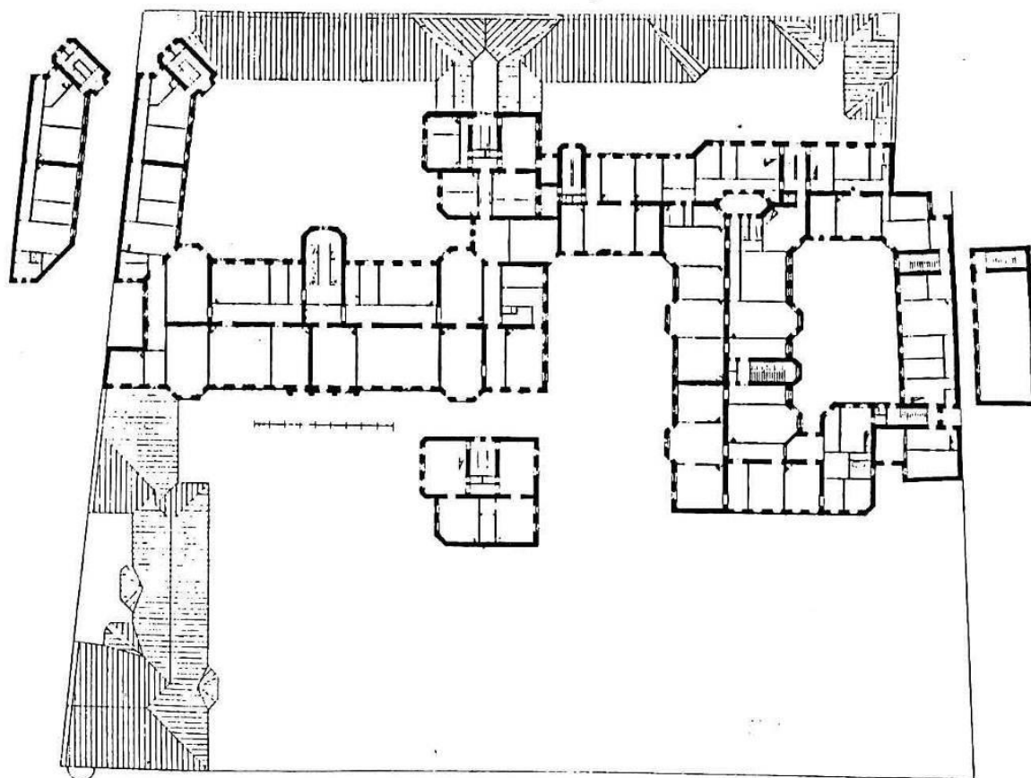
Чер. 428. Домъ страхов. об-ва «Россия». Планъ 4-го этажа.
