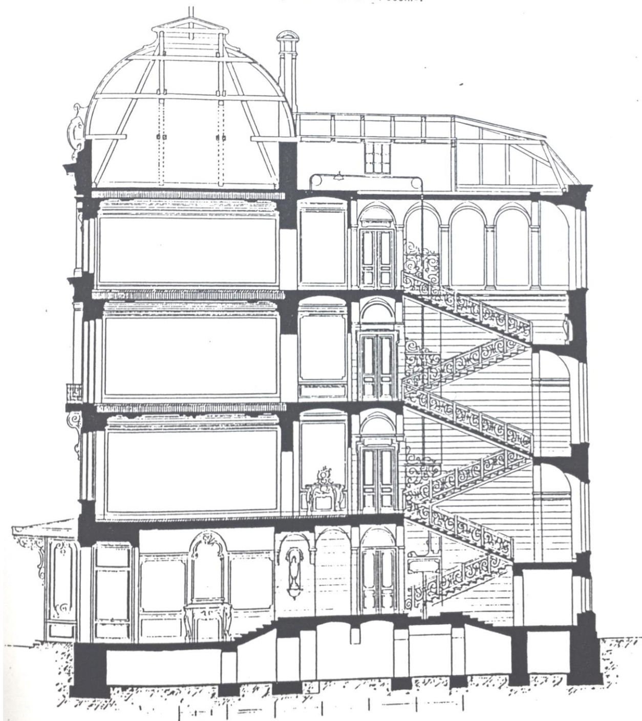
Чер. 432. Разрѣзъ по № 1 му.
