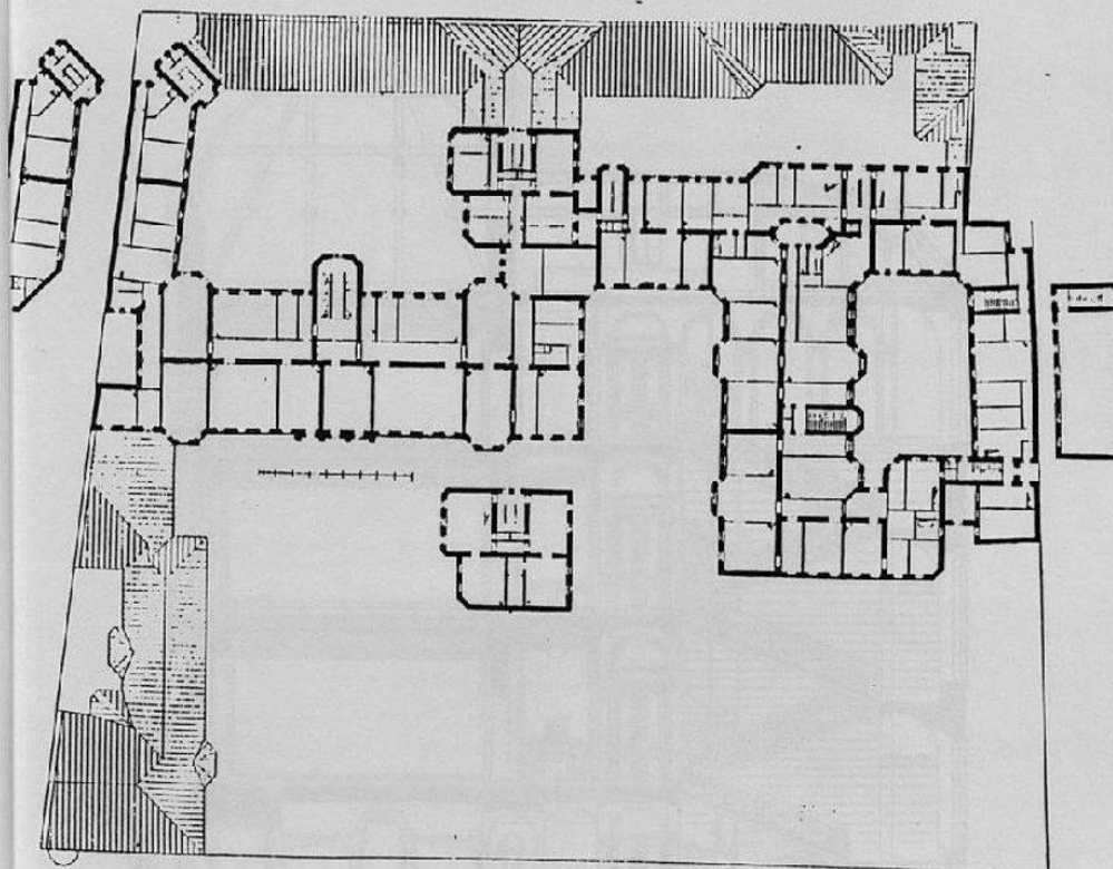
Чер. 428. Домъ страхов. об-ща «Россия». Планъ 4-го этажа.
