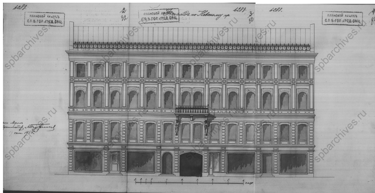
13. Фасад по Невскому проспекту. 1909 г. ЦГИА СПб. Ф.515. Оп.4. Д. 3908. Лл. 32-34.
