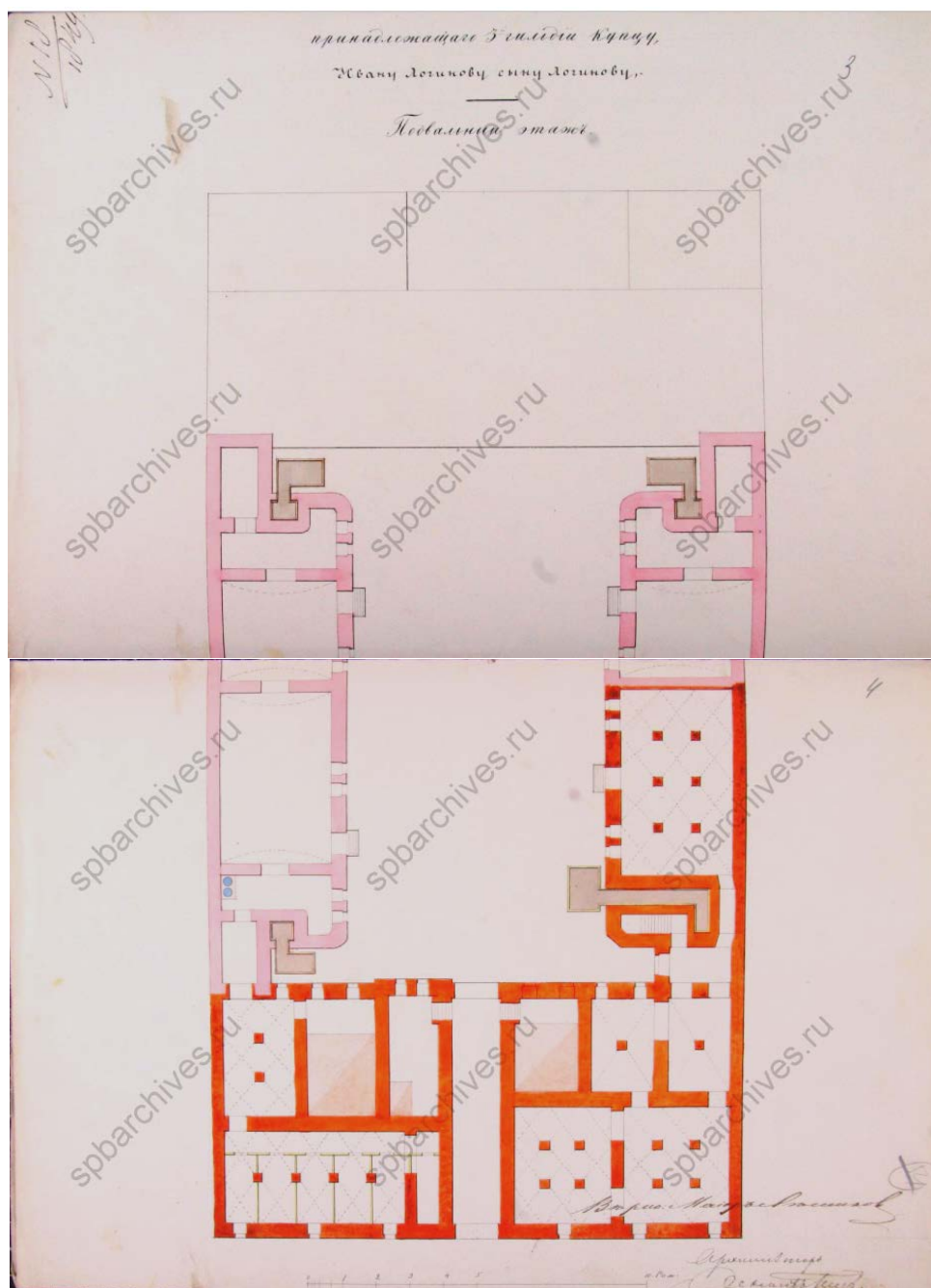
3. План подвального этажа. 1849 г. Арх. А.Х.Пель. ЦГИА СПб. Ф.513. Оп. 102. Д. 5020. Лл. 3-4.
