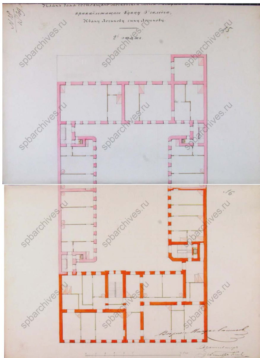
5. План второго этажа. 1849 г. Арх. А.Х.Пель. ЦГИА СПб. Ф.513. Оп. 102. Д. 5020. Лл. 15-16.
