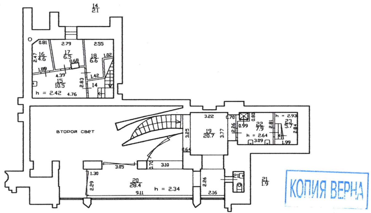
План антресоли
