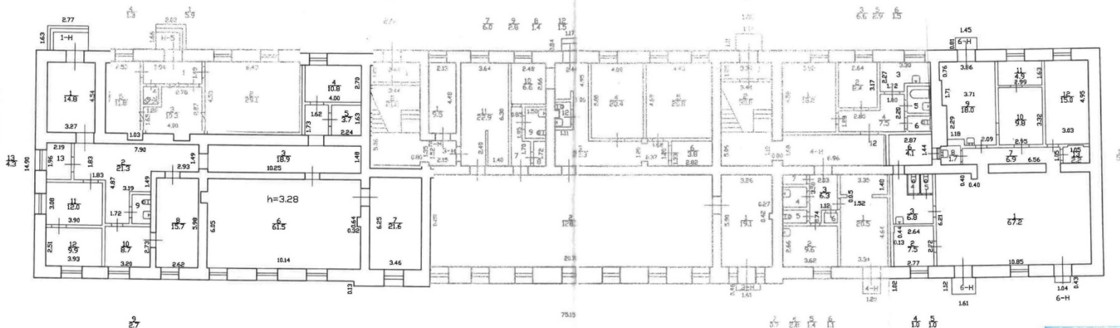
План 1 этажа
