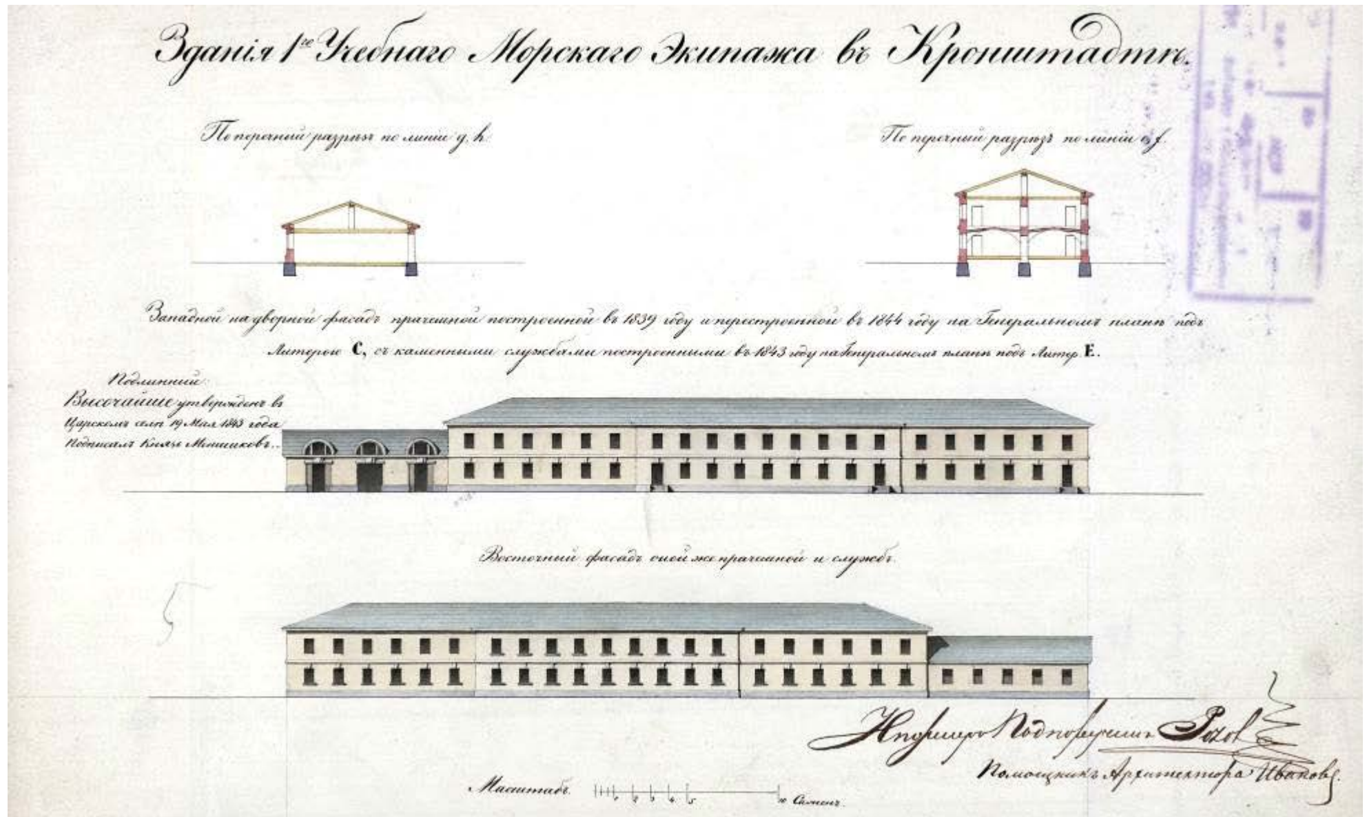
Илл. 9. «Чертеж здания прахешной при казарме 1-го Учебного морского экипажа – западный и восточный фасады и профили». Инженер-подпоручик [Н.Я.] Розов, помощник архитектора Иванов. 1843–1844 гг. – РГА ВМФ. Ф. 326. Оп. 1. Д. 6936.
