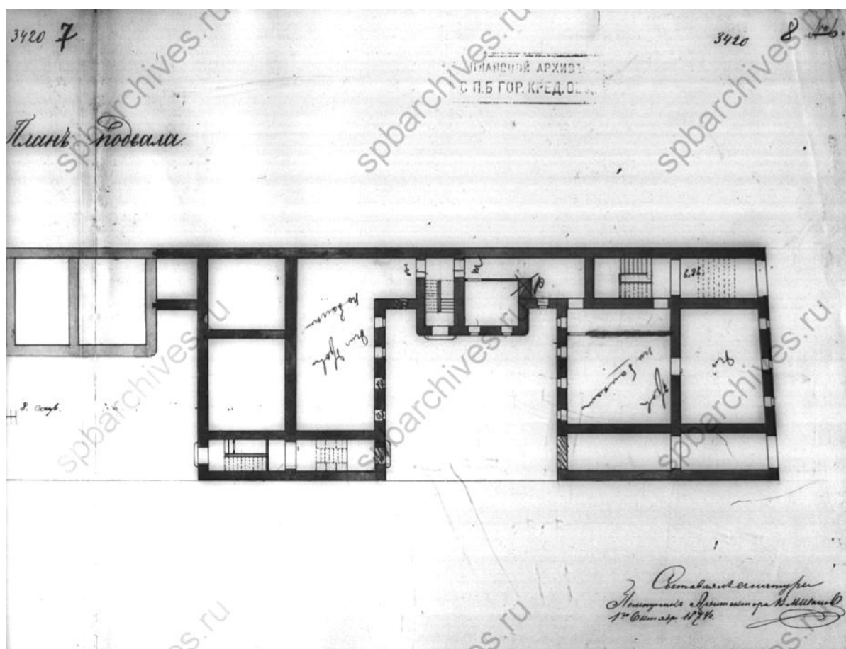
Илл.23. План подвала. 1874 г. (Фрагмент) ЦГИА СПб. Ф. 515. Оп. 4. Д. 11. Л. 7-8.
