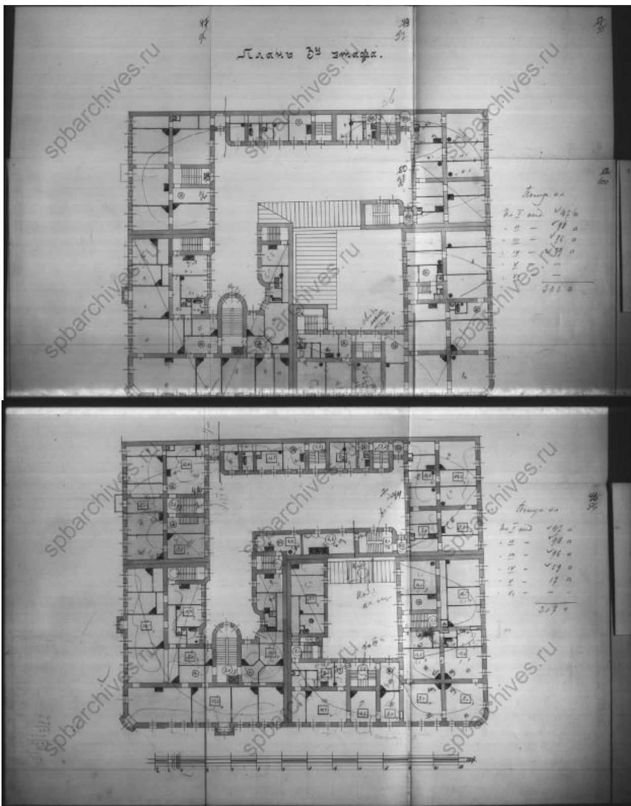
19. План 3-го этажа дома А.Е. Бурцева 1906. // ЦГИА СПб Ф. 515, Оп. 4, Д. 3726А. Л.47-54
