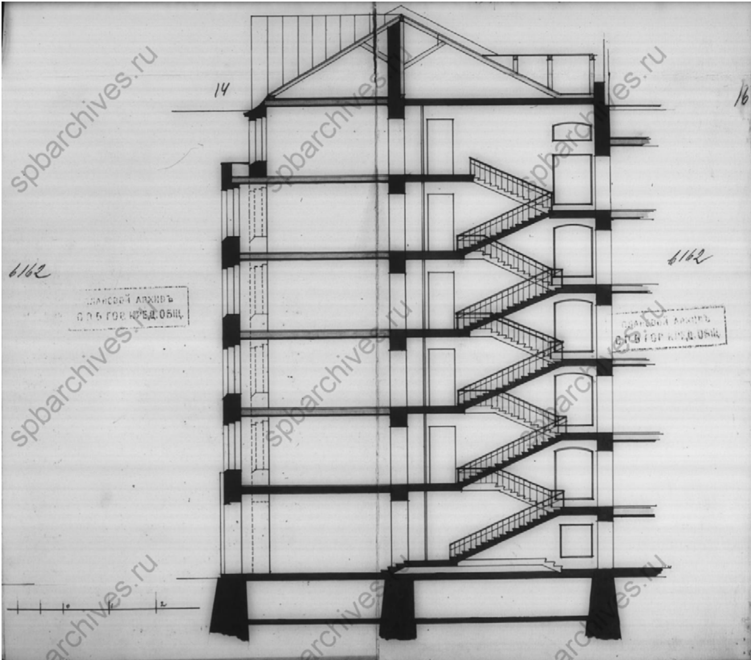
24. Разрез по СД. Б/д. // Источник: ЦГИА СПб Ф.515 Оп.4 Д.2333 Л.13-16.
