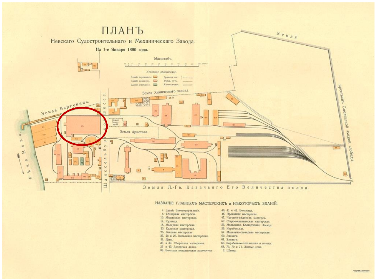
7. План Невскаго судостроительнаго и механическаго завода. 1890 г. // Невскій судостроительный и механический завод. К выпуску 3000 паровоза с основанія завода. СПб., 1910.
