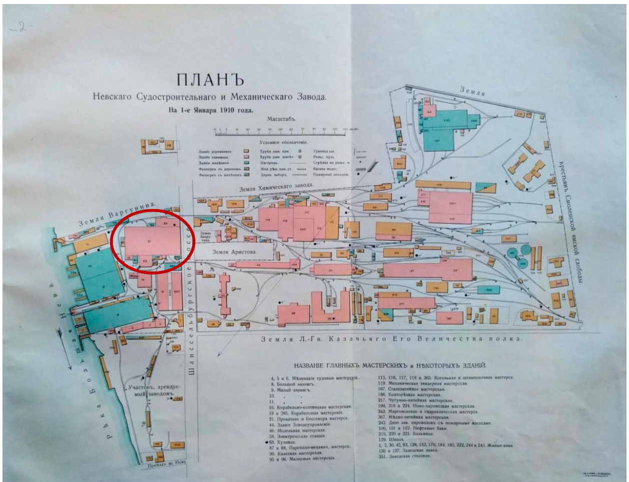
8. План Невскаго судостроительнаго и механическаго завода. 1910 г. // Невскій судостроительный и механический завод. К выпуску 3000 паровоза с основанія завода. СПб., 1910.
