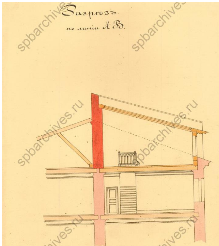
Илл. 15. Разрез по линии АВ. Дата: 1882 г. Автор: гражд. инж. Д. Прусак. Источник: ЦГИА СПб, ф. 513, оп. 102, д. 138.
