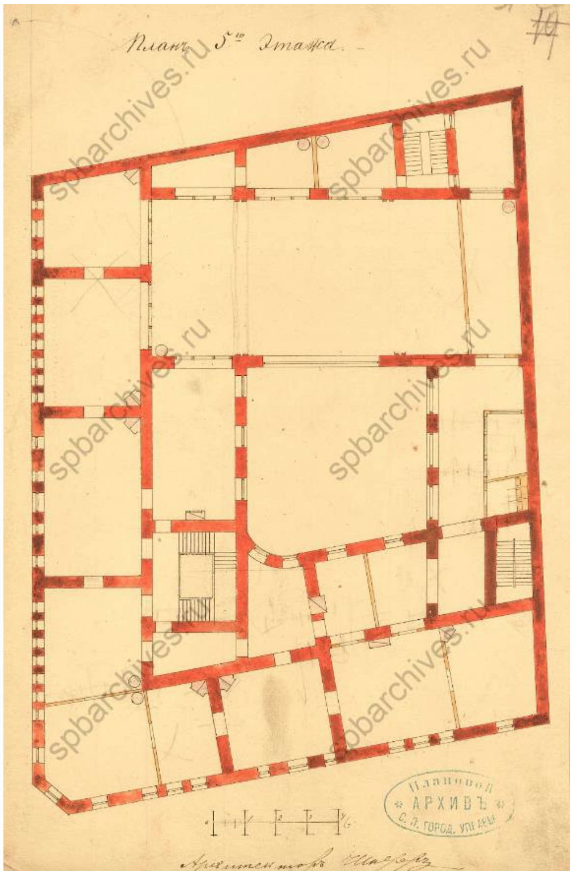
Илл. 9. План 5-го этажа. Автор: арх. Шперер. Дата: 1880 г. Источник: ЦГИА СПб, ф. 513, оп. 102, д. 138.
