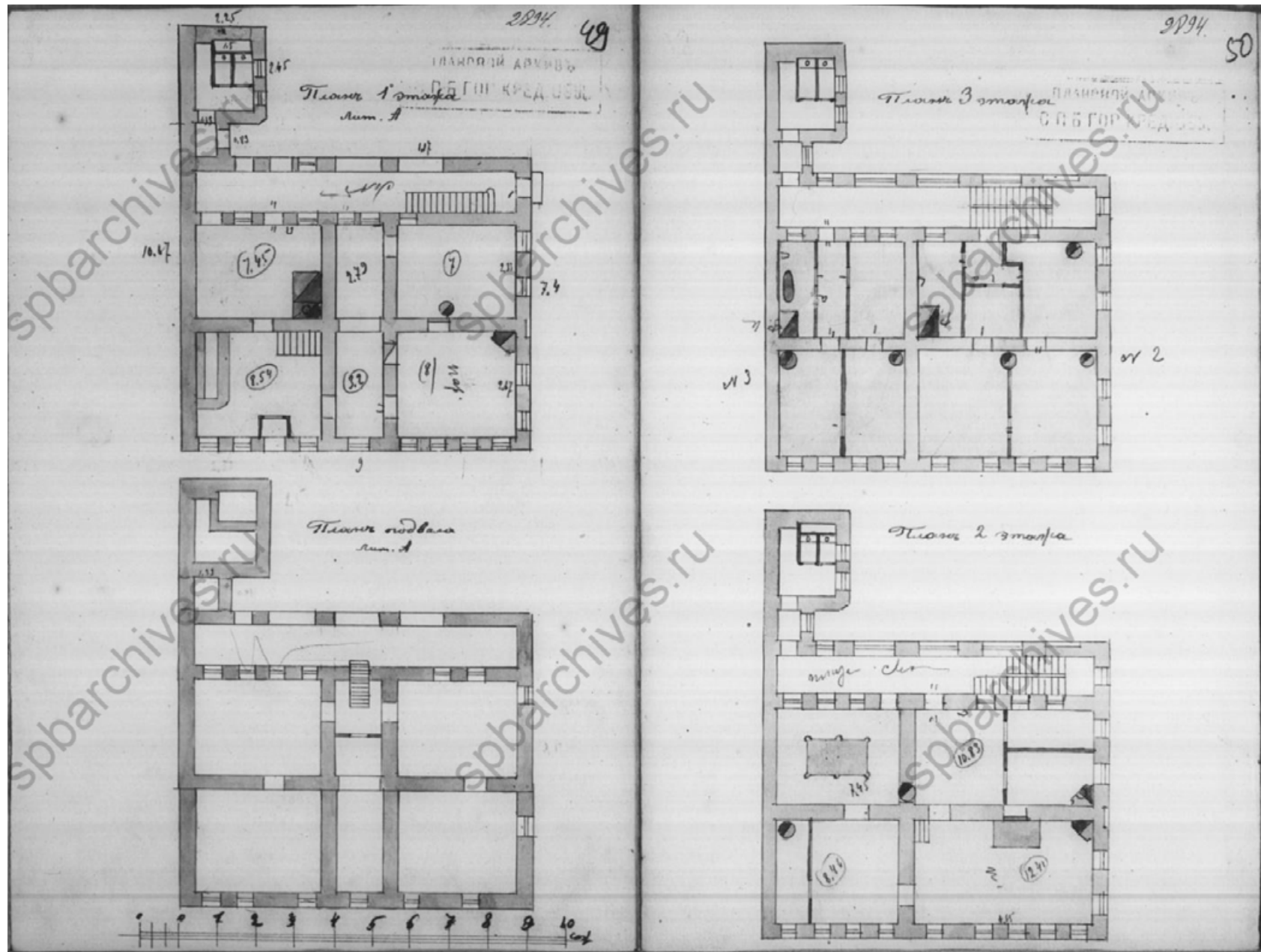
45. Планы подвала, 1-го, 2-го и 3-го этажей. Б/д. // Источник: ЦГИА СПб. Ф.515 Оп.4 Д.2563 Л.49-50.
