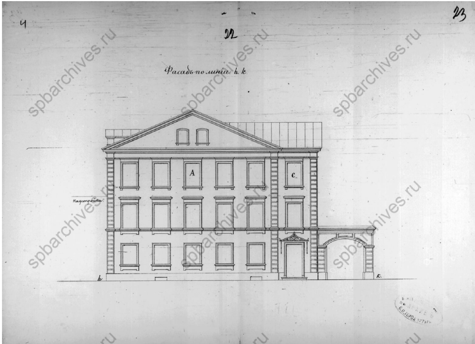
20. Фасад по линии бк. Б/д.// Источник: ЦГИА СПб. Ф. 513. Оп. 102. Д. 564. Л. 22-23.
