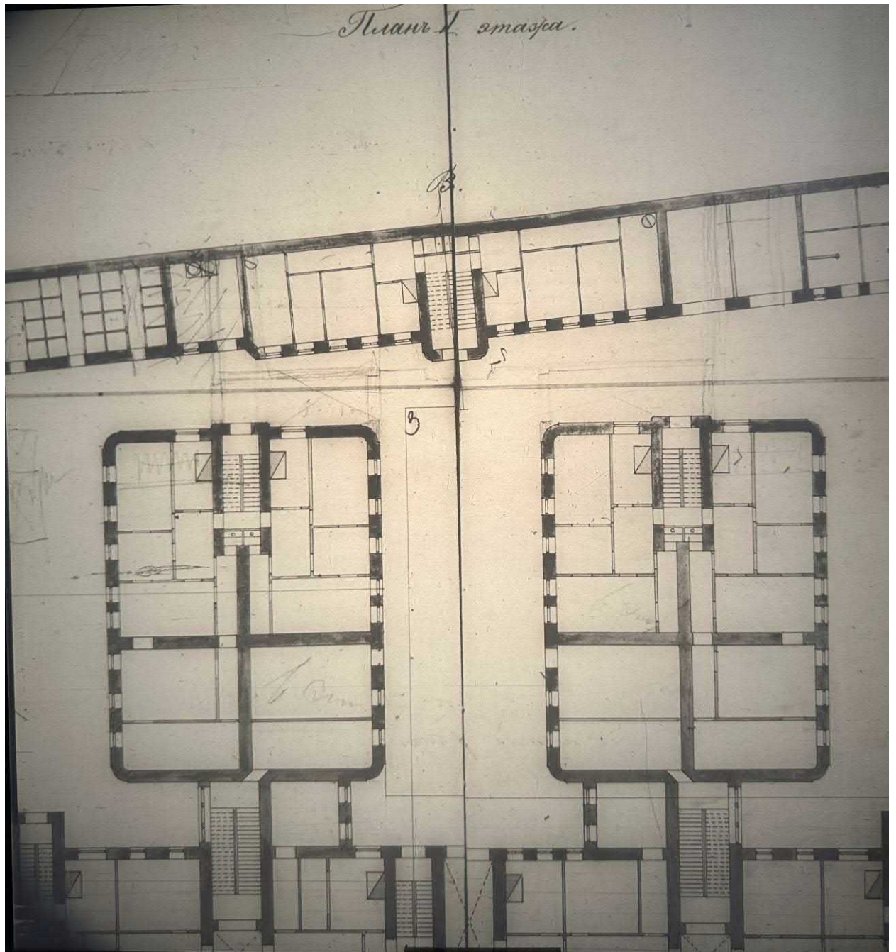
Илл.5. ЦГИА СПб. Фонд 513. Опись 102. Дело 5180. План 1 этажа
