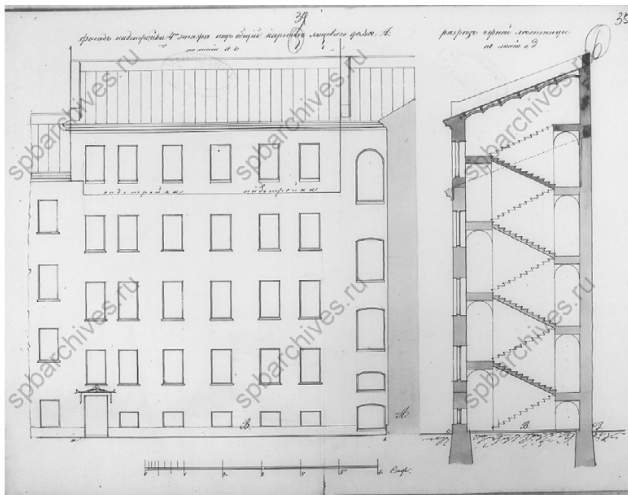
28. Фасад надстройки 4-го этажа по линии аб, и разрез черной лестницы по линии cd. Чертежи дома на участке, принадлежавшем Шварцу, В.И. Черепенникову, И.В. Черепенникову по наб.р. Фонтанки, 39. ЦГИА СПб. Фонд 513. Опись 102. Дело 9926. 1862 – 1902 гг. л. 34-35;
