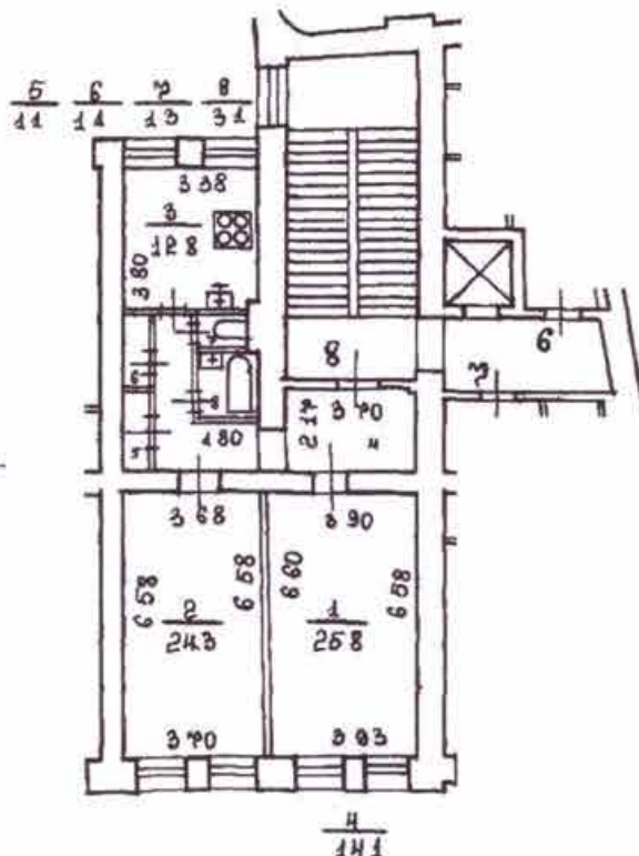
План 3-го этажа
