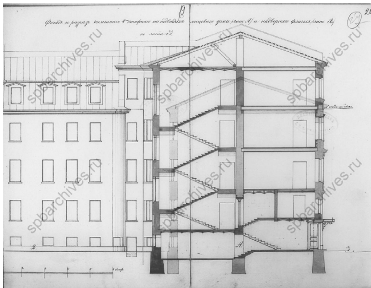
18. Фасад и разрез лестницы флигеля. Чертежи дома на участке, принадлежавшем Шварцу, В.И. Черепенникову, И.В. Черепенникову по наб.р.Фонтанки, 39. ЦГИА СПб. Фонд 513. Описание 102. Дело 9926. 1862 – 1902 гг. л. 19-20;
