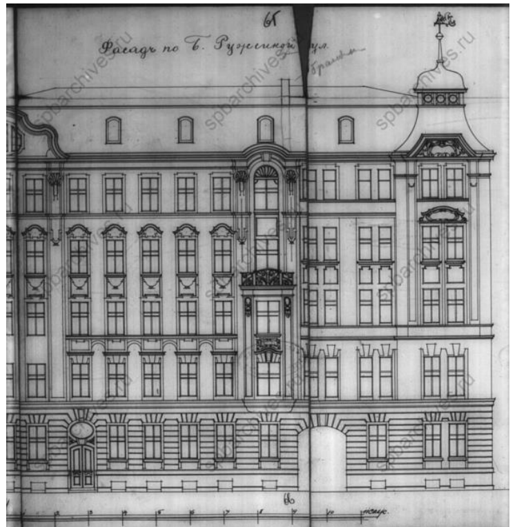
Илл. 30. «Фасад по Б. Ружейной ул.». 1902 г. // ЦГИА СПб. Фонд 513. Опись 102. Дело 7767
