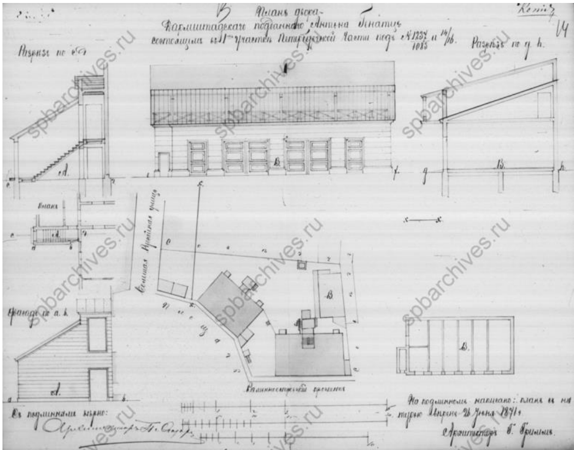
Илл. 9. «План двора Дармштадского подданного Антона Генатцъ состоящим в 1-м участке Петербургской Части под № 1237/1083 и 14/16». 1871 г. // ЦГИА СПб. Фонд 513. Описание 102. Дело 7767.
