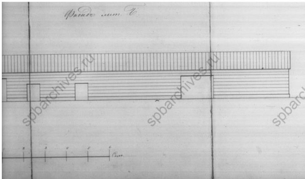
Илл. 17. «Фасад ли. Г». 1884 г. // ЦГИА СПб. Фонд 513. Опись 102. Дело 7767.
