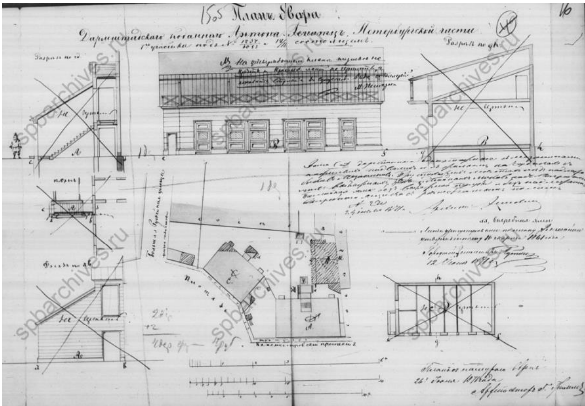
Илл. 9. «План двора Дармштадского подданного Антона Генатцъ состоящим в 1-м участке Петербургской Части под № 1237/1083 и 14/16». 1871 г. // ЦГИА СПб. Фонд 513. Описание 102. Дело 7767.
