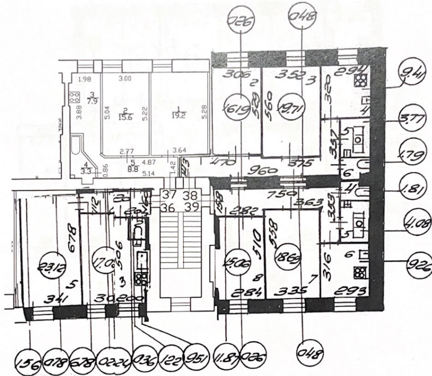
План 4 этажа h = 3.30
