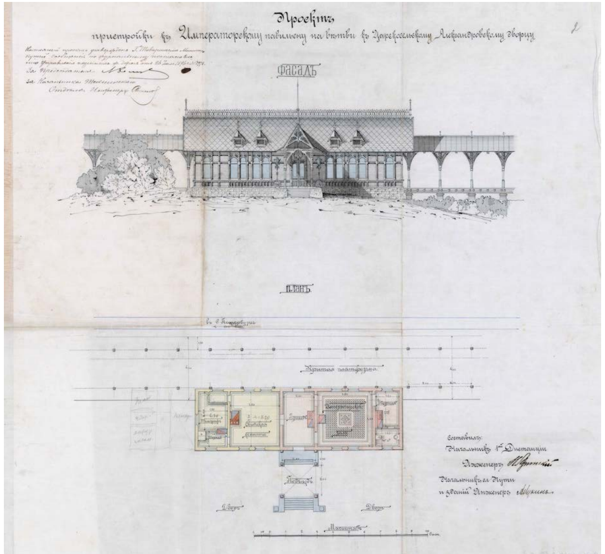
Илл 5. Проект пристройки к Императорскому павильону на ветви к Царскосельскому Александровскому дворцу. Фасад и план. 1896 г. РГИА. Ф 350. Оп. 44. Д. 774. Л. 2.
