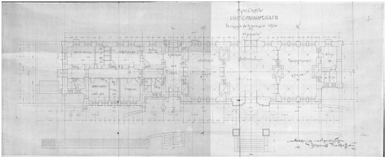
Илл. 14. Проект Императорского вокзала в Царском Селе. Архитектор В.А. Покровский. План. 1911 г. ЦГАНТД. Ф. 282. Оп. 1. Д. 124.
