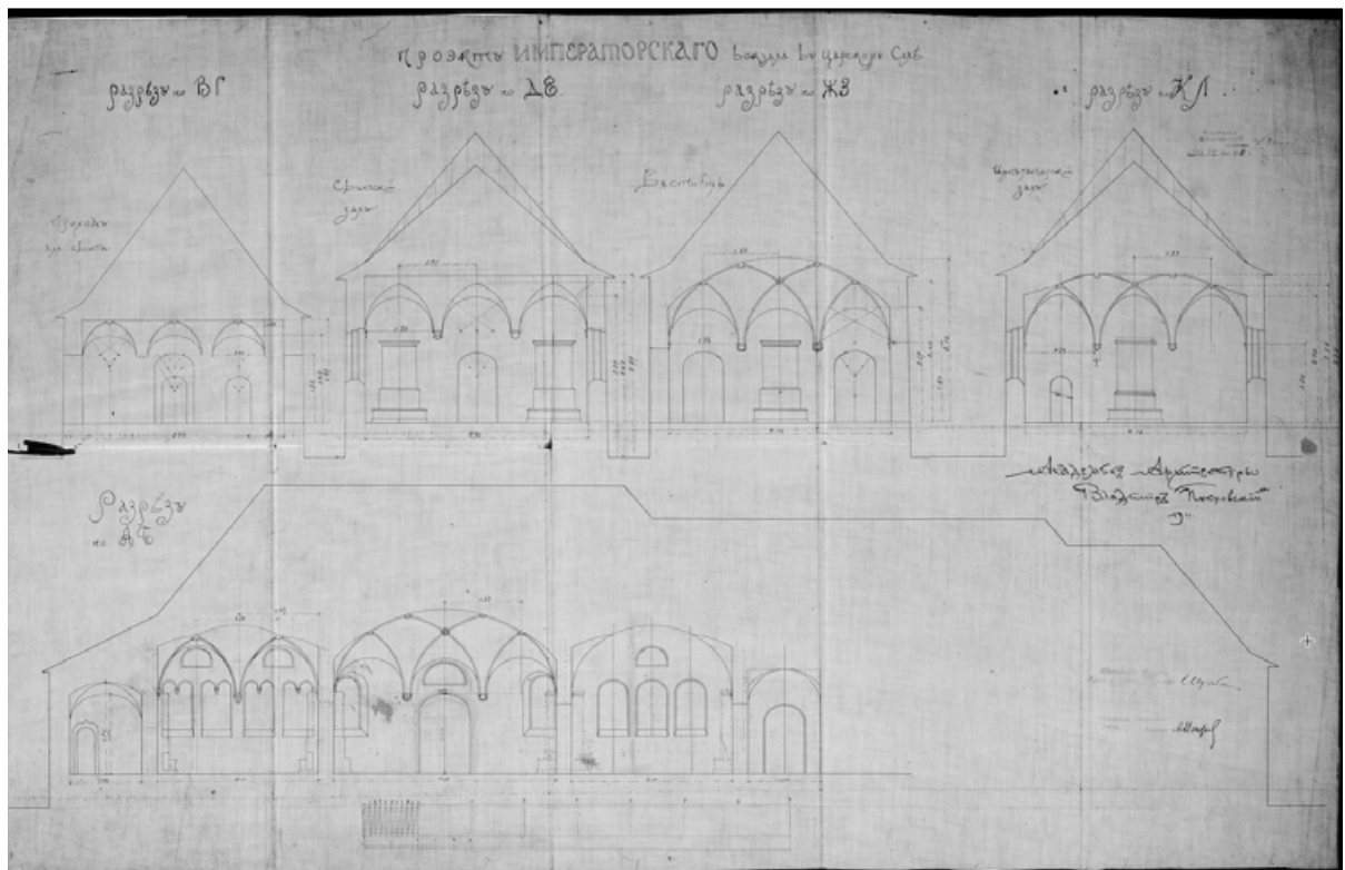
Илл. 13. Проект Императорского вокзала в Царском Селе. Архитектор В.А. Покровский. Разрезы. 1911 г. ЦГАНТД. Ф. 282. Оп. 1. Д. 124.
