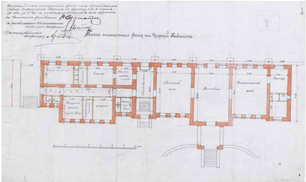
Илл. 17. План стационарного здания ст. Царский Павильон. 1911 г. РГИА. Ф 350. Оп. 44. Д. 775. Л. 2.
