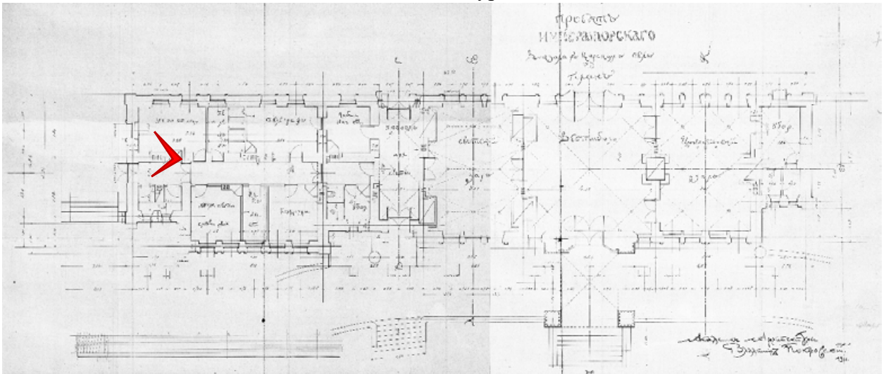
Фото 117. Помещение дежурного по станции.
