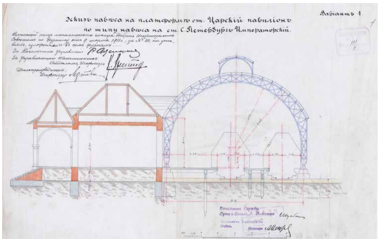
Илл. 18. Эскиз навеса на платформе ст. Царский павильон по типу навеса на ст. С.-Петербург-Императорский. Вариант 1. 1911 г. РГИА. Ф 350. Оп. 44. Д. 776. Л. 1.
