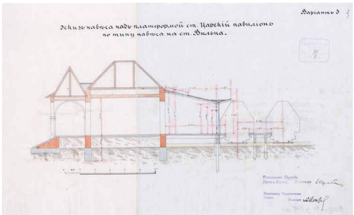
Илл. 20. Эскиз навеса над платформой ст. Царский павильон по типу навеса на ст. Вильна. Вариант 3. 1911 г. РГИА. Ф 350. Оп. 44. Д. 776. Л. 3.
