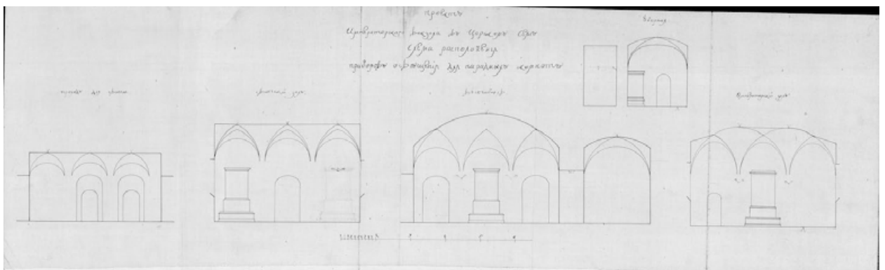
Илл. 15. Проект Императорского вокзала в Царском Селе. Архитектор В.А. Покровский. Схема расположения приборов освещения для парадных комнат. ЦГАНТД. Ф. 282. Оп. 1. Д. 124.
