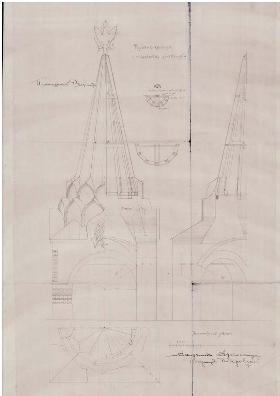
Илл. 16. Чертеж крыльца с показанием конструкции. Архитектор В.А. Покровский Измененный вариант. Диагональный разрез. 1911 г. ЦГАНТД. Ф. 282. Оп. 1. Д. 124.
