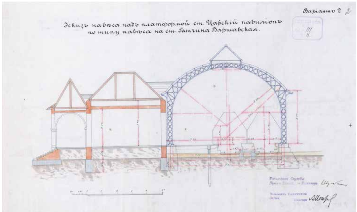
Илл. 19. Эскиз навеса над платформой ст. Царский павильон по типу навеса на ст. Гатчина Варшавская. Вариант 2. 1911 г. РГИА. Ф 350. Оп. 44. Д. 776. Л. 2.
