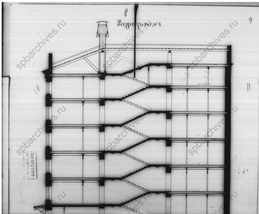
10. Разрез по №1. Чертежи дома В.Н.Крестина по Нюстадтской ул.,11 и Новой ул.,8 (Лесному пр., 13 и Новой ул.,8). ЦГИА СПб. Фонд 515. Опись 4. Дело 2419. Крайние даты документов: 15.09.1904;
