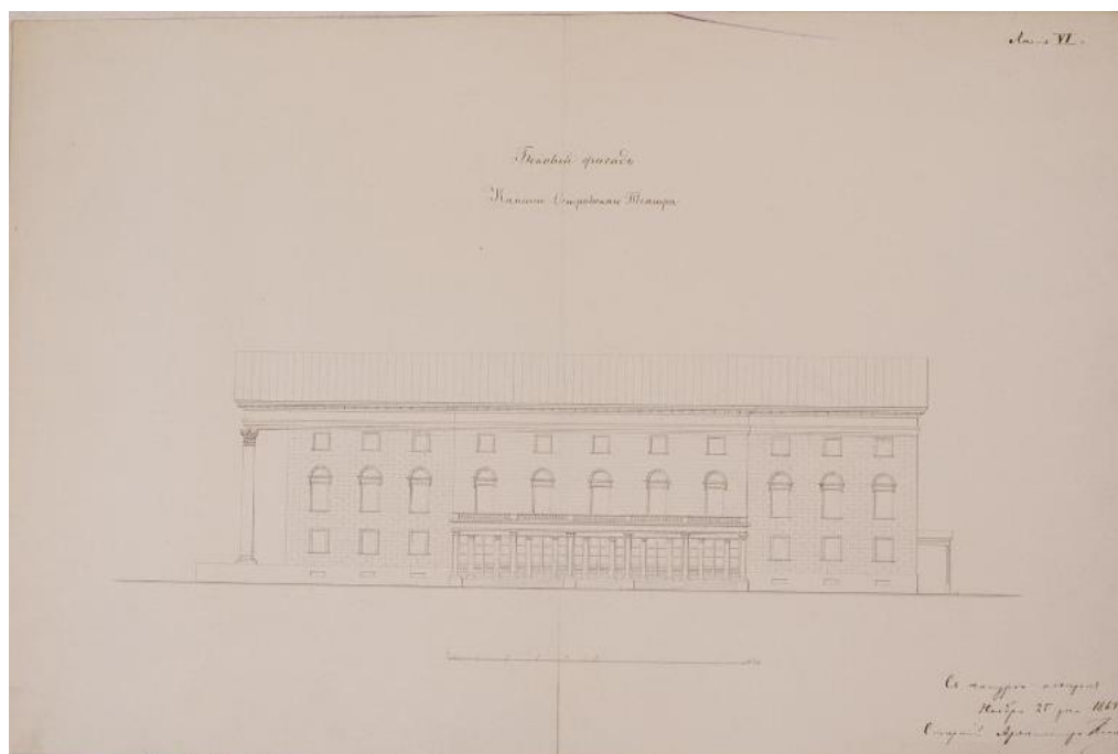
23. Арх. И.И. Климов. Обмер Каменноостровского театра в Санкт-Петербурге (бумага с водяными знаками («i.whatman 1864»), тушь). 1864 г. НИМ РАХ КП-49/26.
