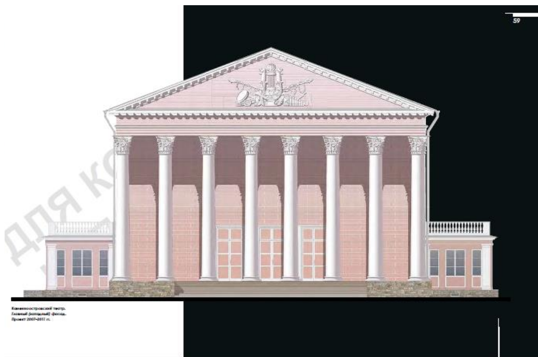
57. Камменноостровский театр. Главный (западный) фасад. Проект реставрации приспособления для современного использования. 2007-2011 гг. Опубликовано в: Дементьева В.А., Рахманов В.С., Шашкин А.Г., Бурыгин В.А. Камменноостровский театр. Синтез достижений реставрации и геотехники». (авторы:). СПб., 2014.
