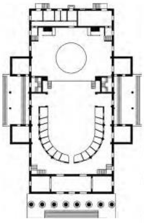
45. Каменноостровский театр. План первого этажа. Проект архитектора Е.И. Катонина. Период 1932-1964 гг. Опубликовано в: Дементьева В.А., Рахманов В.С., Шашкин А.Г., Бурьгин В.А. Каменноостровский театр. Синтез достижений реставрации и геотехники». (авторы:). СПб., 2014.
