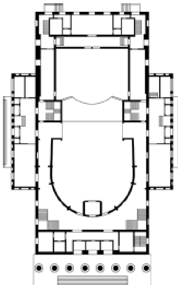
53. Каменноостровский театр. План первого этажа. Проект архитектора И.Н. Бенуа Период 1964-2007 гг. Опубликовано в: Дементьева В.А., Рахманов В.С., Шашкин А.Г., Бурьгин В.А. Каменноостровский театр. Синтез достижений реставрации и геотехники». (авторы:). СПб., 2014.
