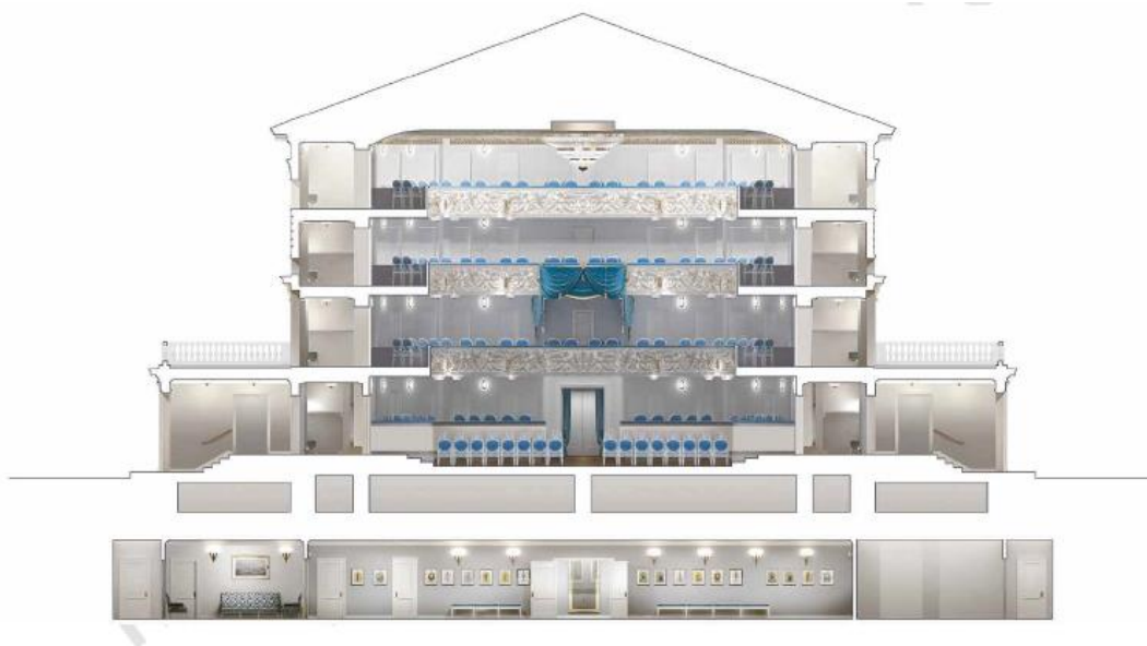
69. Каменноостровский театр. Проект реставрации приспособления для современного использования. 2007-2011 гг. Поперечный разрез по зрительному залу. Опубликовано в: Дементьева В.А., Рахманов В.С., Шашкин А.Г., Бурыгин В.А. Каменноостровский театр. Синтез достижений реставрации и геотехники». (авторы:). СПб., 2014.
