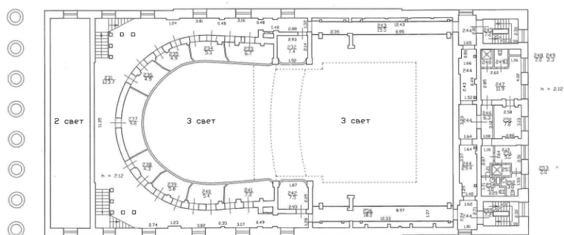
План 3 этажа
