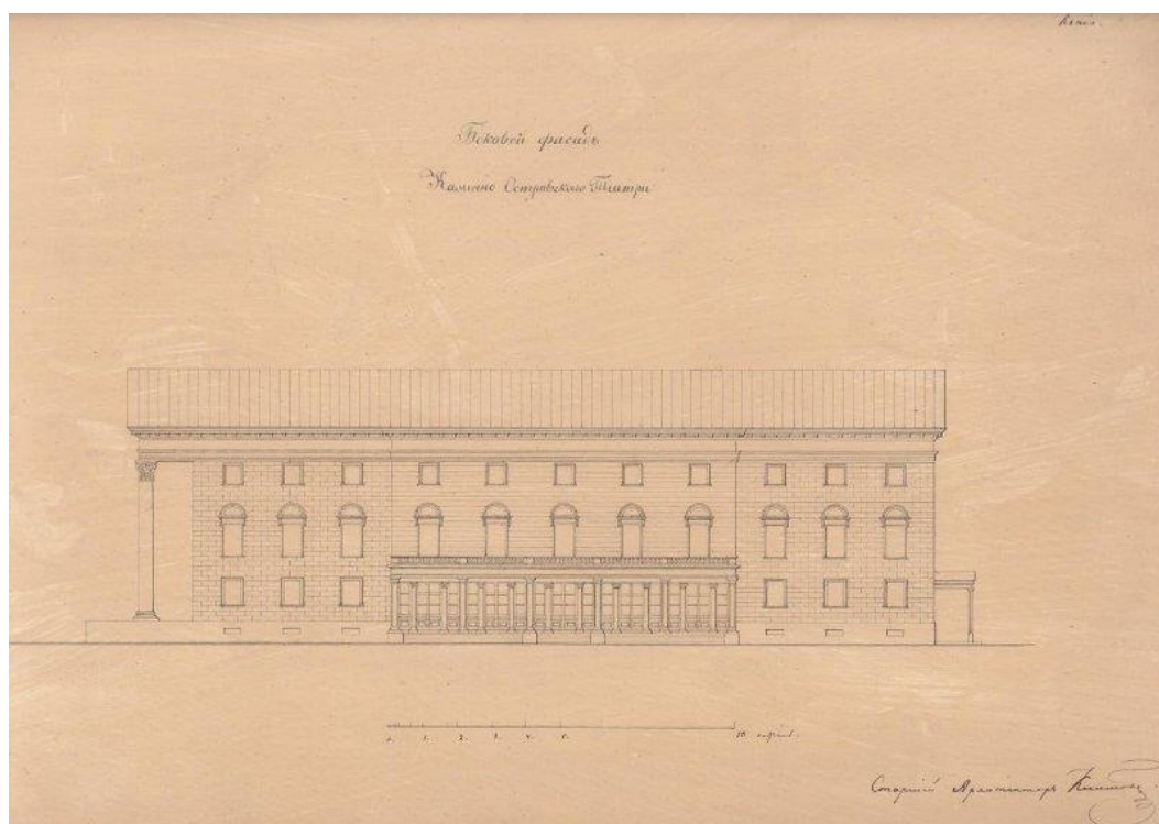
32. Арх. И.И. Климов Иван Иванович. Архитектурный рисунок. Боковой фасад Каменноостровского театра (бумага, акварель, тушь пером, лак). Последняя треть XIX в. СПбГМТМИ ГИК 3910/5.
