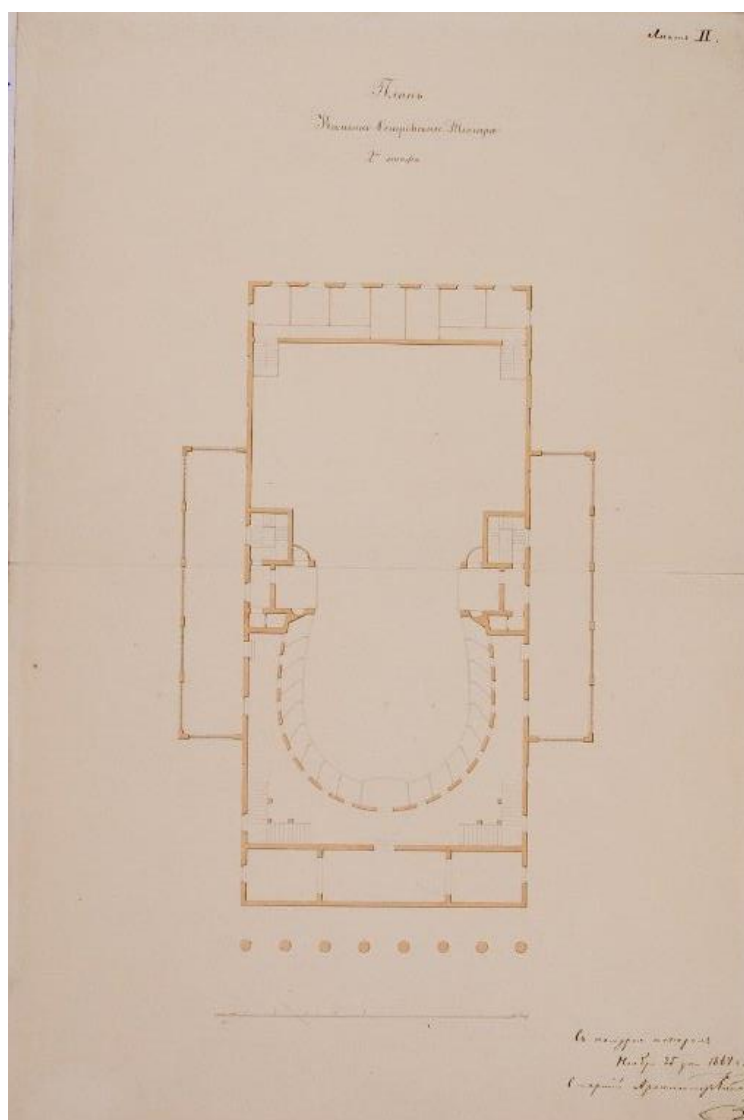
27. Арх. И.И. Климов. Обмер Каменноостровского театра в Санкт-Петербурге (бумага, тушь, заливка акварелью). 1864 г. НИМ РАХ КП-49/22.
