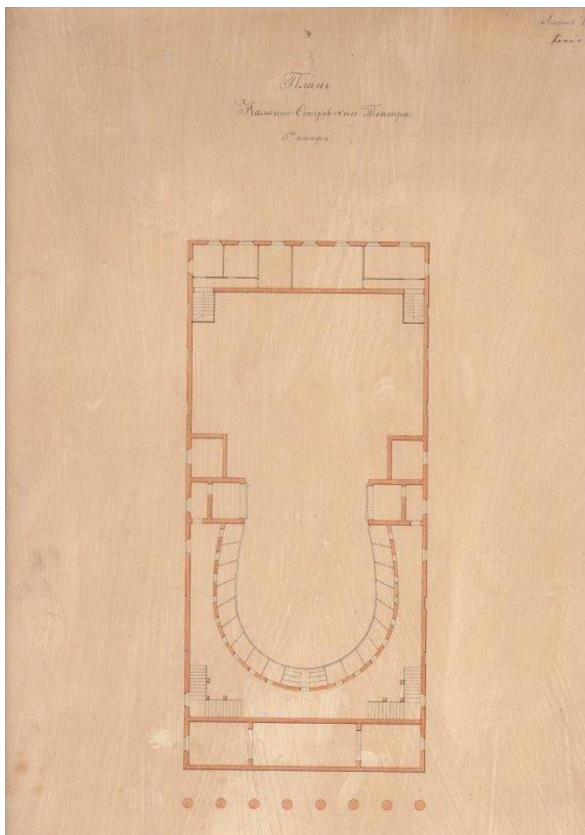
34. Арх. И.И. Климов. План Каменноостровского театра. Третий этаж (бумага, акварель, тушь пером, лак). Последняя треть XIX в. СПбГМТМИ ГИК 3910/2.
