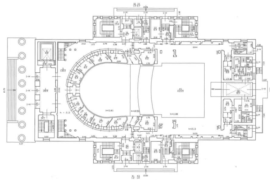
План 1 этажа
