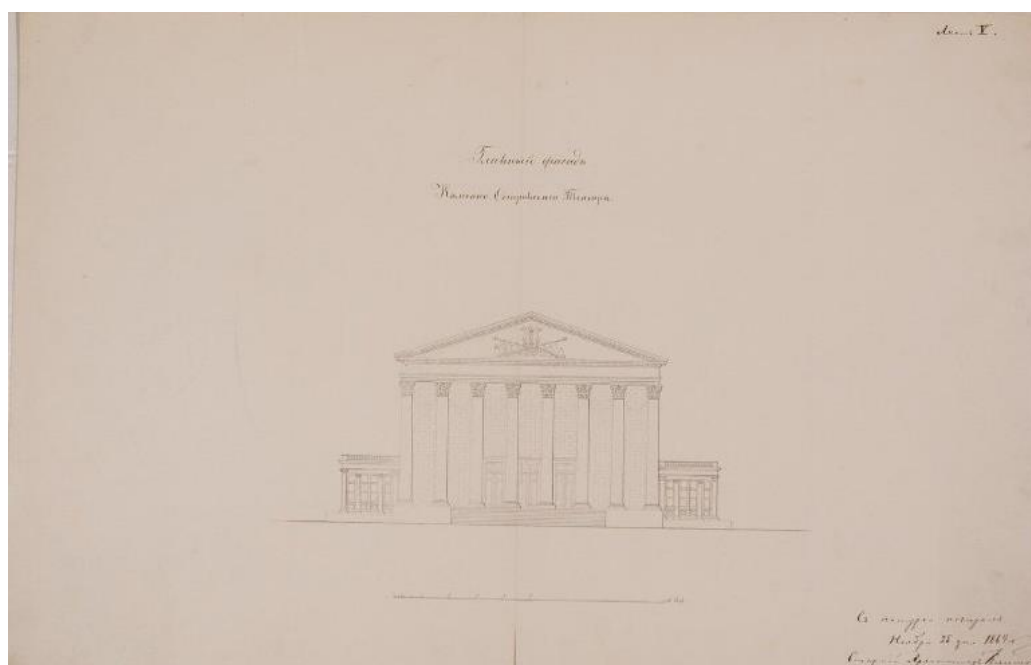
22. Арх. И.И. Климов. Обмер Каменноостровского театра в Санкт-Петербурге (бумага, тушь, заливка акварелью). 1864 г. НИМ РАХ КП-49/25.
