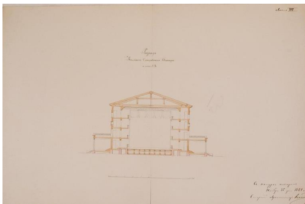
24. Арх. И.И. Климов. Обмер Каменноостровского театра в Санкт-Петербурге (бумага, тушь, заливка акварелью). 1864 г. НИМ РАХ КП-49/27.
