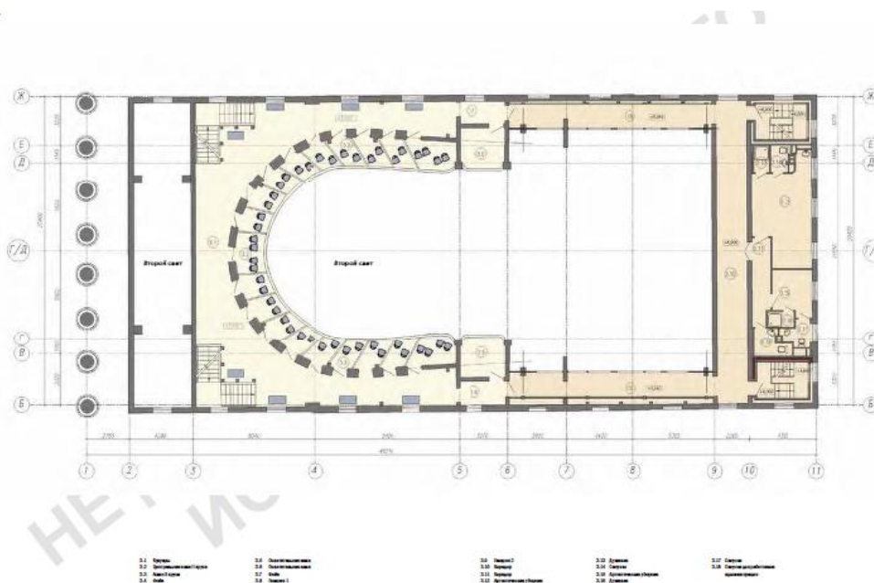
64. Каменноостровский театр. План третьего этажа. Проект реставрации приспособления для современного использования. 2007-2011 гг. Опубликовано в: Дементьева В.А., Рахманов В.С., Шашкин А.Г., Бурьгин В.А. Каменноостровский театр. Синтез достижений реставрации и геотехники». (авторы:). СПб., 2014.
