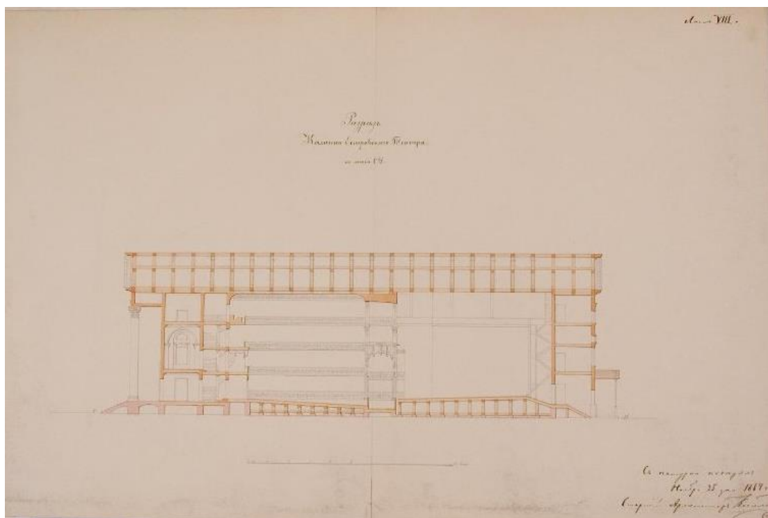
25. Арх. И.И. Климов. Обмер Каменноостровского театра Санкт-Петербурга (бумага, тушь, заливка акварелью). 1864 г. НИМ РАХ КП-49/28.
