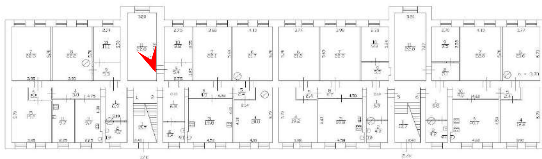
План 1 этажа
