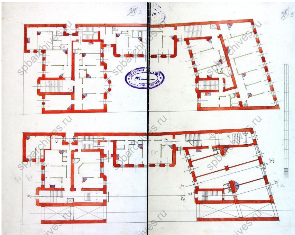
Илл. 10. ЦГИА СПб. Ф 513. Оп 102. Д. 3589. Чертежи дома на участке, принадлежавшем С.С. Трайнину по наб. Екатерининского кан., 158. 1911 г. Л. 2-5.
