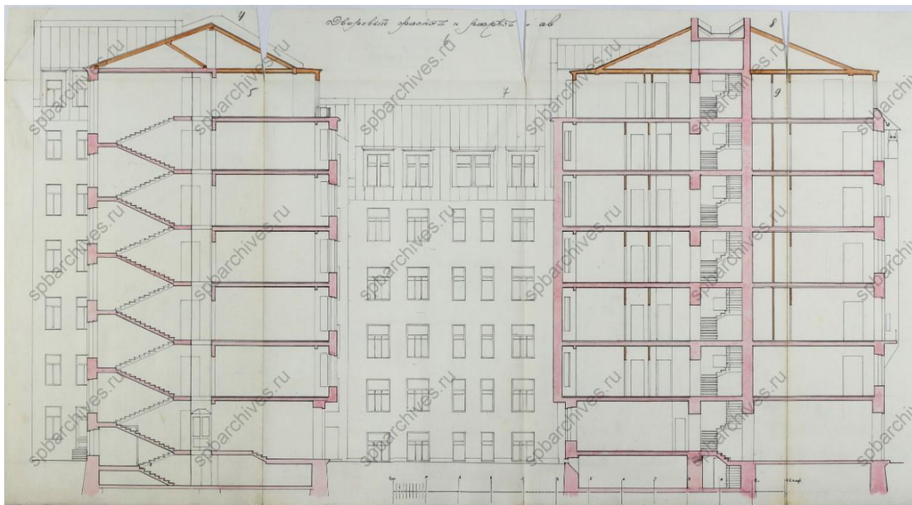
Илл. 13. ЦГИА СПб. Ф 515. Оп 4. Д. 914. План двора Соломона Самуиловича Трайнина Коломенской части 2-го участка по по наб. Екатерининского кан., 158. Разрез. 1912 г. Л. 4-8.
