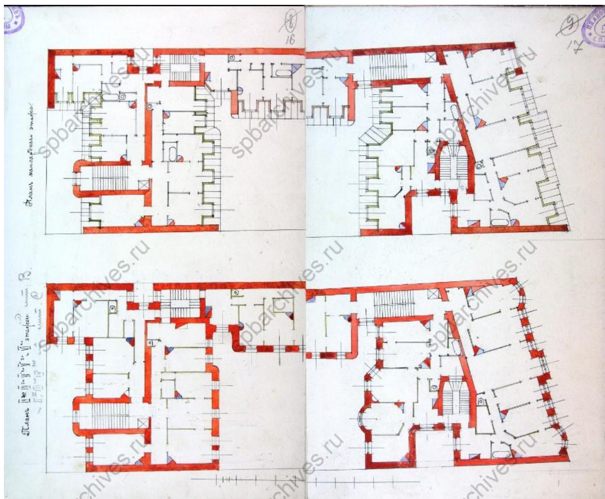
Илл. 12. ЦГИА СПб. Ф 513. Оп 102. Д. 3589. Чертежи дома на участке, принадлежавшем С.С. Трайнину по наб. Екатерининского кан., 158. 1911 г. Л. 16-17.
