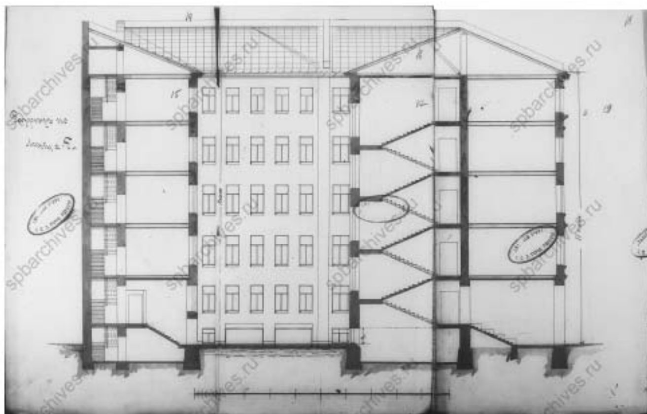
10. Разрез по линии аб. 1908 г. // Источник: ЦГИА СПб Ф.513 Оп.102 Д.9551 Л.14-19.
