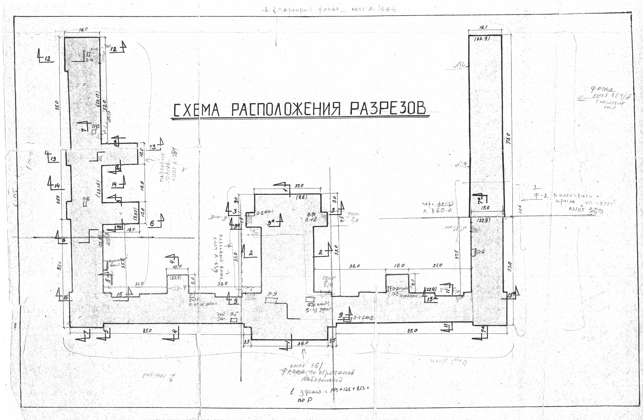
Илл. 7 Главное здание Военно-морской академии. Схема расположения разрезов. 1938. Арх. А.И. Васильев, А.П. Романовский. Архив Военно-морской академии.
