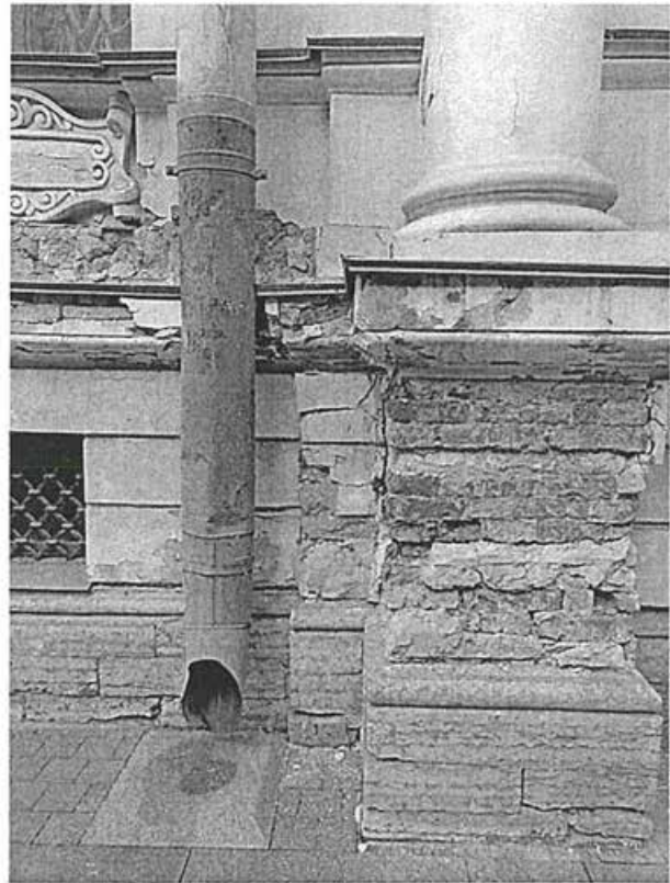
2. Вид на северный фасад объекта культурного наследия, биопоражения из-за деформации элемента водосточной трубы
