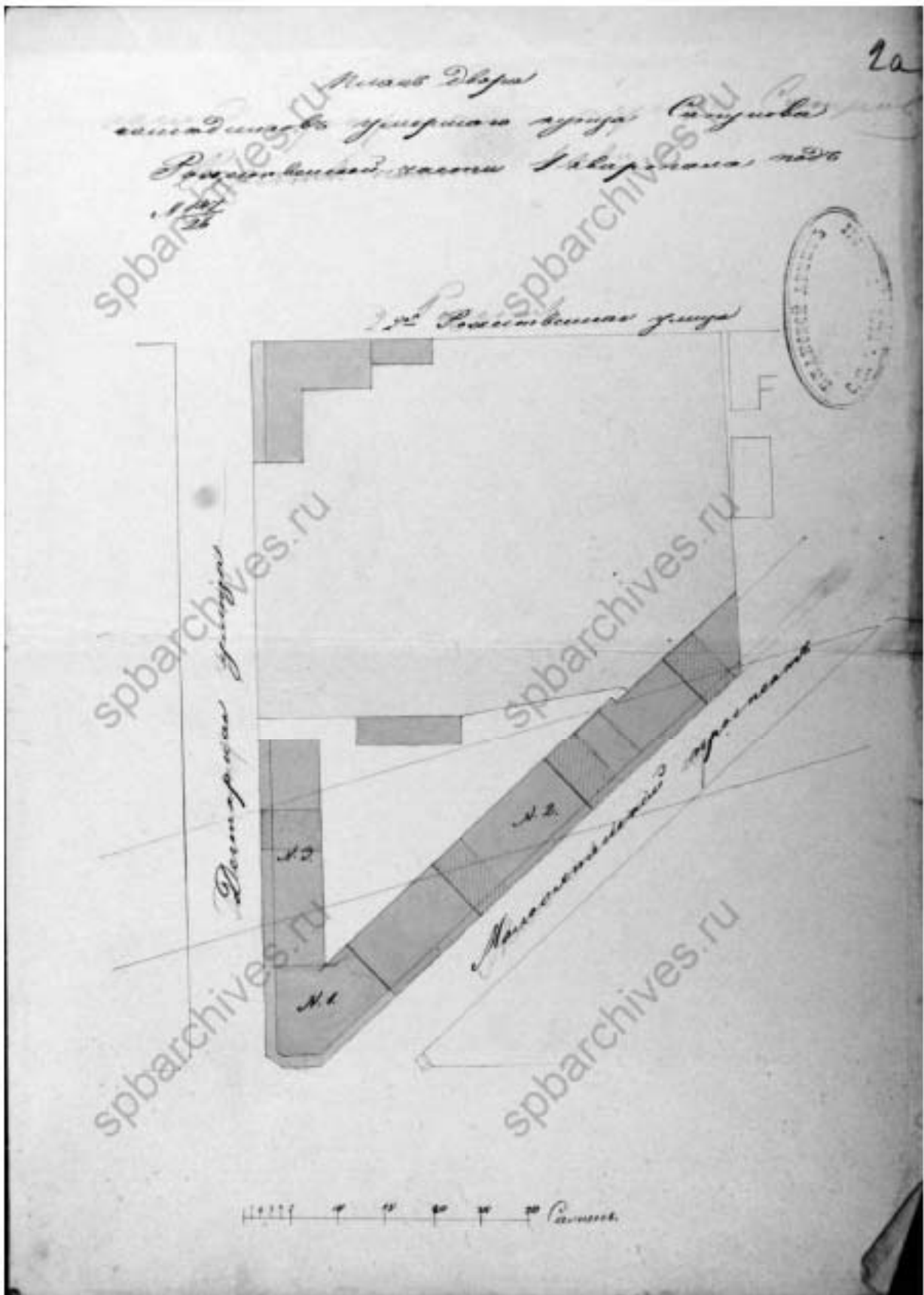
6. План двора наследников умершего купца Сапунова Рождественской части 1 квартала под №147/26. 1848 г. // Источник: ЦГИА СПб. Ф.513 Оп.102 Д.9154
