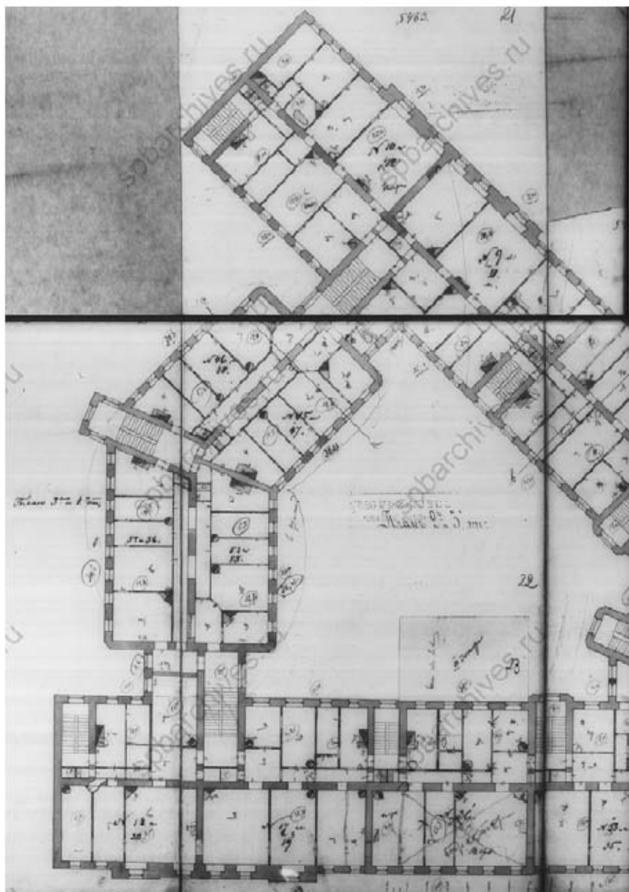
35. Фрагмент 2 и 3 этажей с перепланировкой. // Источник: ЦГИА СПб Ф.515 Оп.4 Д.84
