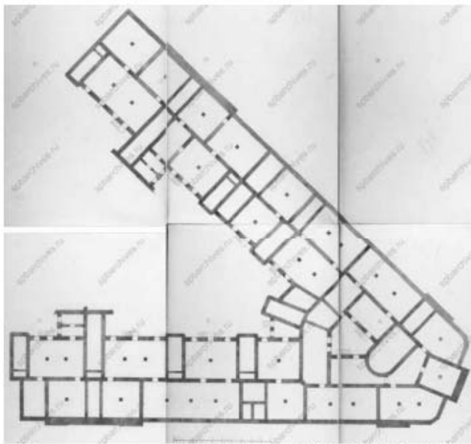
23. Без підписи (план підвала). 1880 г. // Источник: ЦГИА СПб Ф.513 Оп.102 Д.9154
