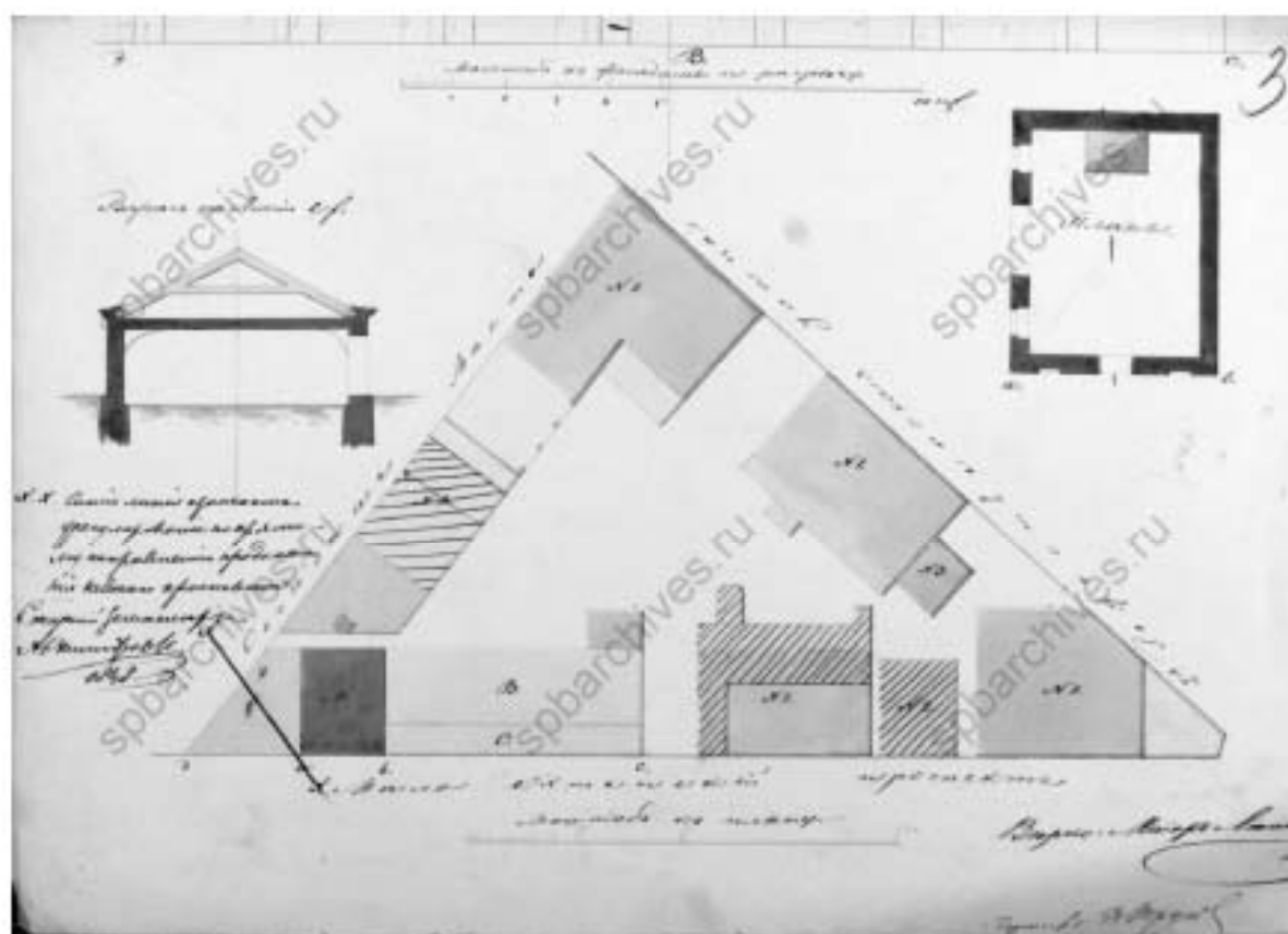
7. План двора С-Петербургского кушца Елисея Синтюрина состоящего Рождественской части 1-го квартала под №33/2 по Малому Охтенскому проспекту и 2 Рождественской улицы. 1848 г. // Источник: ЦГИА СПб ф 513 Оп.102 Д. 9154 Л.3.
